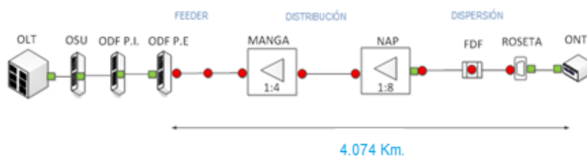
Figura 4.26: Modelo de Red GPON para la Ciudadela La Atarazana. [2]
