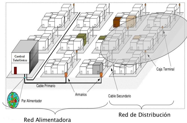
Figura 2.1: Elementos de Planta Externa. [5]
