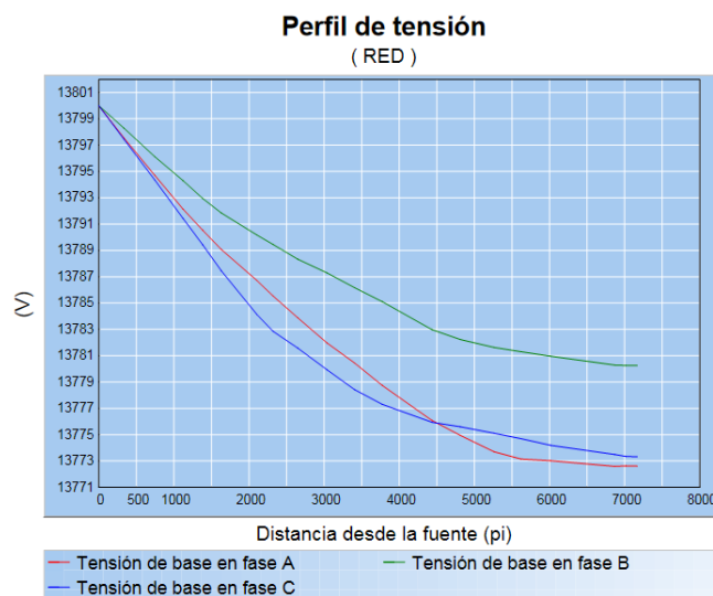
Figura 3.12. Perfil de Tensión a demanda máxima.
