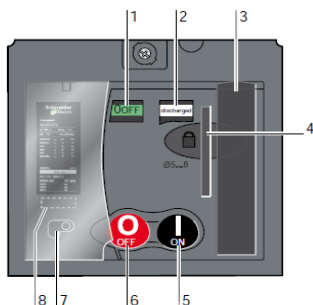
Compact NSX250 con mando motorizado.
