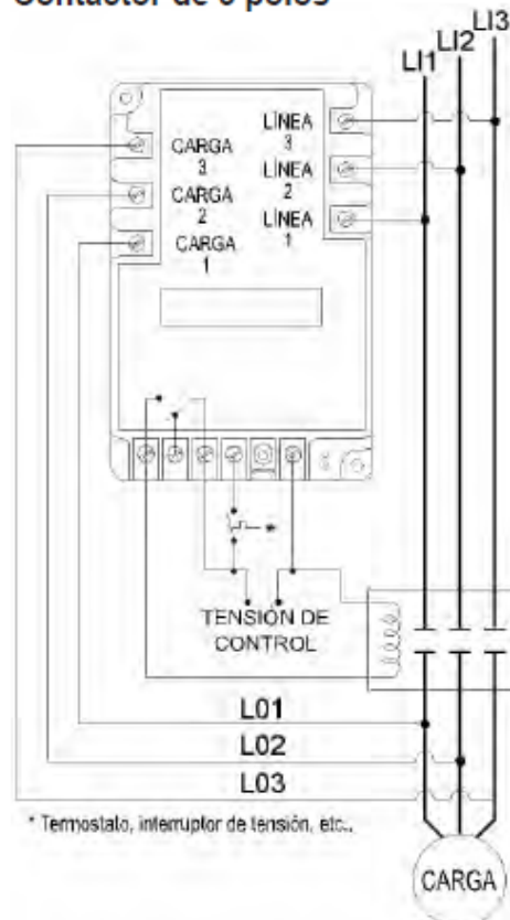
Contactor de 3 polos
