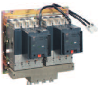
Interenclavamiento por placa soporte de dos interruptores automáticos Compact NS telemandados.
