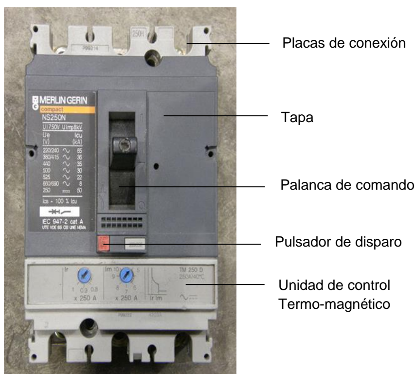
Figura 1.6: Partes del Interruptor automático Compact.
