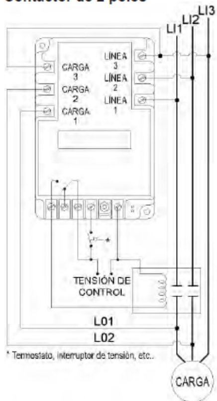
Contactor de 2 polos
