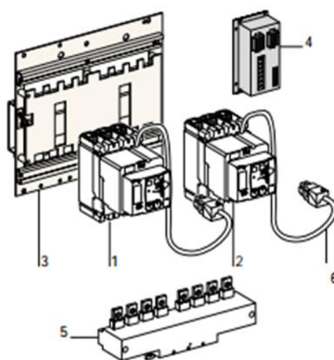
Figura 1.3: Elementos de la Transferencia de redes sin automatismo.
