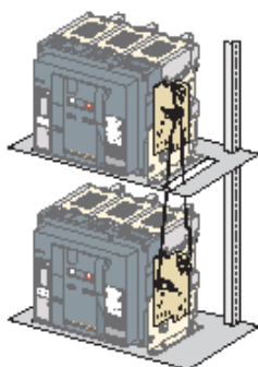
Interenclavamiento por varillas de 2 aparatos Masterpact NT y NW.
