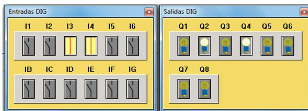
Figura 2.8: Modo manual y generador: Presencia de generador.
