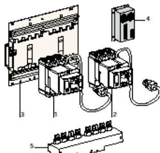
Sistema de inversión de redes motorizado.
