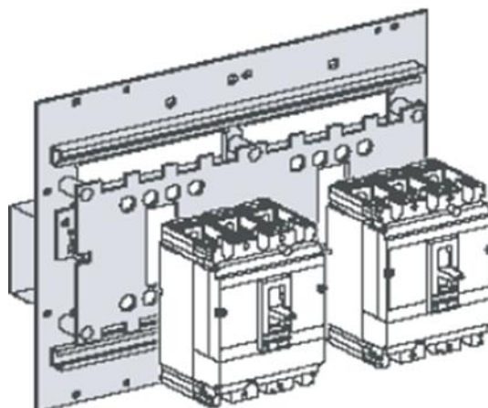
Figura 1.8: Enclavamiento mecánico por platina.
