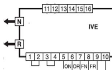
Figura 2.11: Terminales del bloque IVE.
