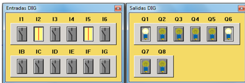
Figura 2.6: Apagado de generador y presencia de red.
