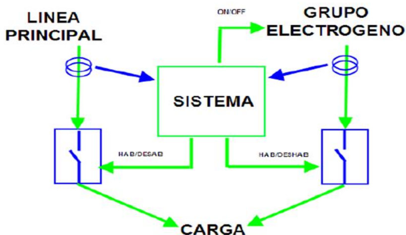
Figura 1.1: Sistema de transferencia entre dos fuentes.
