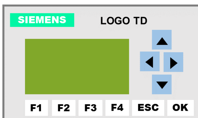
Figura 4.2. Pantalla de control LOGO TD.
