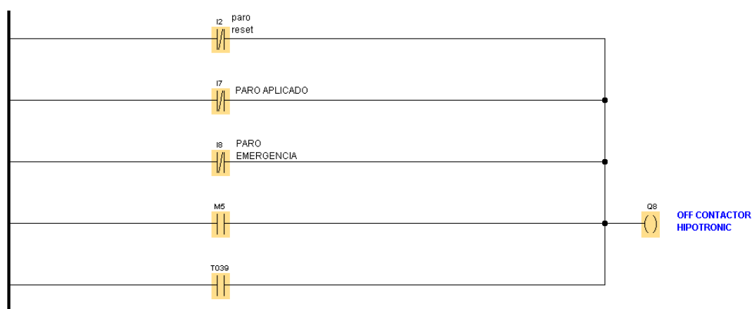
Figura 3.10. Activación de la máquina HIPOTRONIC a través del micro PLC LOGO.
