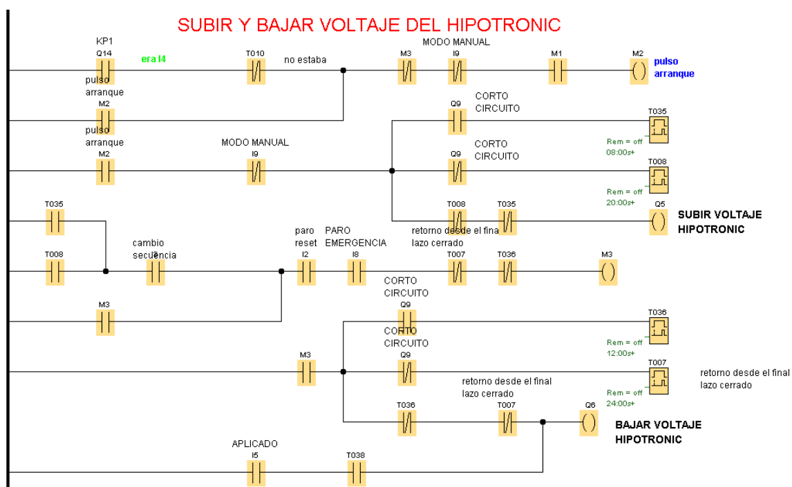
Figura 3.12. Control para subir y bajar voltaje del Hipotronic.
