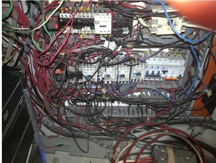
Figura 1.1. circuito de fuerza actual de pruebas de vacío y cortocircuito.
