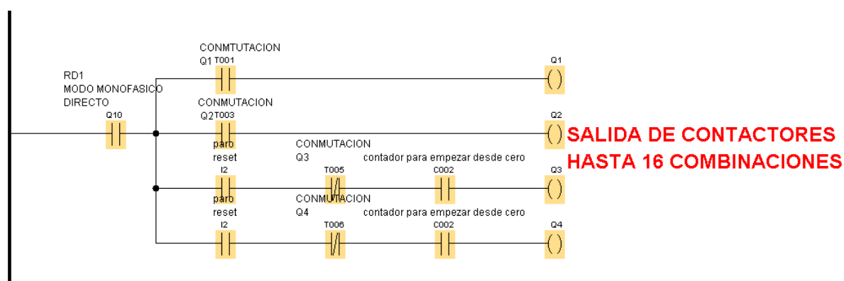
Figura 3.8. Combinación binaria de 4 salidas a 16 combinaciones.
