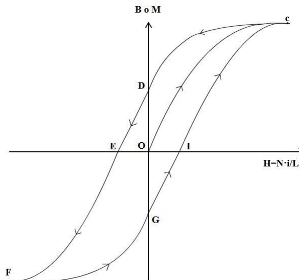
Figura 2.4. Ciclo de histéresis en un material ferromagnético. [7]
