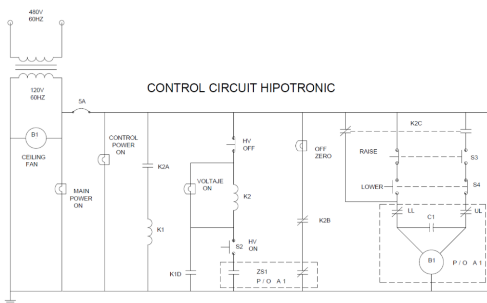
Figura 3.13. Circuito original del control máquina HIPOTRONIC.
