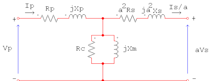
Figura 2.2. Circuito equivalente de un transformador. [3]
