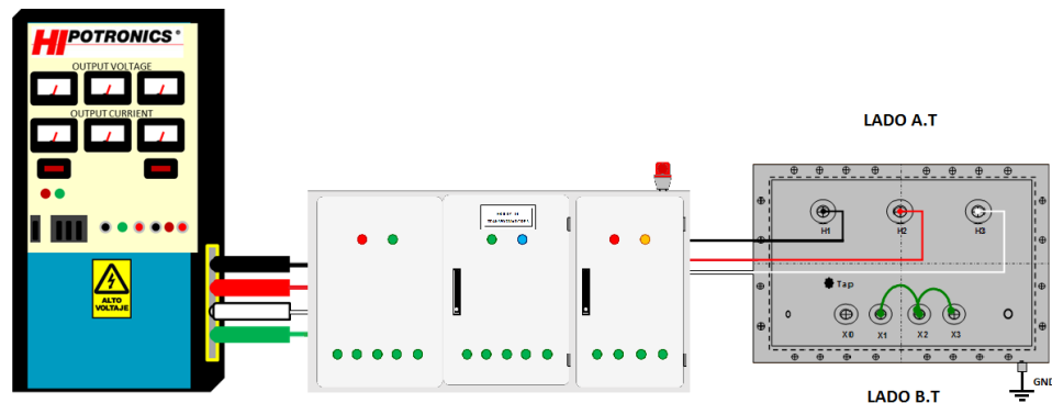
Figura 5.27. Prueba de cortocircuito de un transformador trifásico.
