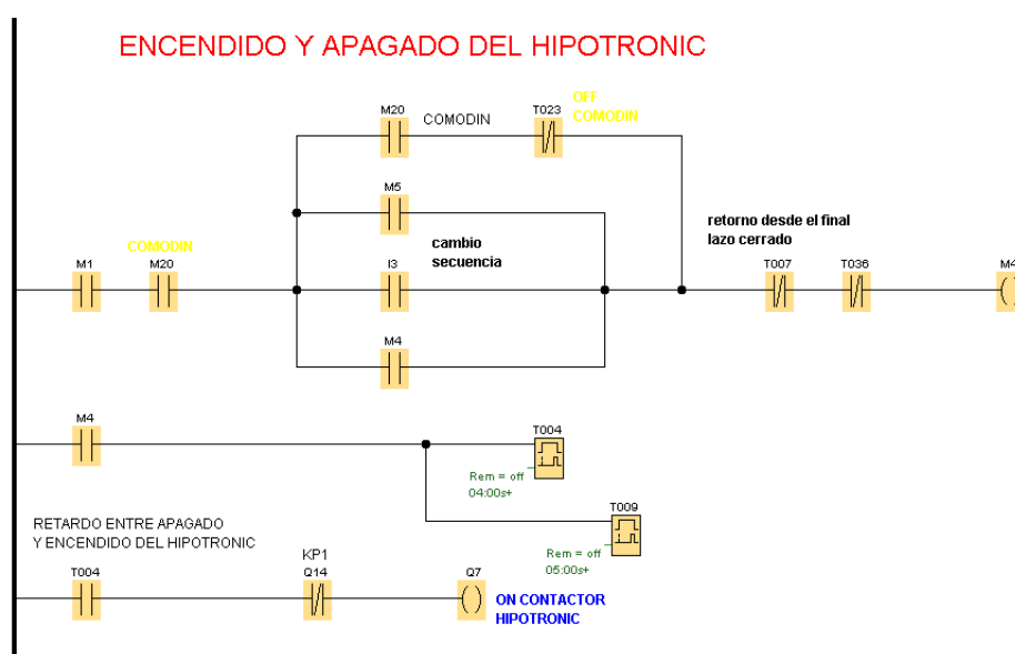
Figura 3.10. Activación de la máquina HIPOTRONIC a través del micro PLC LOGO.
