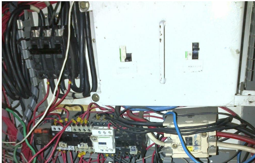
Figura 1.2. Transferencia de alimentación monofásica a manual.
