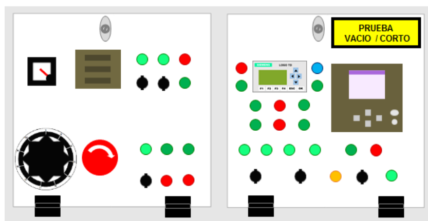
Figura 4.1. Diseño del nuevo panel de control.
