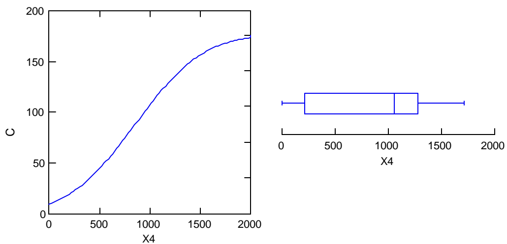
Figura 1.8 Ojva y Diagrama de Cajas de la variable X_4
