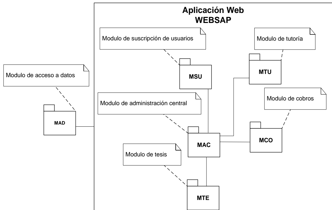
Figura 5.2 Módulos del Sistema.
