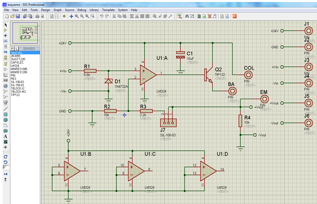
Figura 1: Diseño Amplificador
