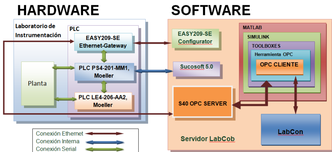
Figura 2.20: Arquitectura de control del proyecto de graduación
