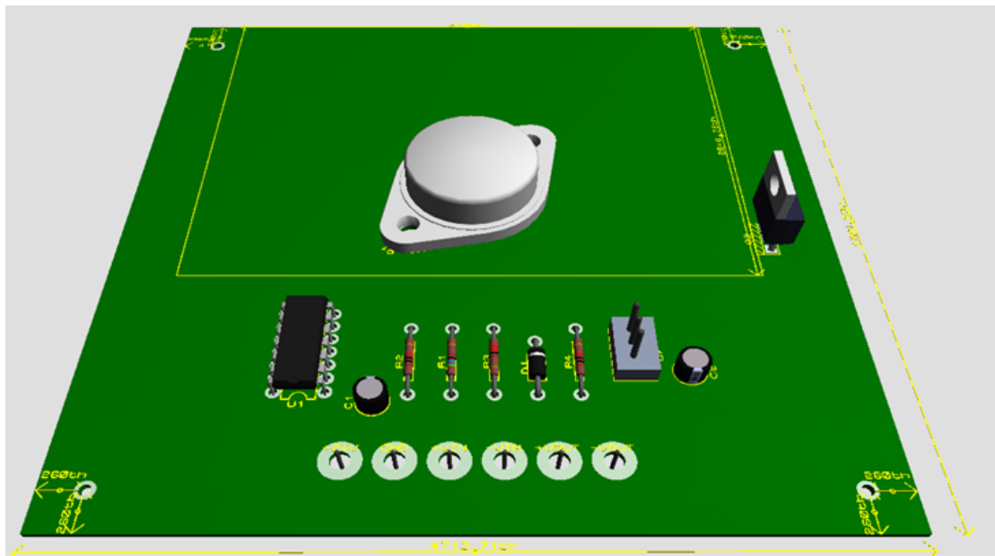
Figura 2: Vista de la amplificador terminado
