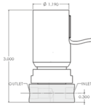
Figura 2.16: Válvula de control neumática IQ Mini
