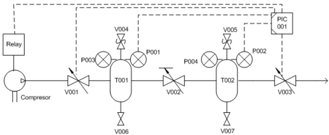
Figura 2.19: Diagrama P&ID de la planta de regulación de presión
