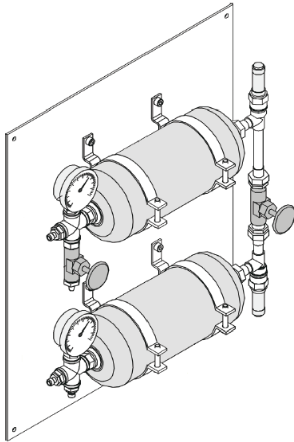
Figura 2.10: Tanques de Presión-Planta Gunt RT450.03
