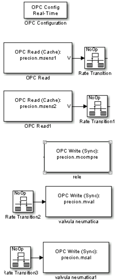
Figura 3.34: Bloque configurados de la planta de regulación de presión
