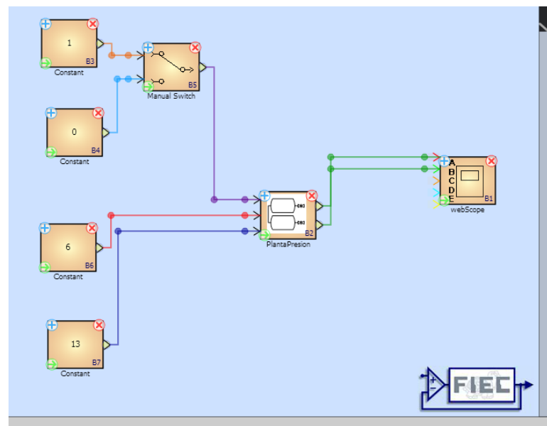
Figura 4.4: Diagrama de Bloques Práctica
