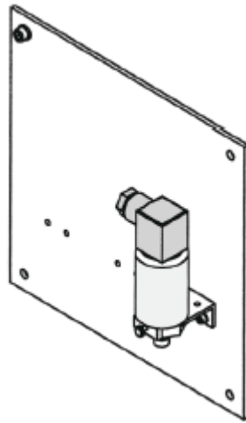
Figura 2.12: Sensor de Presión-Planta Gunt RT450.03
