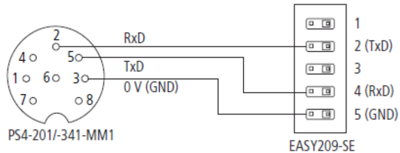
Figura 3.1: Configuración de cable de comunicación de la interfaz RS232
