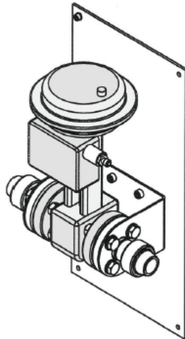
Figura 2.11: Válvula de control neumática-Planta Gunt RT450.03
