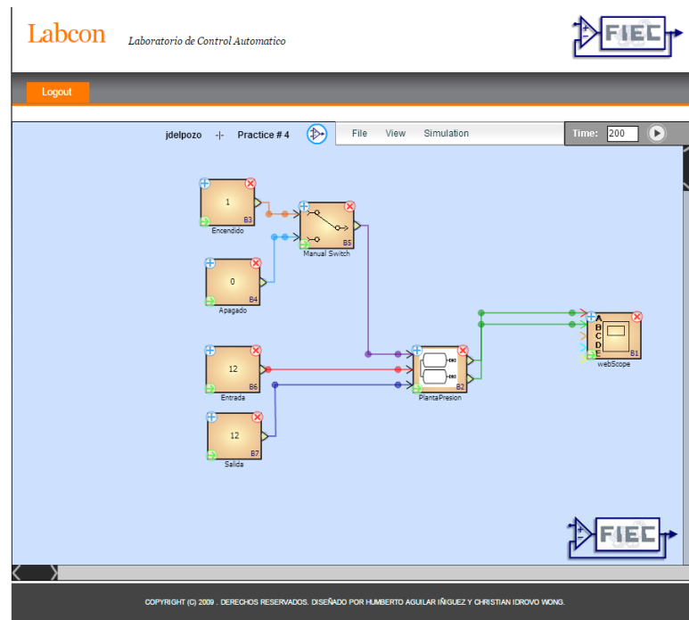
Figura 4.2: Diagrama de Bloques Prueba de comunicación
