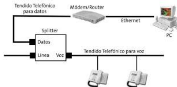
Figura 2.- Uso del Splitter del lado del usuario [3]
