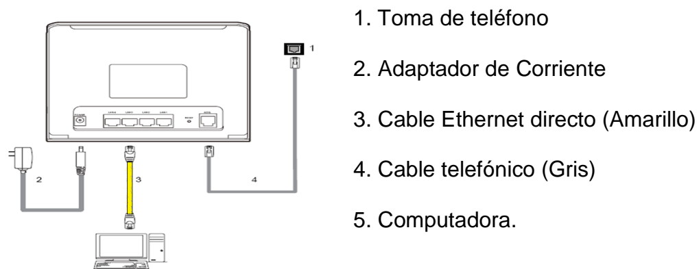
Figura 23.- Conexión Simple del Modem [28]
