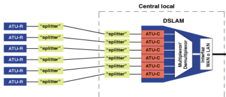
Figura 15.- Estructura de un armario DSLAM [20]
