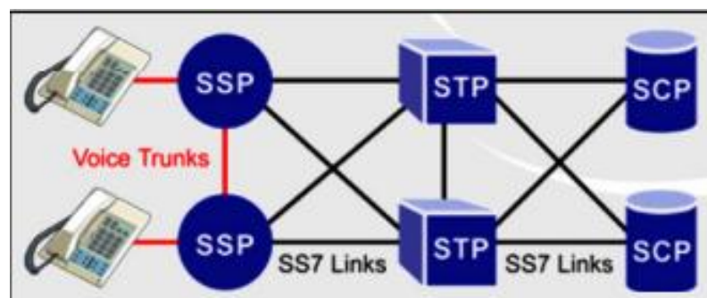
Figura 1.6: Arquitectura Básica de Señalización [6]
