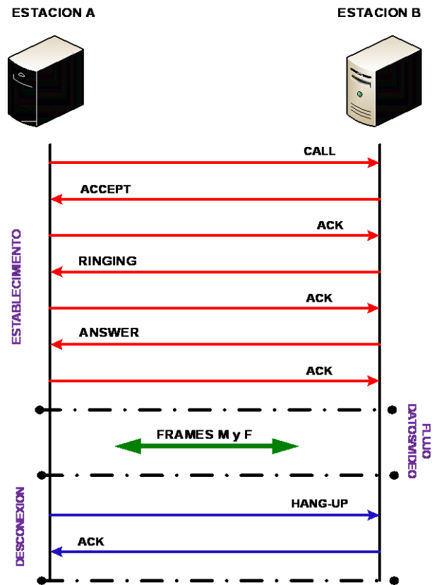
Figura 3.23: Proceso de una llamada IAX [10]
