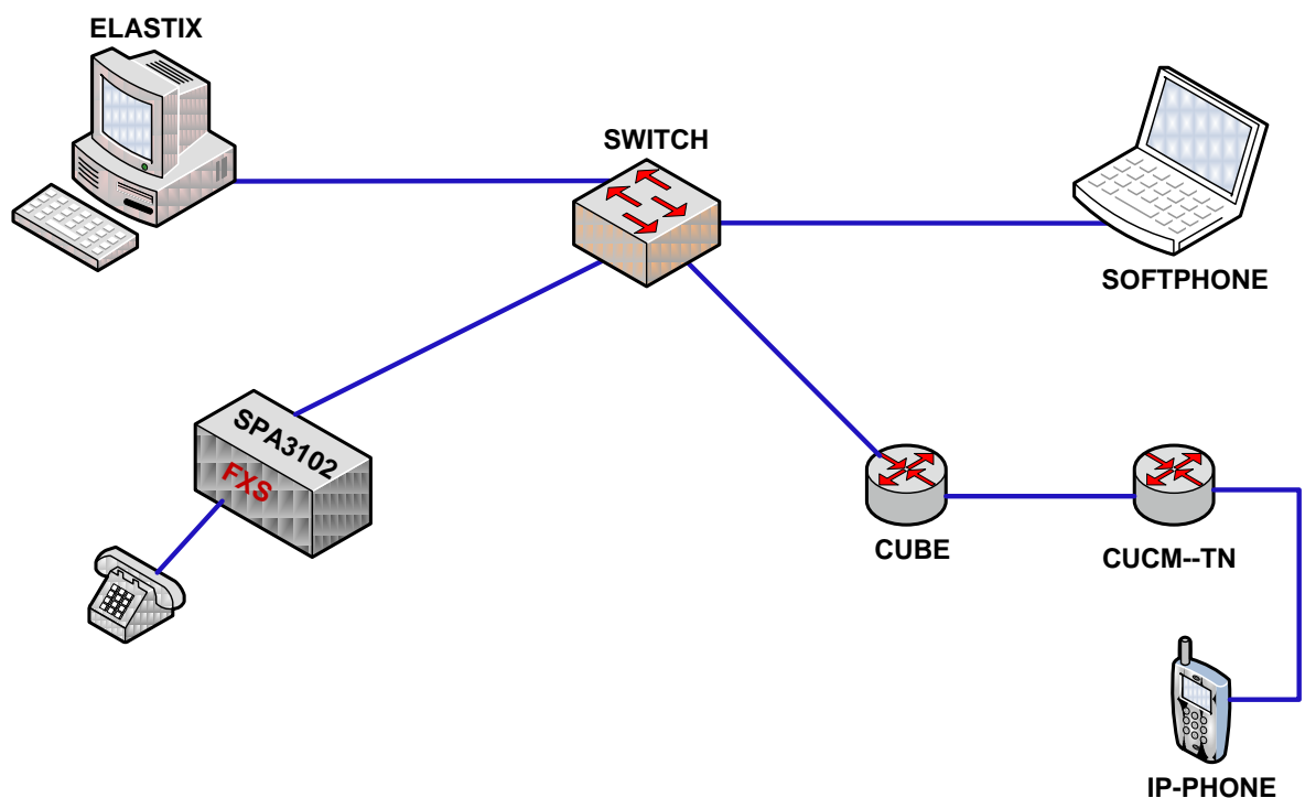
Figura 3.18: Diseño Red Cisco Conectada a una PSTN
