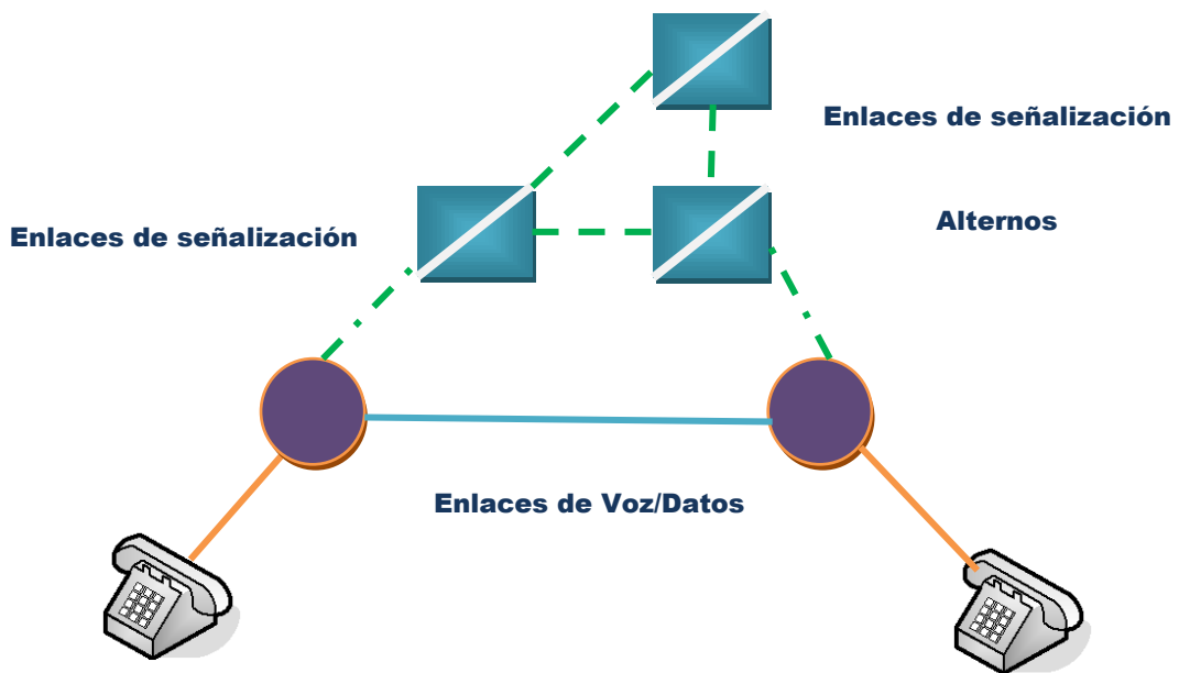
Figura 1.5: Modo Cuasi-Asociado de Señalización [8]
