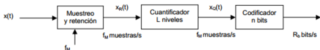
Figura 2.2: Modulación PCM [2]
