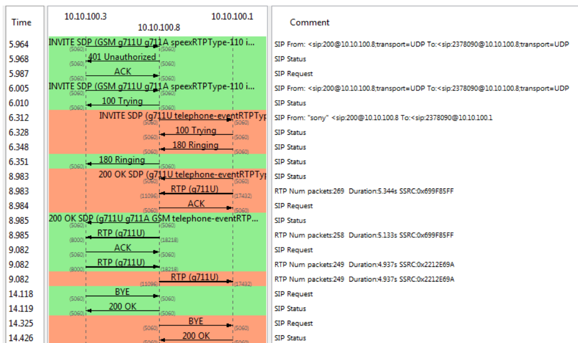
Figura 3.26: Flujo de una Llamada Exitosa-Extensiones 201-200.
