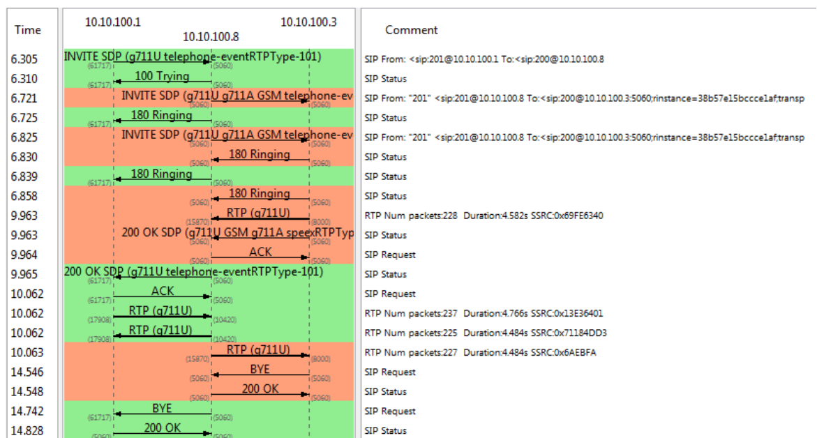
Figura 3.25: Flujo de una Llamada Exitosa-Extensiones 201-200.
