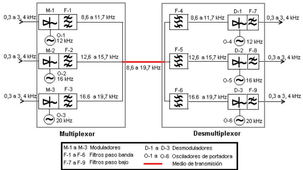
Figura 3.20: Multiplexor de Frecuencia [11]
