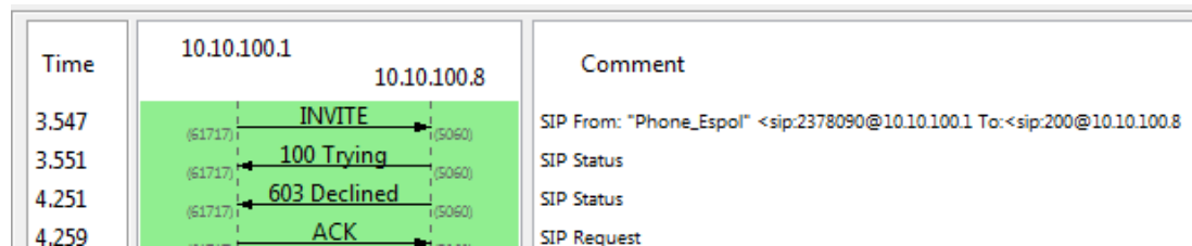
Figura 3.24: Término de una Llamada.
