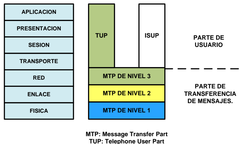
Figura 1.7: Protocolos de Señalización [3]
