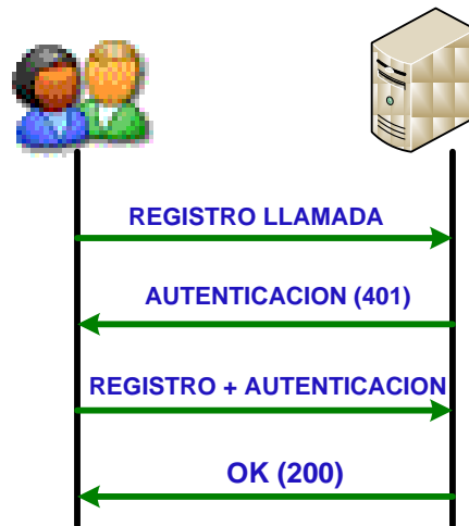
Figura 3.22: Proceso de una llamada SIP [10]
