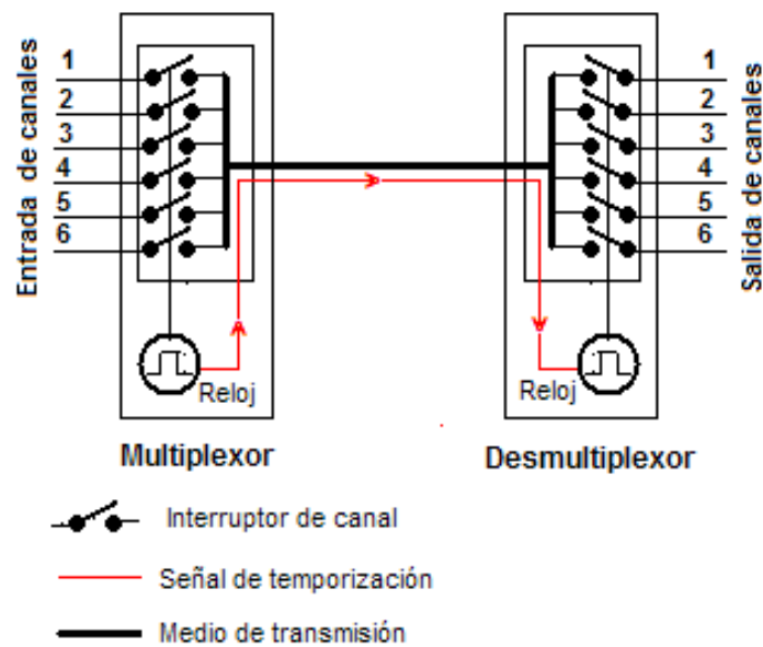
Figura 3.21: Multiplexor de Tiempo [12]
