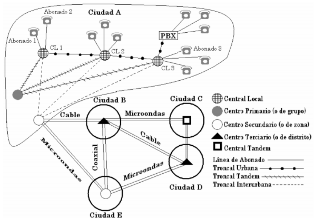
Figura 2.3: Estructura de la PSTN [2]
