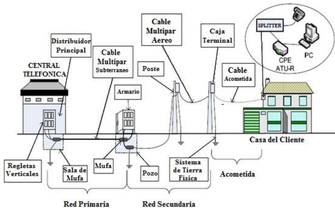
Fig. 2.11 Planta Externa. [23]
