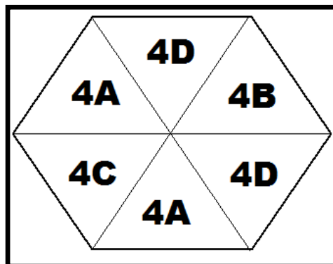
Figura 4.8 Orden de las frecuencias utilizando el plan de frecuencia 4
