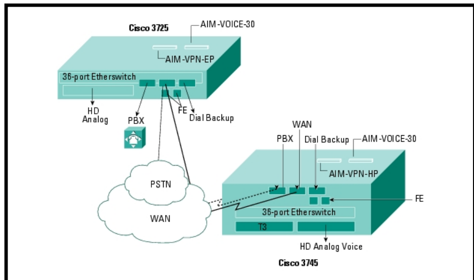
Figure 4.14. Escenarios de la Sucursal de Servicio Completo.
