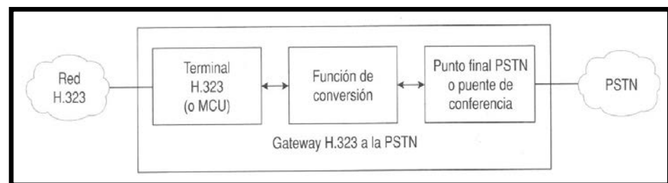
Figura 2.7. Estructura lógica de un gateway H.323.
