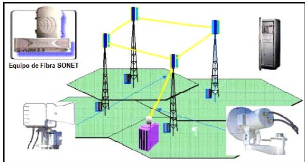
Figura 1.13. Topología de red LMDS con infraestructura de fibra
