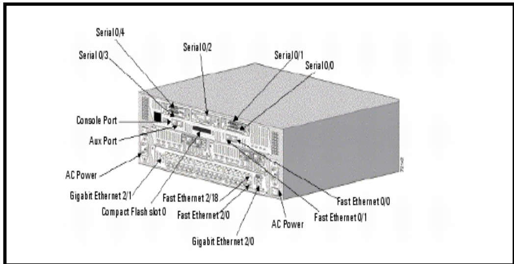
Figura 4.10. Router de acceso múltiple cisco 3745
