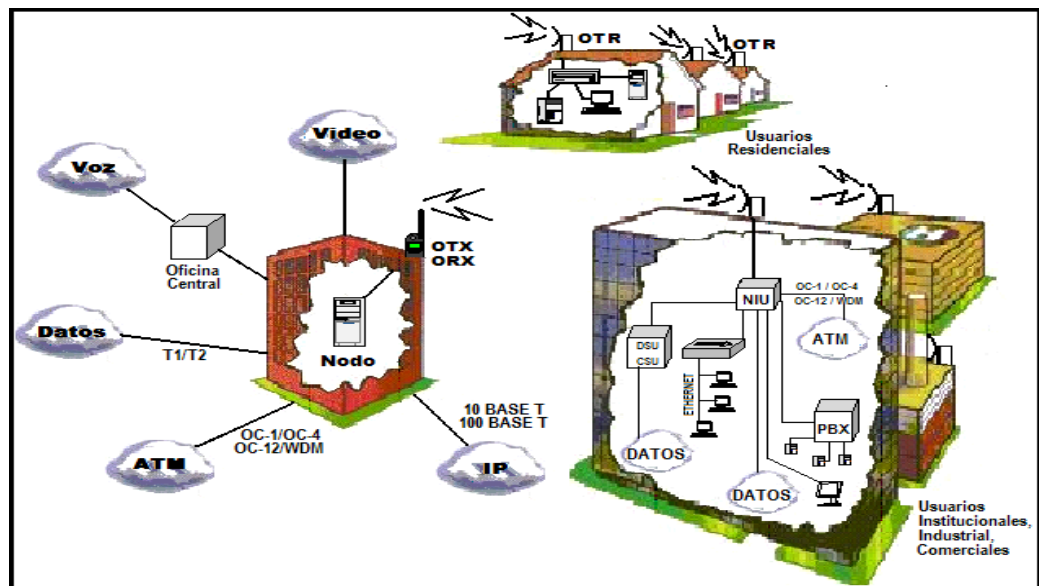
Figura 1.12. Representación de una red LMDS.
