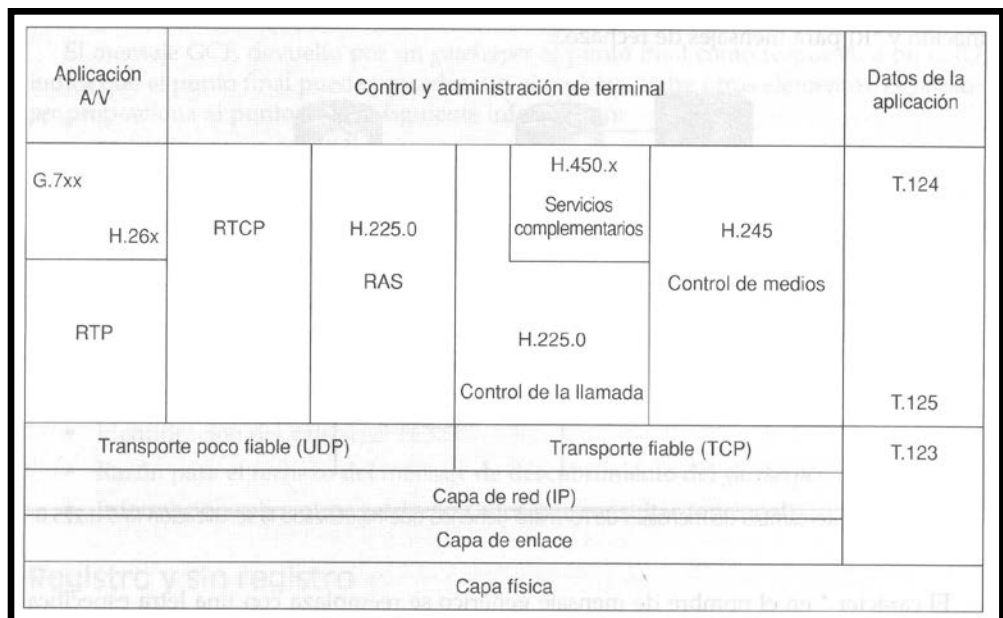
Figura 2.8. Pila del protocolo H.323.
