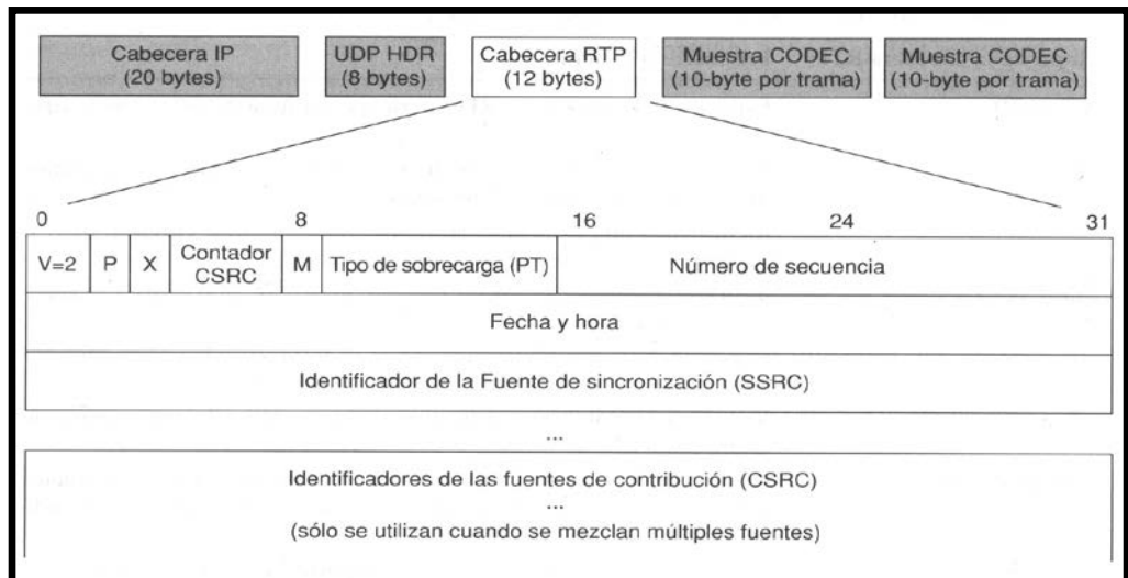
Figura 2.2. Paquete VoIP con cabecera RTP enfatizada.
