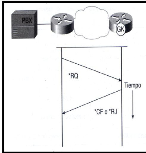
Figura 2.9 Intercambio de mensajes de formato genérico que ha utilizado la señalización H.225
