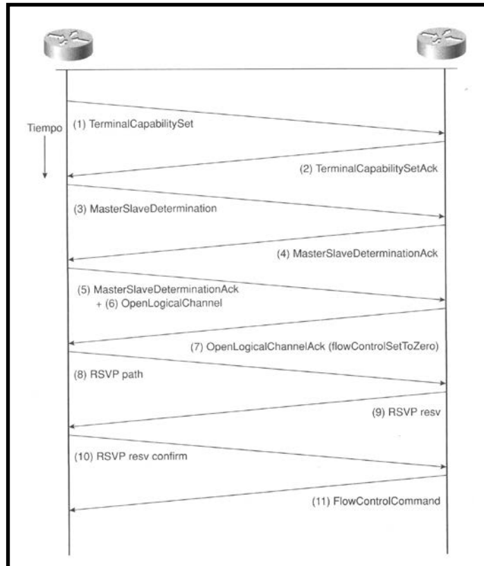
Figura 2.10. El flujo de medios se establece mediante los mensajes de control de medios H.245
