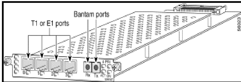
Figura 4.16: Tarjeta DFC de 4 puertos E1
