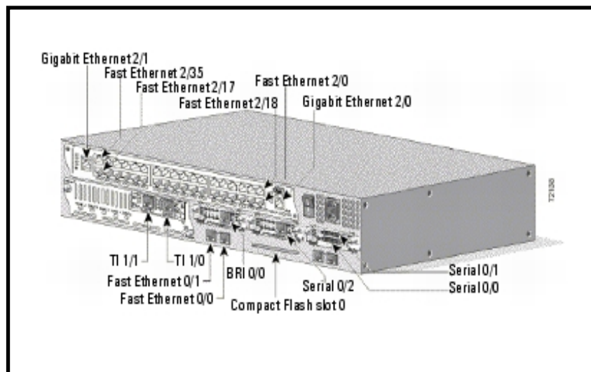
Figura 4.11. Router de acceso multiservicio cisco 3725
