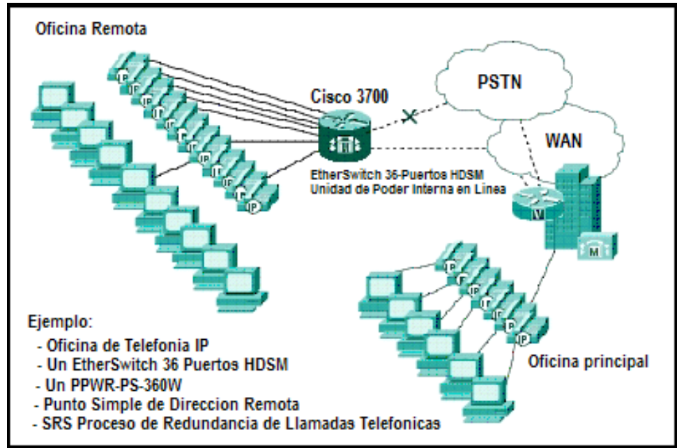
Figure 4.13. Capacidades integradas de una sucursal de servicio completo cisco serie 3700
