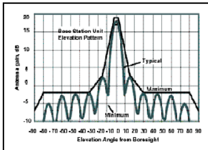
Figura 4.6. Elevación Antena de la Estación Base
