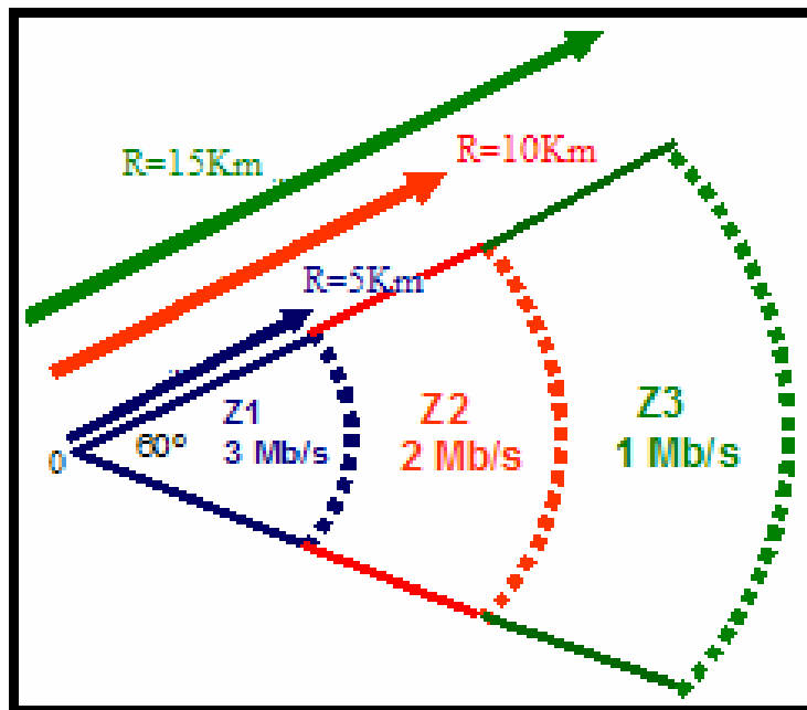
Figura 1.2. Representación de la velocidad de transmisión con respecto al radio de cobertura
