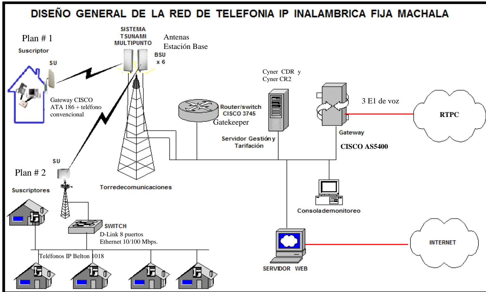
Figura 4.2. Diagrama general del diseño de la red telefonía IP.
