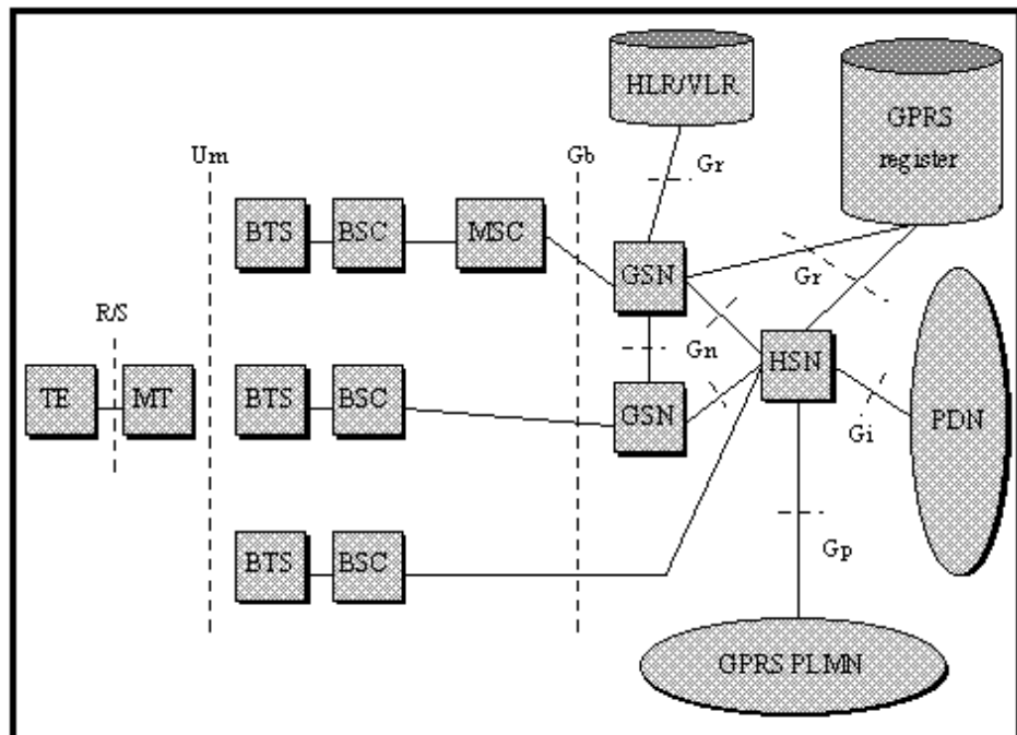
Figura. 1.5. Modelo de red GPRS
