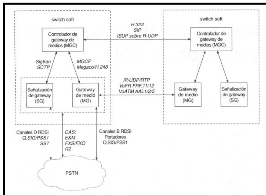
Figura 2.1. Arquitectura de RTPC integrada y telefonía en Internet.
