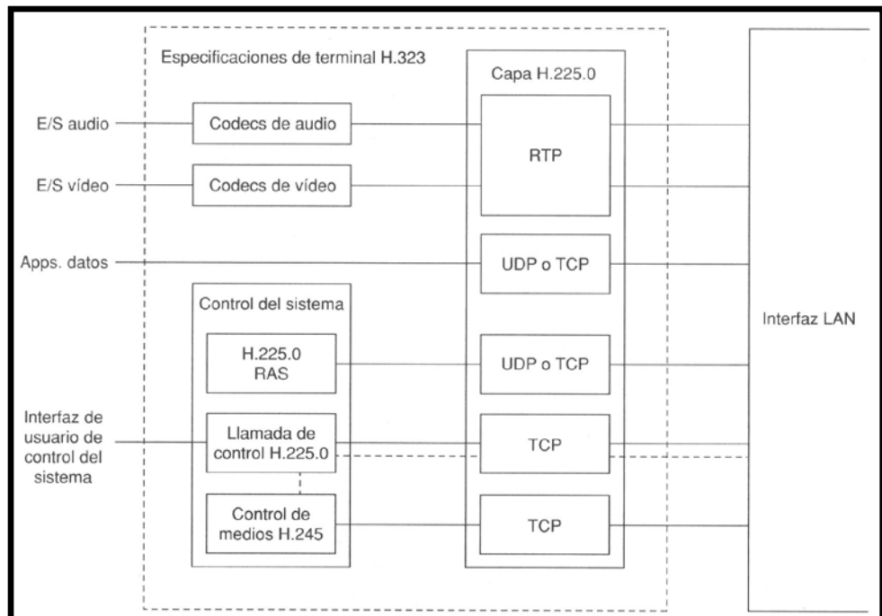
Figura 2.5. Elementos funcionales de un terminal H.323
