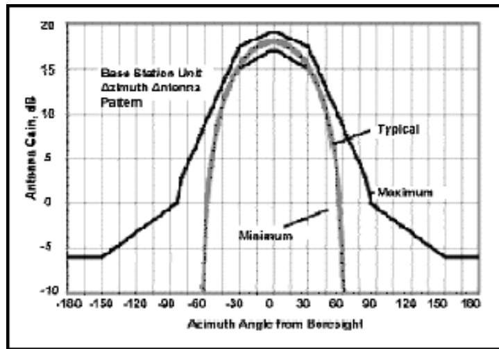
Figura 4.5. Azimuth Antena de la Estación Base
