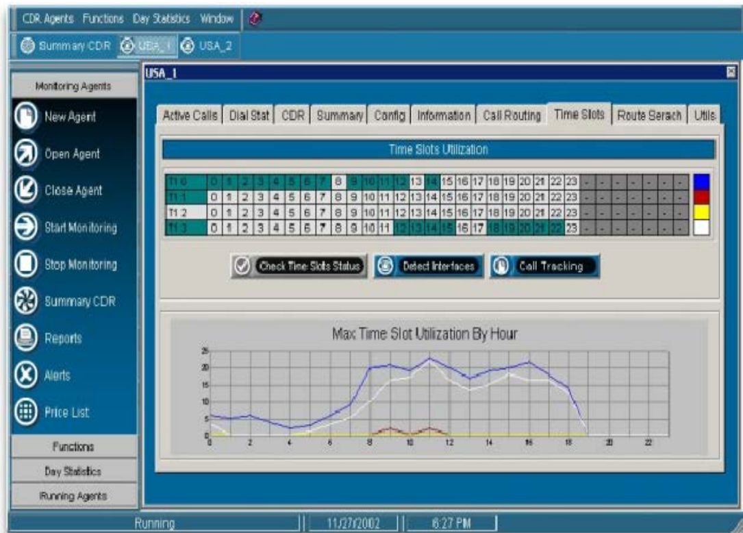
Figura 6.7. Ranuras de tiempo utilizadas a intervalos de una hora
