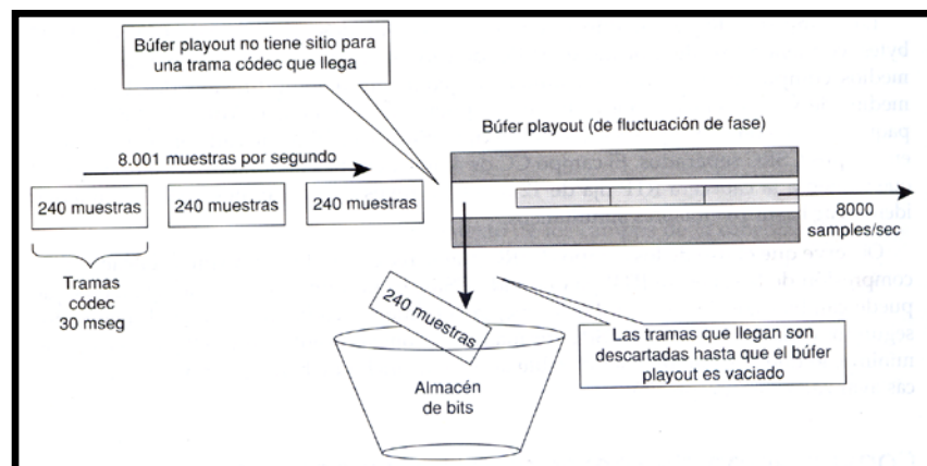
Figura 2.3. Diferencia entre los relojes de muestreo de envío y recepción afectan a los buffer playout.
