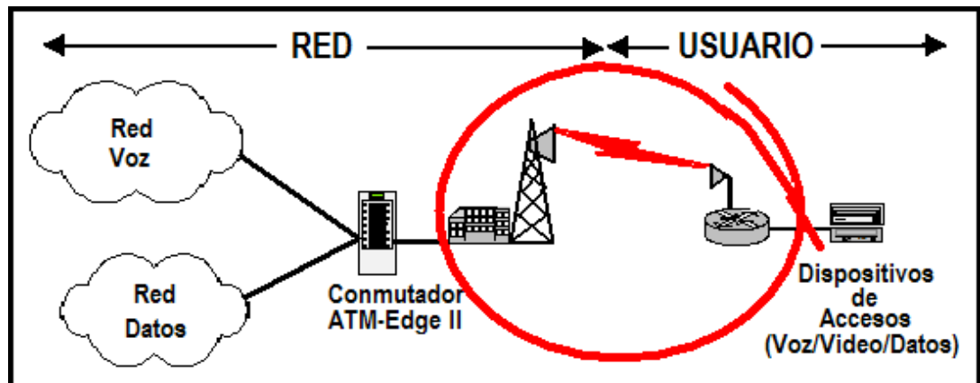
Figura 1.14. Topología de red LMDS entre el suscriptor y la red de servicios.
