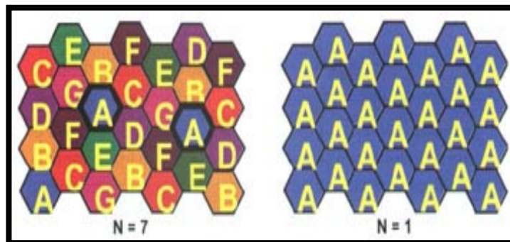
Figura 1.11. En los sistemas AMPS, FDMA y TDMA el espectro debe ser segmentado en 7 partes para evitar interferencias entre celdas adyacentes. En cambio la planificación de CDMA se simplifica
