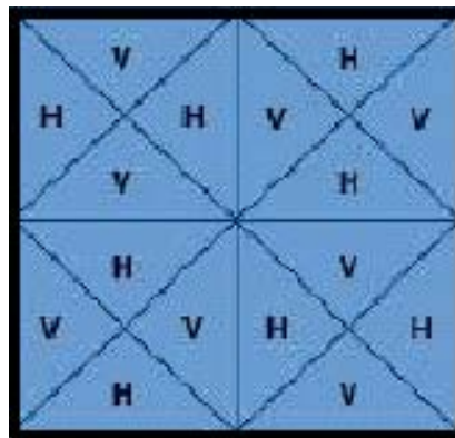
Figura 1.15. Re-uso de la polarización vertical y horizontal
