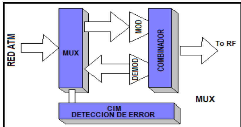
Figura 1.16. Arquitectura de Nodo de Red
