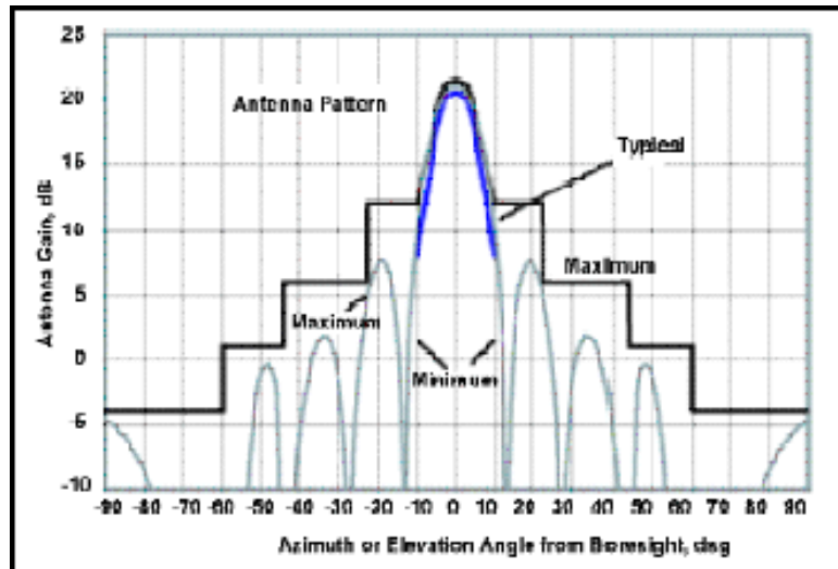
Figura 4.7 Azimuth/Elevación de la Antena
