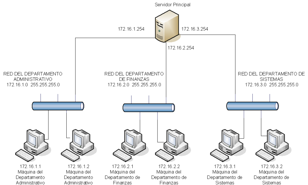
Figura 2.4. Esquema de la red del canal luego del enmascaramiento.
