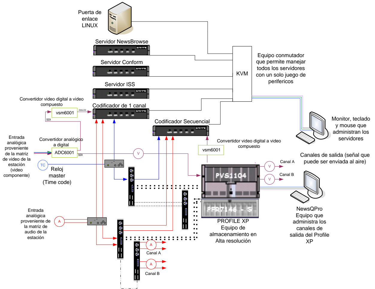
Figura 3.12. Conexiones entre equipos
