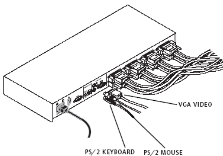
Figura 3.17. Equipo KVM.
