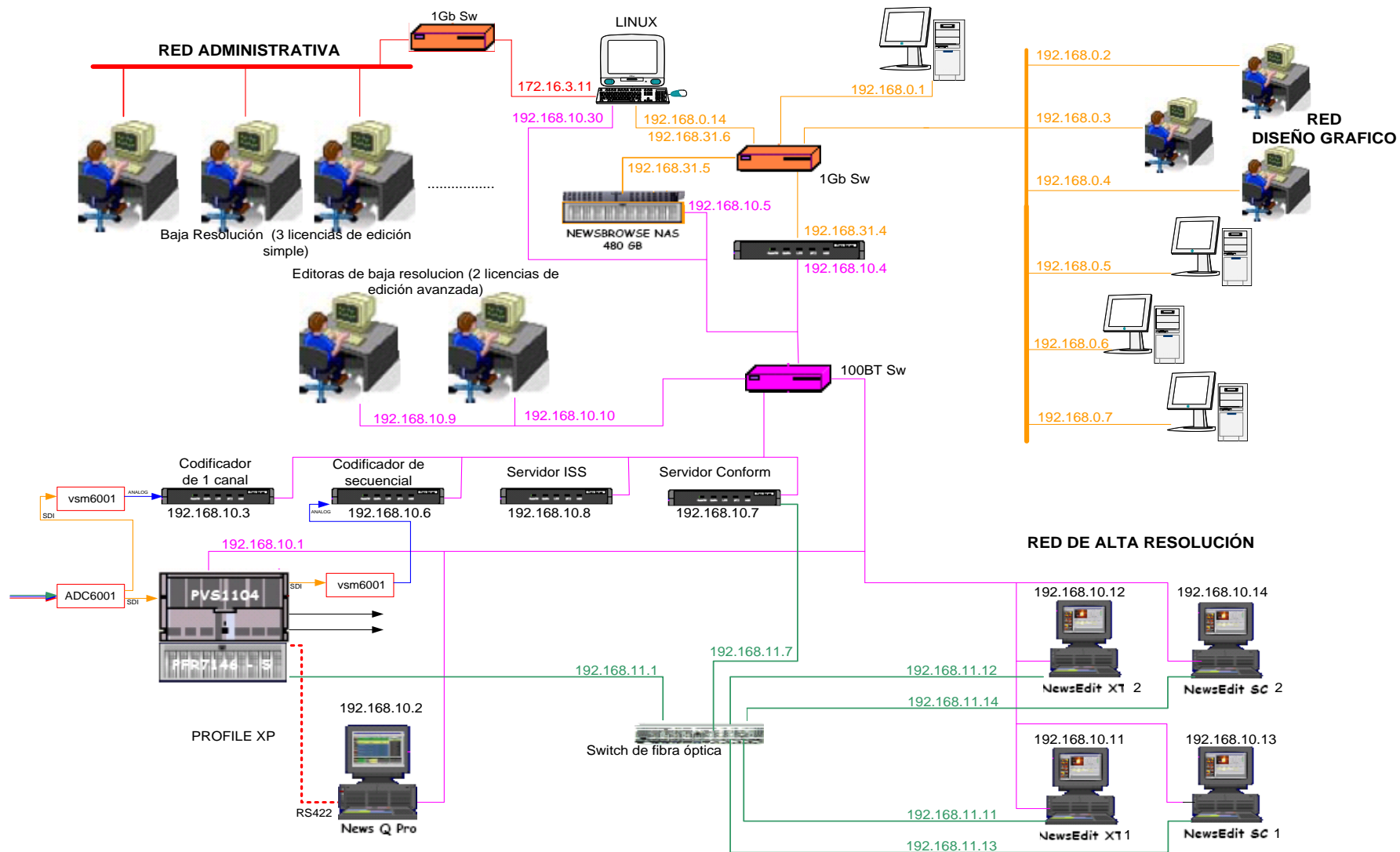
Figura 3.1a. Diseño general del sistema de edición digital
