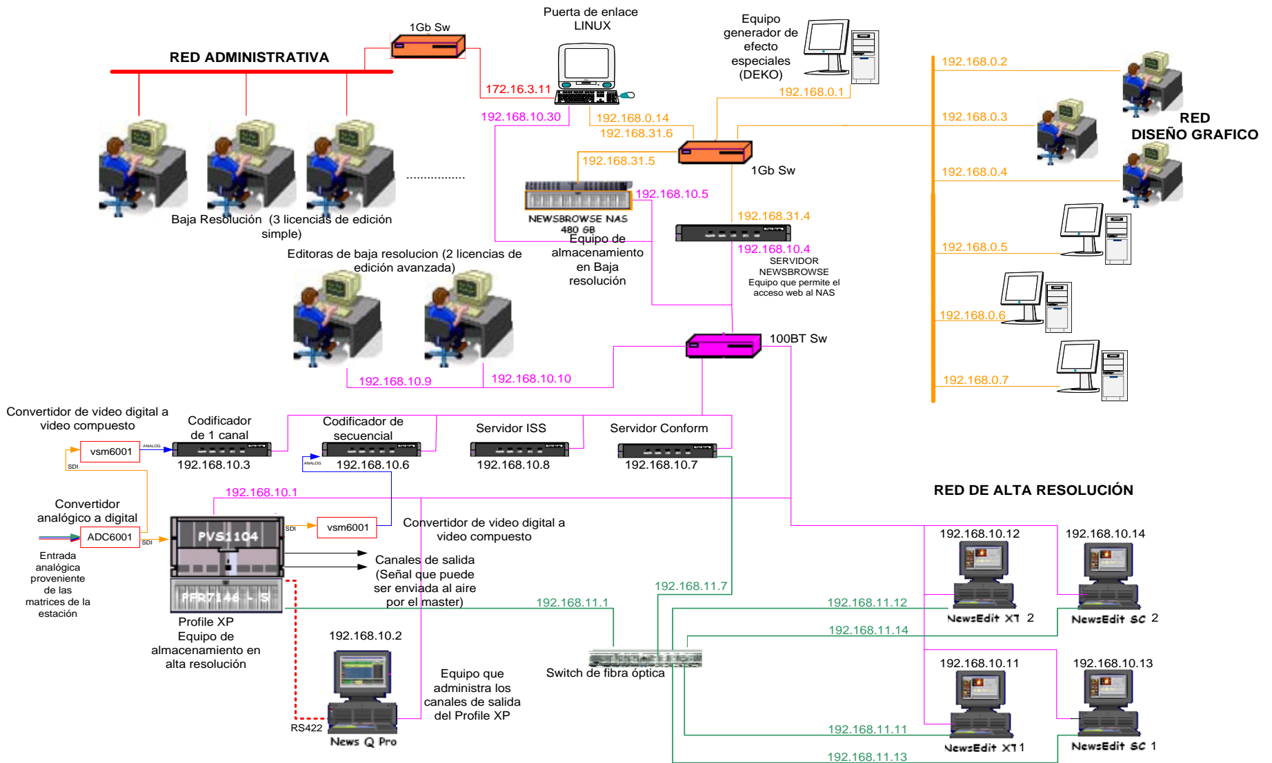
Figura 3.15. Esquema final de la red de edición digital
