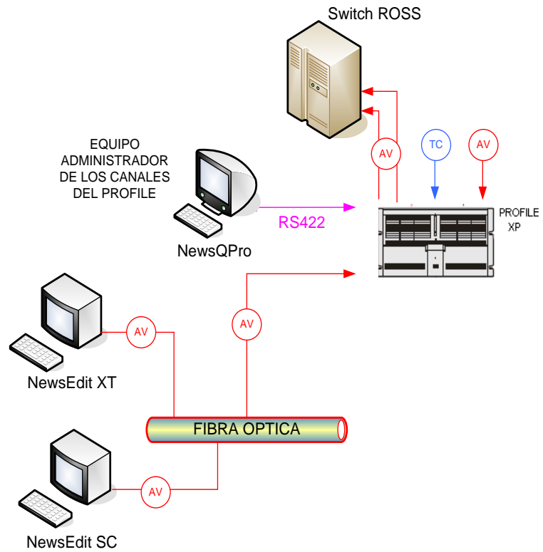
Figura 3.2. Proceso de edición en alta resolución
