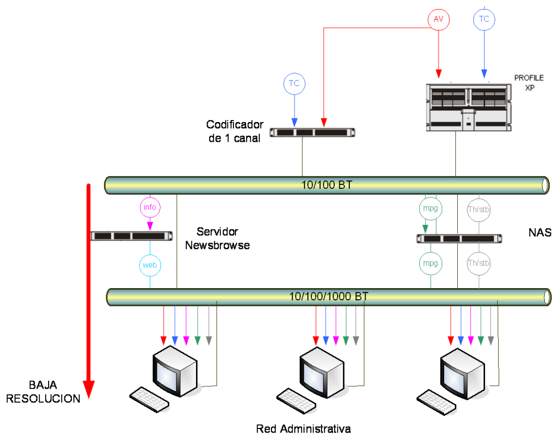
Figura 3.6. Conexión entre la red de edición digital y la red administrativa
