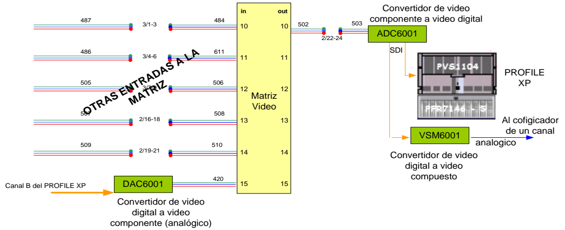
Figura 3.13. Entrada de canales de video a la matriz y al Switcher
