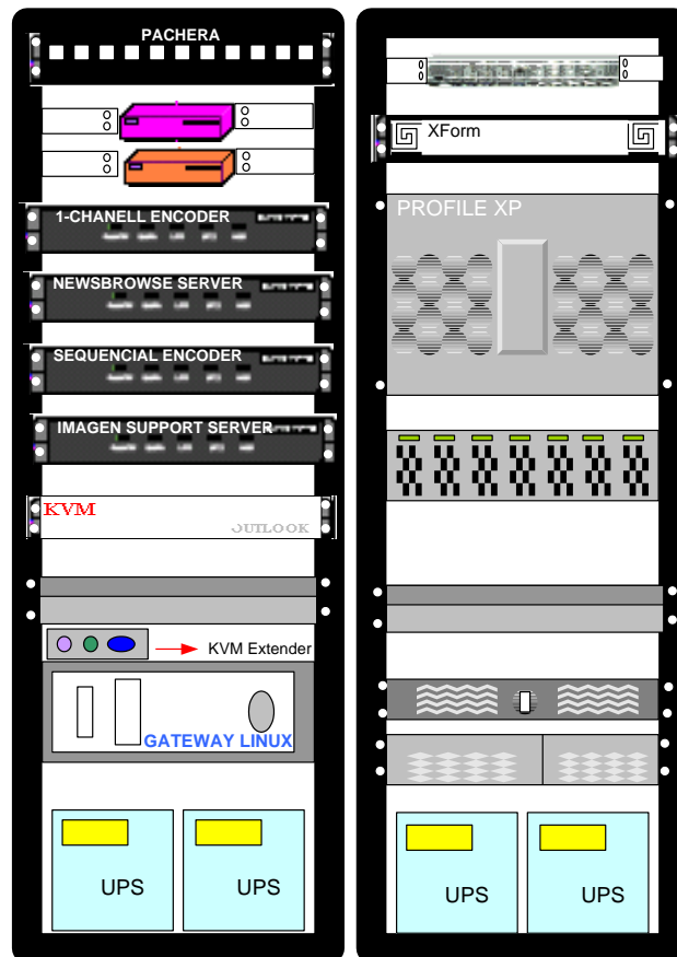
Figura 3.16. Distribución de los equipos en el cuarto de equipos
