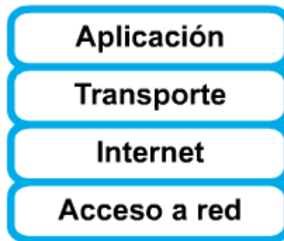
Figura 1.8. Modelo TCP/IP
