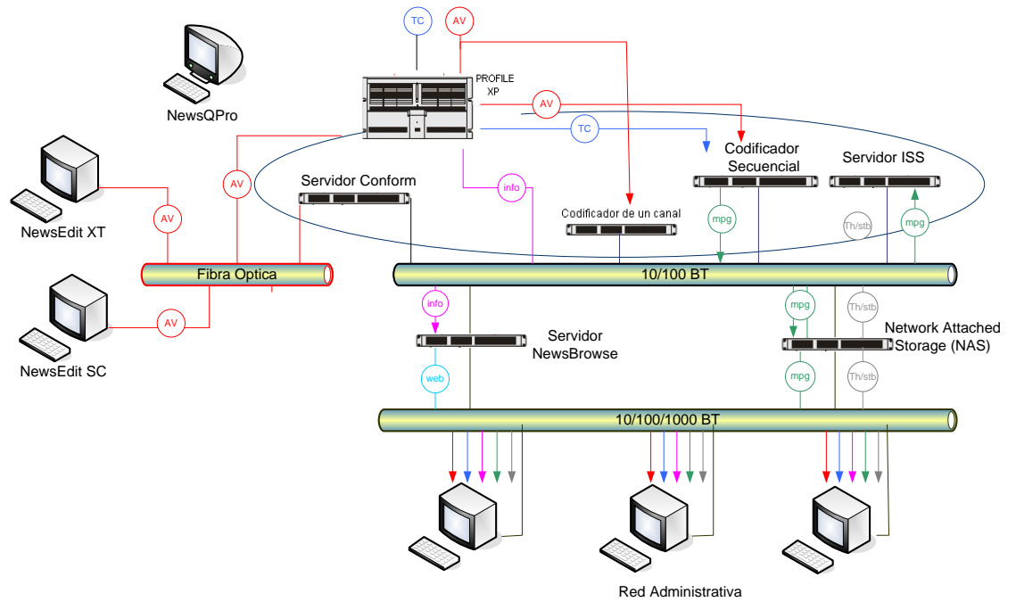
Figura 3.8. Sistema de edición no lineal (digital).
