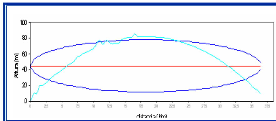
Fig. 55 Primera zonal de Fresnel de La Chivería – La Cadena
