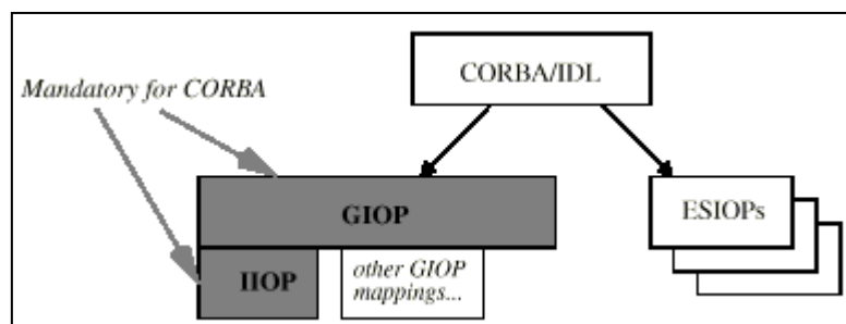
Figura 9. Capa elementos de Interoperabilidad
