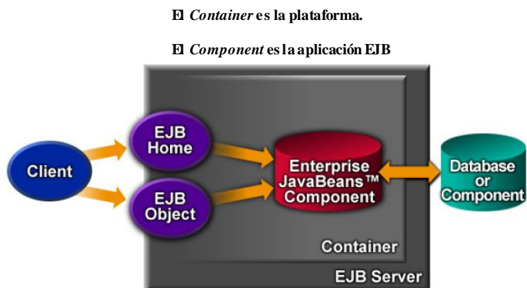
Figura 10. Arquitectura EJB.
