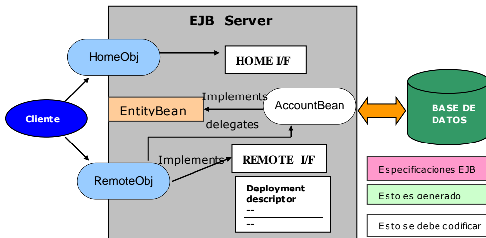
Figura 17. Deploy
