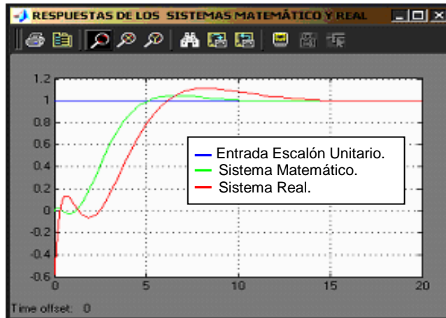
FIGURA 3.4.1.2. RESPUESTA DEL SISTEMA A 25 CM. DE NIVEL.
