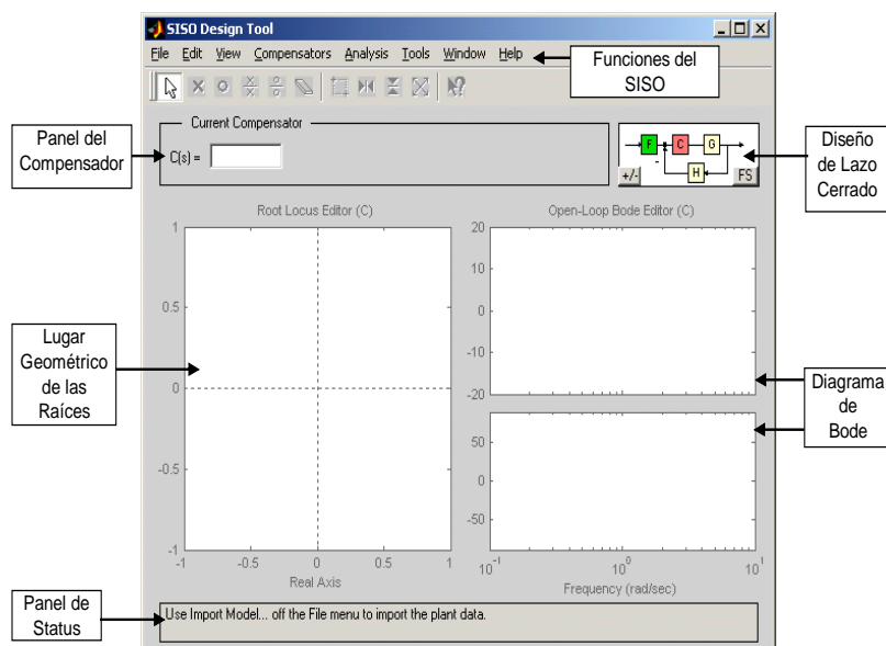
FIGURA 3.3.2.1. HERRAMIENTA SISO.
