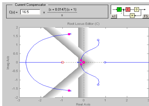
FIGURA 3.3.3.2.4. AGREGACIÓN DE DOS CEROS AL CONTROLADOR.
