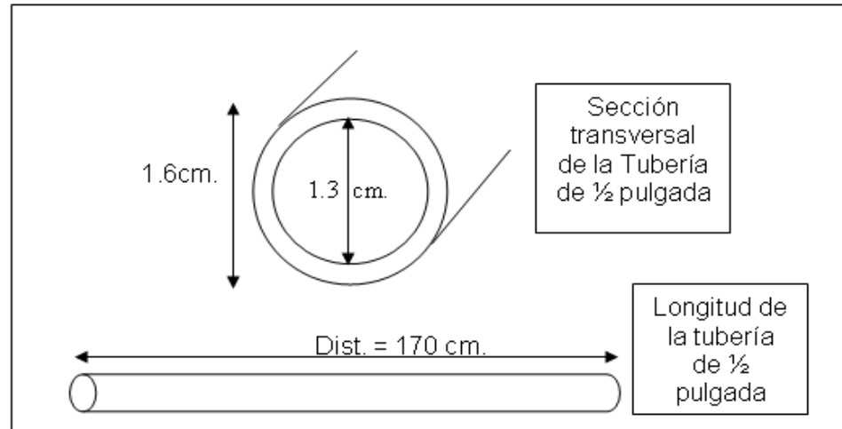
FIGURA 2.2.6. SECCIÓN TRANSVERSAL Y LONGITUD DE LA TUBERÍA DE ½ PULGADA UTILIZADA EN LA PLANTA.
