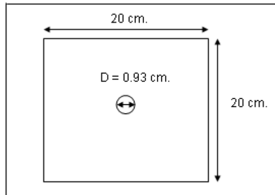
FIGURA 1.3.1.2. VISTA INFERIOR DEL TANQUE PRINCIPAL DE VIDRIO.
