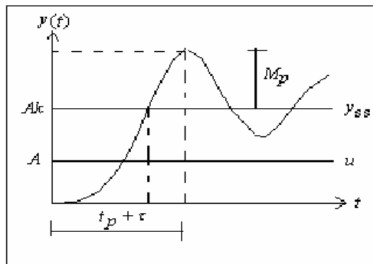
Figura 2. Método de Respuesta Transitoria. Modelo General de Segundo Orden.
