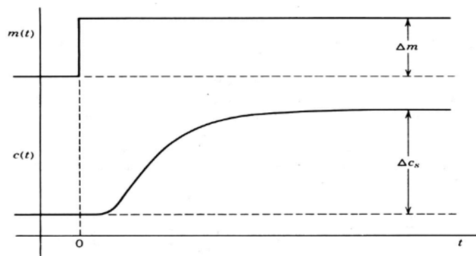
Figura 1. Respuesta a la entrada Escalón.
