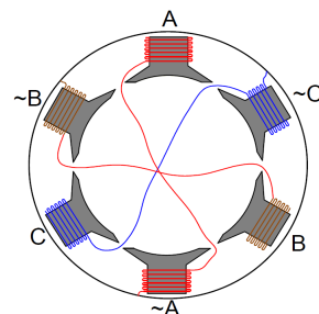
Figura 4. Devanados internos del motor BLDC (motor elemental).
