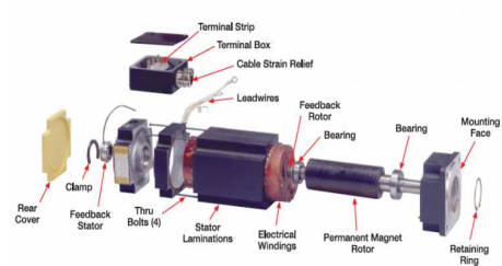
Figura 3. Despiece del Motor BLDC [1].
