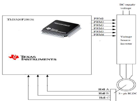
Figura 7. Sistema implementado con realimentación de sensores Hall.
