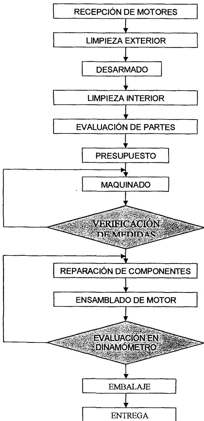
FIGURA 1.2 DIAGRAMA DE FLUJO DE REPARACIONES DE MOTORES
