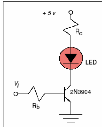
Figura 3.8. Esquema de un modulador digital básico.
