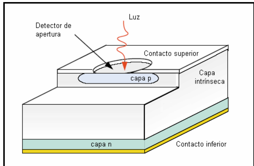
Figura 2.11. Corte transversal de un fotodiodo PIN.
