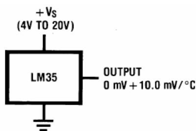
Figura 11.- Sensor de Temperatura LM35
