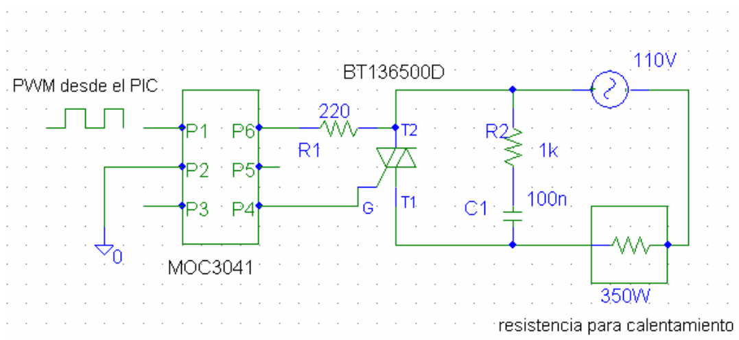
Figura 20.- Calentamiento del ambiente en la incubadora
