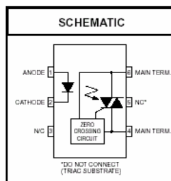
Figura 18.- Top view del MOC3041M
