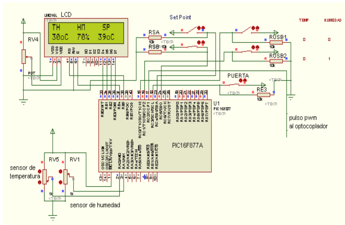
Figura 24.- Microcontrolador PIC16F877A
