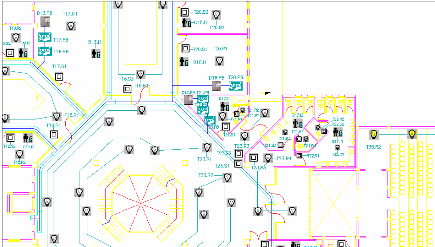
FIGURA 3.37 PLANO ILUMINACION PLANTA BAJA SECCION 5
