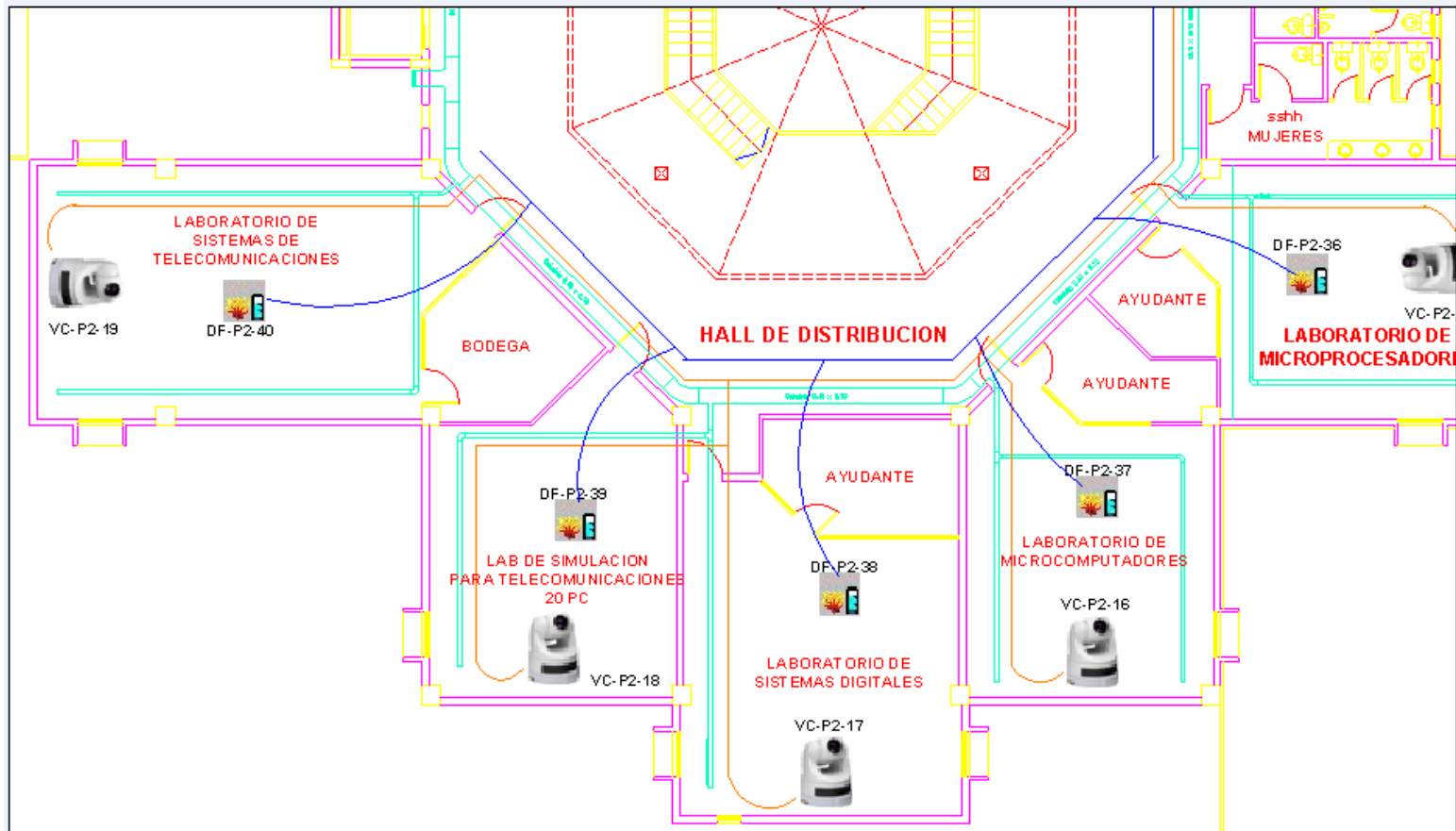
FIGURA 3.80 PLANO SEGURIDAD SEGUNDO PISO SECCION 3
