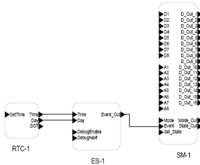
FIGURA 3.60 BLOQUES FUNCIONALES DEL CONTROLADOR DE EVENTOS
