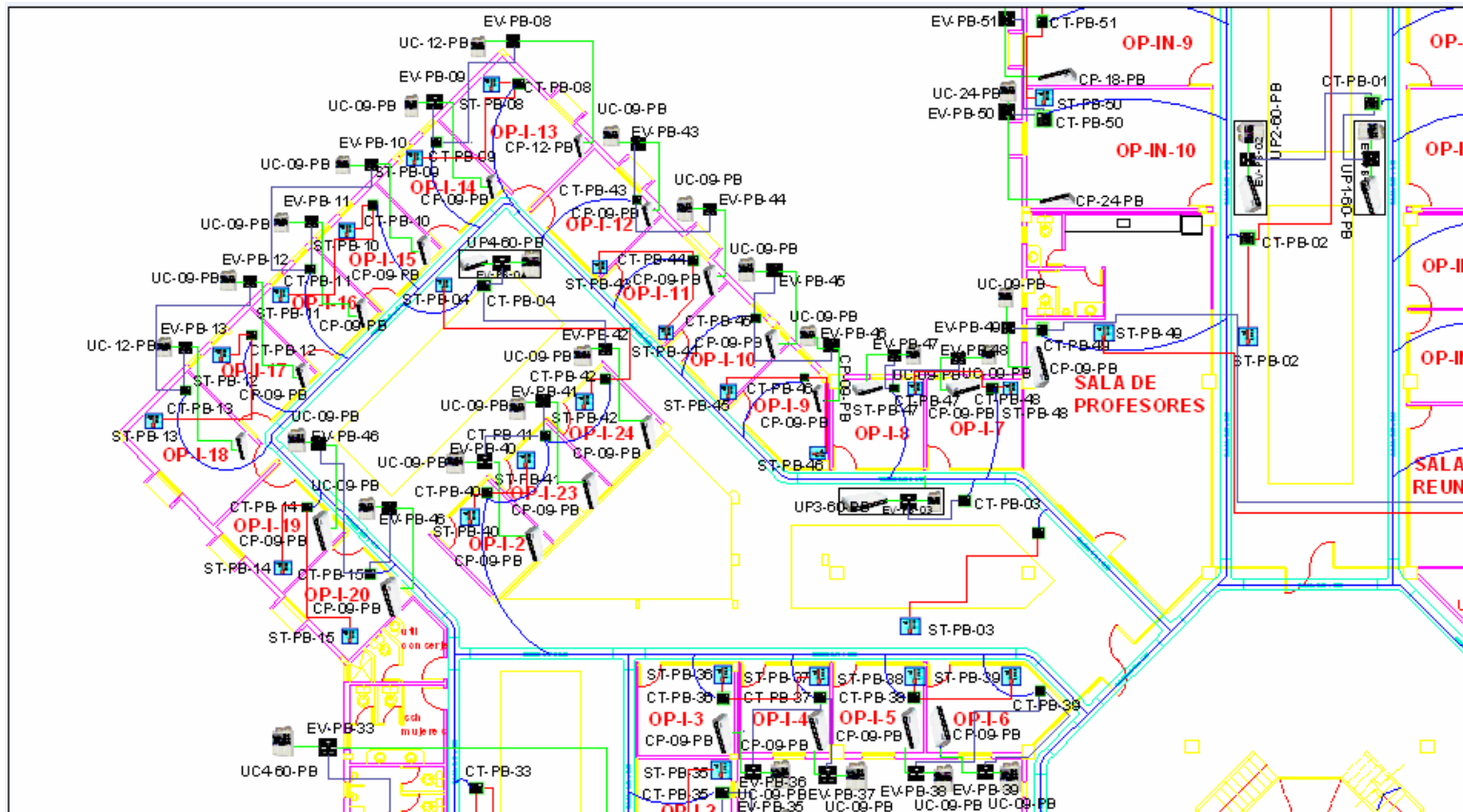
FIGURA 3.5 PLANO CLIMATIZACIÓN PLANTA BAJA SECCION 2
