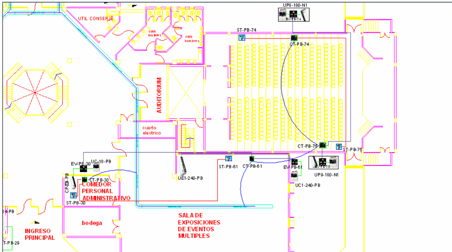
FIGURA 3.7 PLANO CLIMATIZACIÓN PLANTA BAJA SECCION 4
