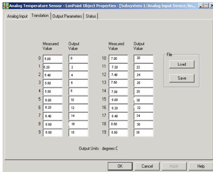
FIGURA 3.24 TRASLACION DE ENTRADA ANALÓGICA EN VOLTIOS A TEMPERATURA EN CELSIUS
