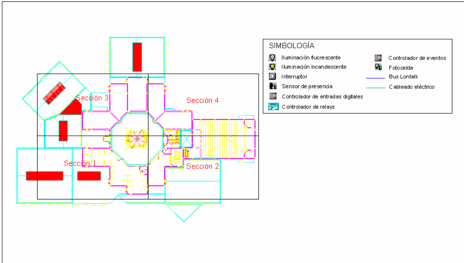
FIGURA 3.41 PLANO ILUMINACIÓN PRIMER PISO GENERAL
