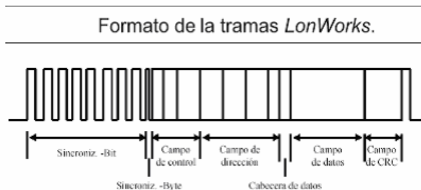
FIGURA 1.19 FORMATO DE LA TRAMA LONWORKS
