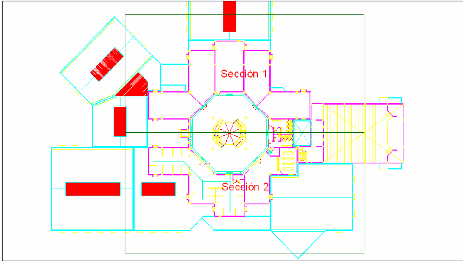
FIGURA 3.8 PLANO CLIMATIZACIÓN PRIMER PISO GENERAL
