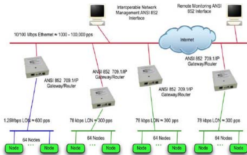
FIGURA 3.94 APLICACIÓN CON BACKBONE IP
