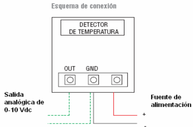
FIGURA 3.14 ESQUEMA DE CONEXIÓN SENSOR DE TEMPERATURA
