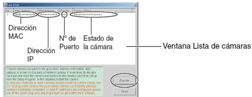
FIGURA 3.90 DETECCIÓN DE CAMARAS
