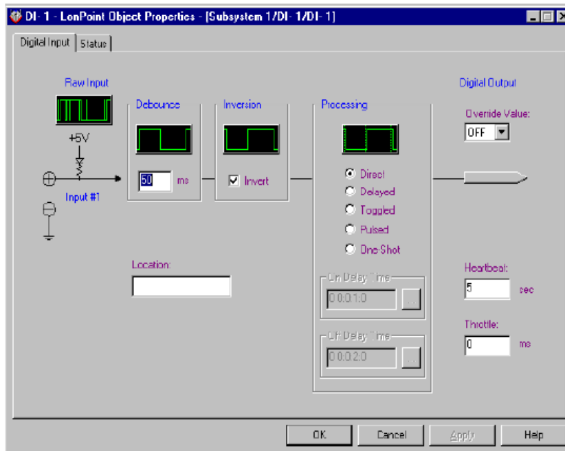
FIGURA 3.27 VENTANA PARA CONFIGURACION DE ENTRADA DIGITAL
