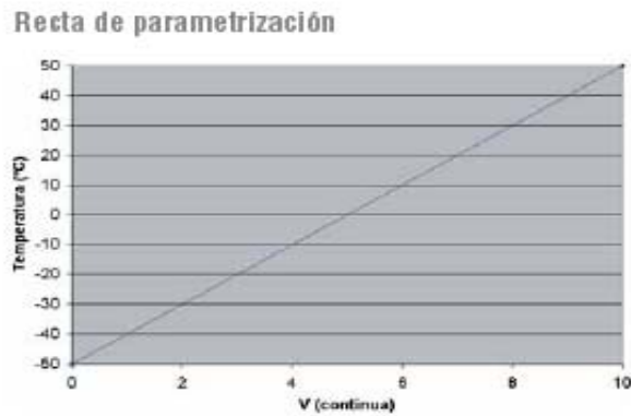
FIGURA 3.15 RECTA DE PARAMETRIZACIÓN TEMPERATURA (°C) VS. VOLTAJE [V]
