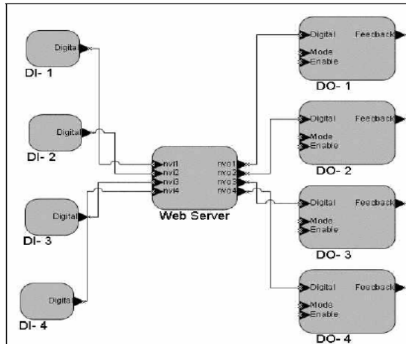
FIGURA 3.106 EJEMPLO DE BLOQUES FUNCIONALES PARA CONTROL REMOTO A TRAVES DEL Lon 100
