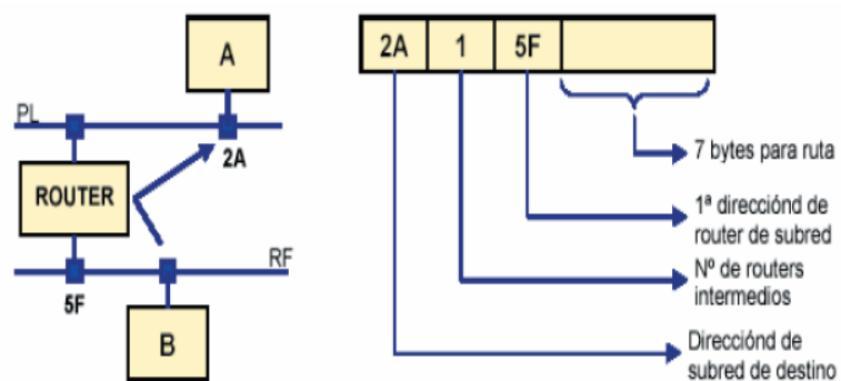
FIGURA 1.16 DIRECCIONAMIENTO DE SUBREDES EHS
