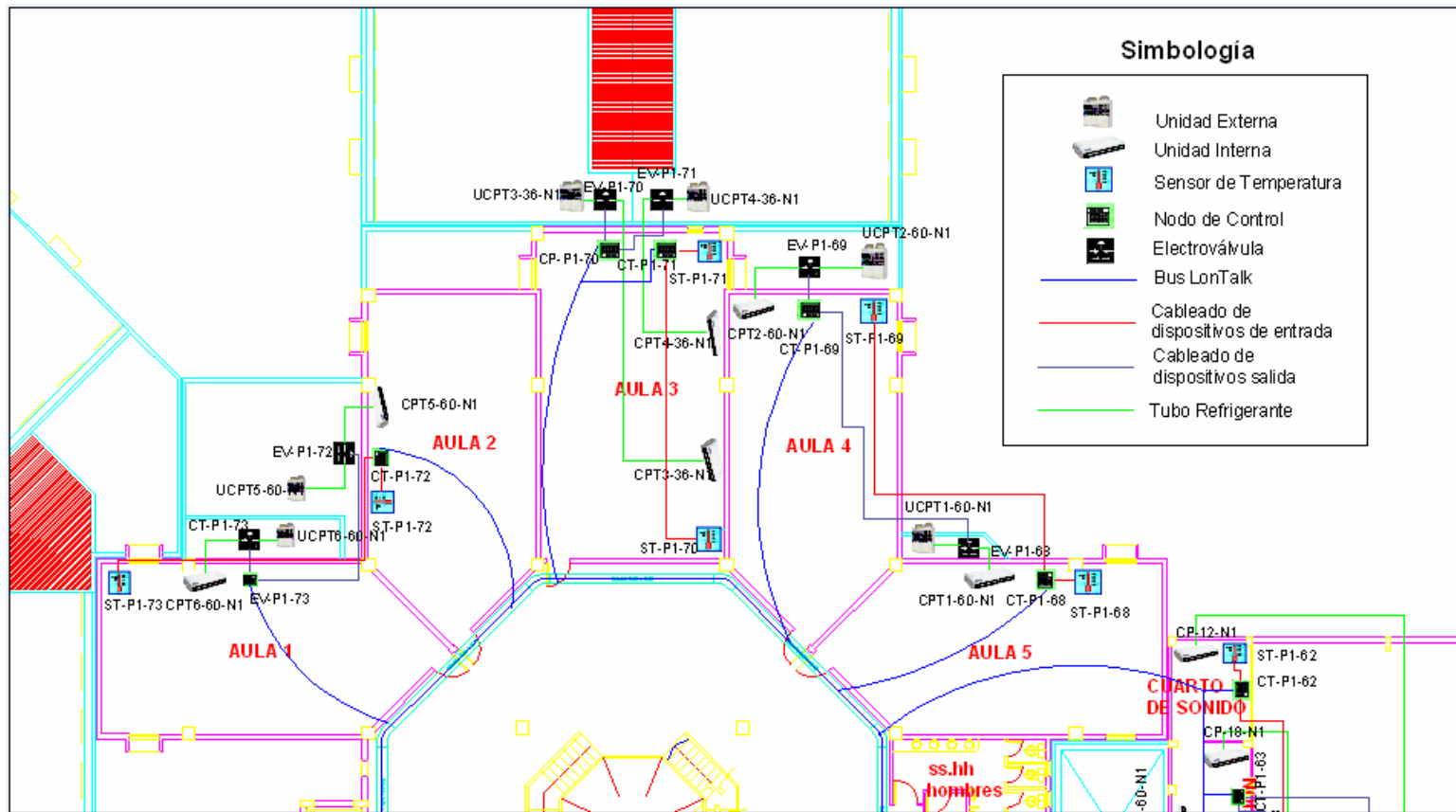
FIGURA 3.9 PLANO CLIMATIZACIÓN PRIMER PISO SECCION 1
