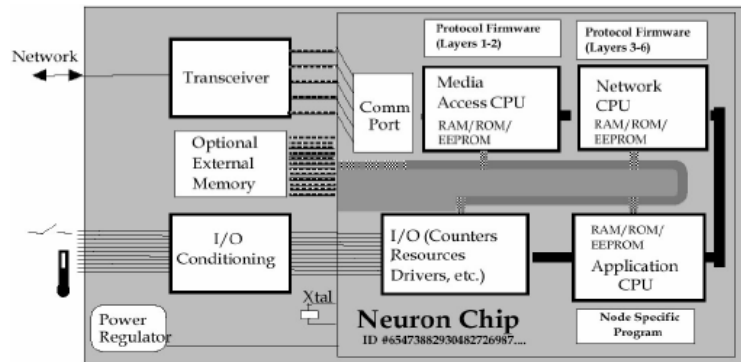
FIGURA 1.25 ESQUEMA MODULAR DE UN INTERFAZ LONWORKS DE UN NODO DE SU RED
