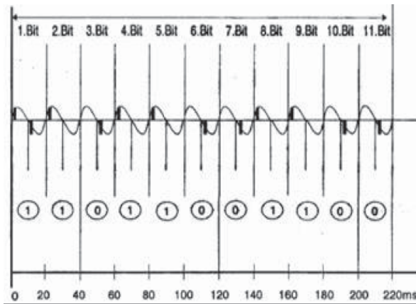
FIGURA 1.13 ESTRUCTURA DE UN DATAGRAMA X-10
