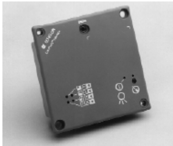
FIGURA 3.55 CONTROLADOR DE ENTRADAS DIGITALES DI-10 MODELO 41100
