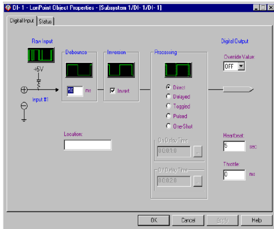
FIGURA 3.58 BLOQUE FUNCIONAL ENTRADA DIGITAL
