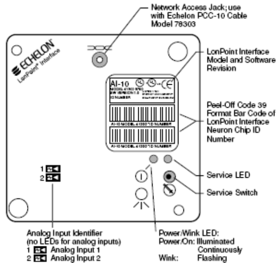
FIGURA 3.20 INTERFASE DE ENTRADAS ANALÓGICAS LONPOINT
