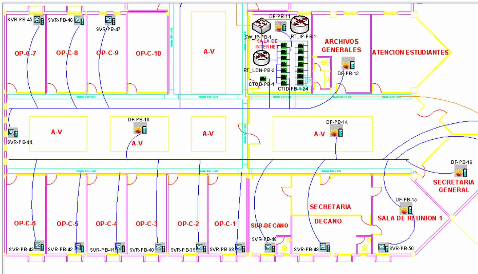
FIGURA 3.72 PLANO SEGURIDAD PLANTA BAJA SECCION 6
