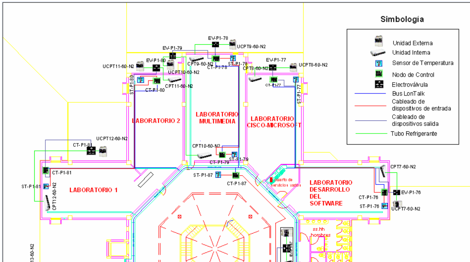
FIGURA 3.12 PLANO CLIMATIZACIÓN SEGUNDO PISO SECCION 1
