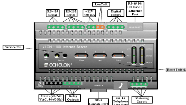
FIGURA 3.98 CONEXIONES DEL SERVIDOR Iion 100
