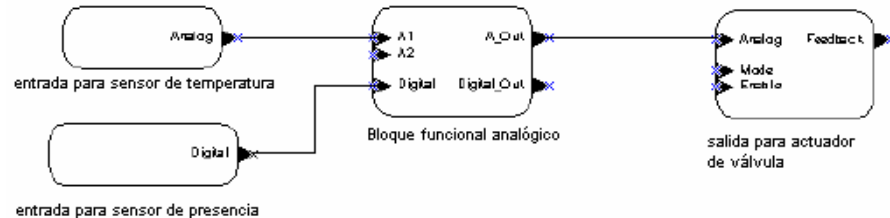
FIGURA 3.23 BLOQUES FUNCIONALES CONECTADOS PARA CONTROL DE CLIMATIZACION
