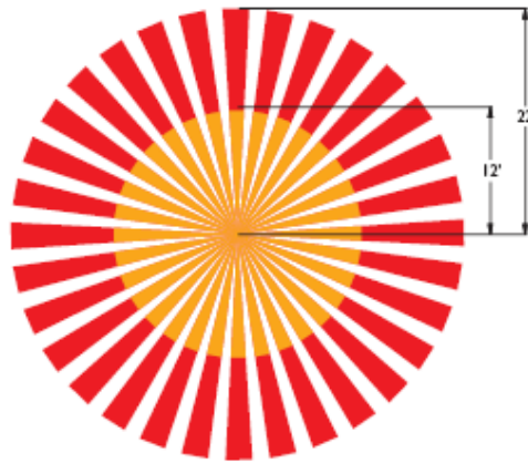
FIGURA 3.50 PATRÓN DE COBERTURA DE SENSOR PASIVO INFRARROJO DE MONTAJE EN CIELO RASO
