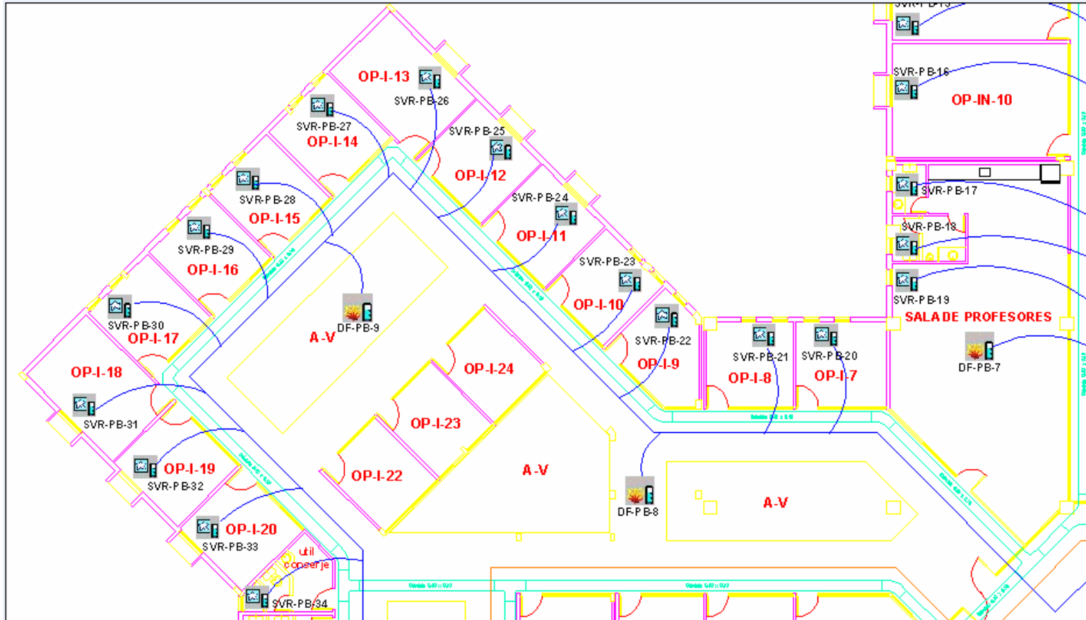
FIGURA 3.70 PLANO SEGURIDAD PLANTA BAJA SECCION 4
