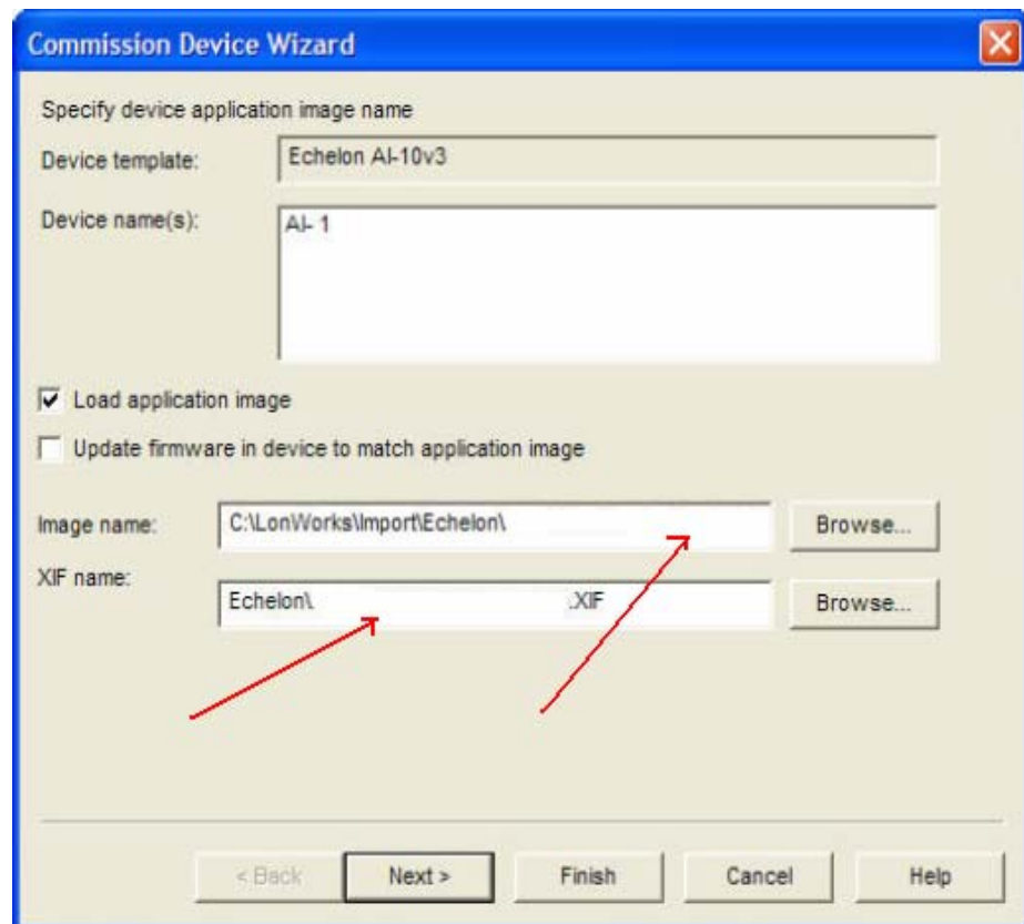
FIGURA 3.59 COMISIONAMIENTO DE DISPOSITIVOS
