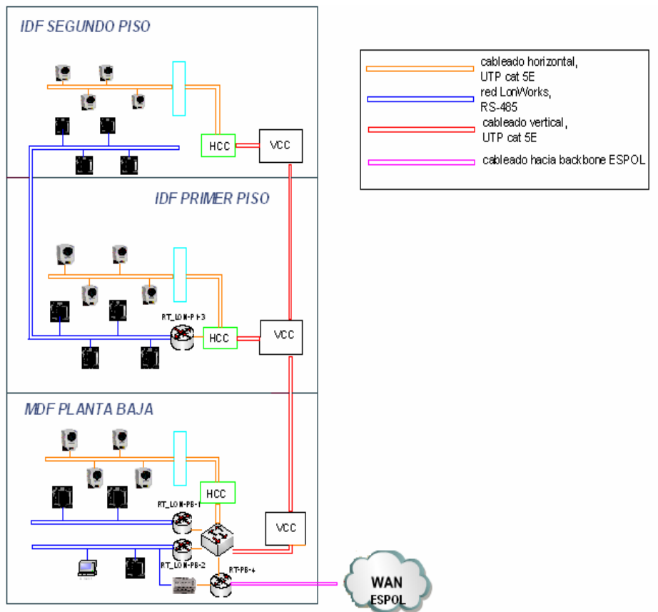
FIGURA 3.93 CABLEADO HORIZONTAL Y VERTICAL EDIFICIO FIEC
