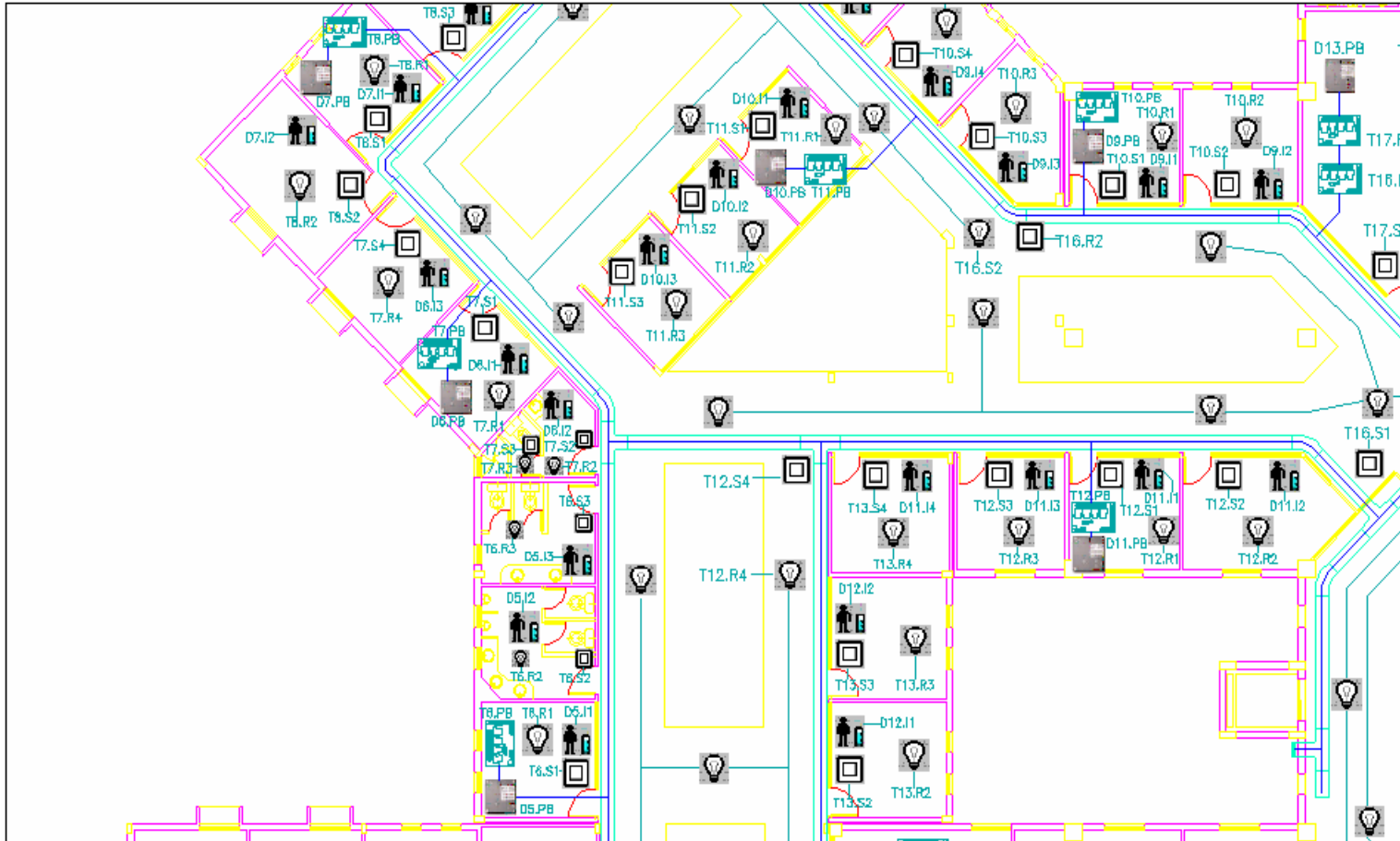
FIGURA 3.36 PLANO ILUMINACION PLANTA BAJA SECCION 4
