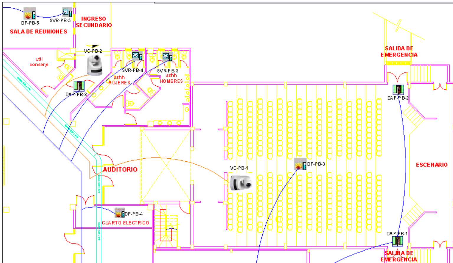
FIGURA 3.68 PLANO SEGURIDAD PLANTA BAJA SECCION 2
