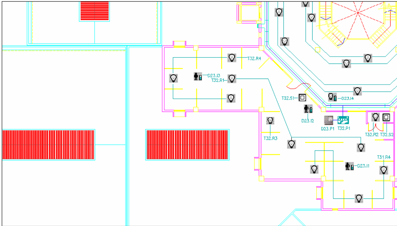
FIGURA 3.42 PLANO ILUMINACION PRIMER PISO SECCION 1
