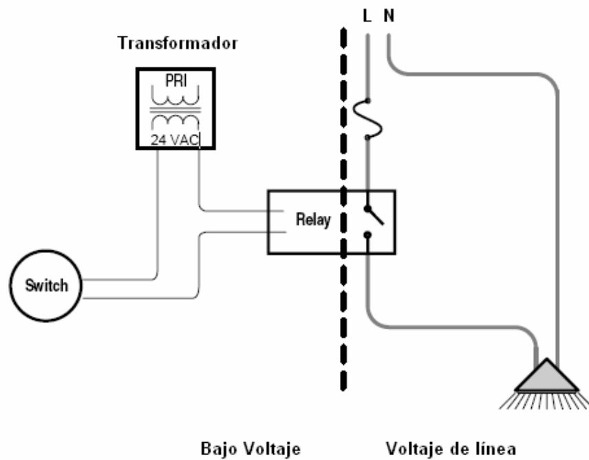
FIGURA 3.29 CONTROL DE CIRCUITO MEDIANTE RELAY
