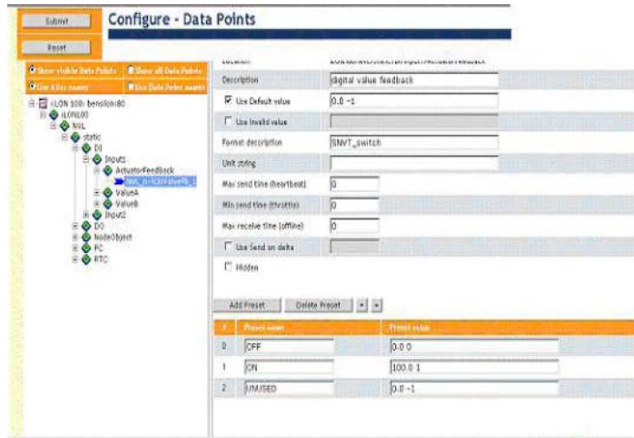
FIGURA 3.109 CONFIGURACION DE PUNTOS DE DATO
