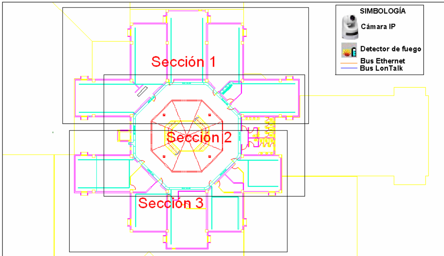
FIGURA 3.77 PLANO SEGURIDAD SEGUNDO PISO GENERAL
