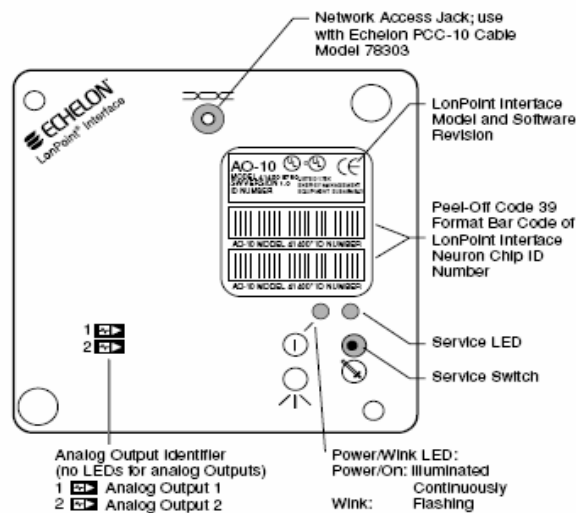
FIGURA 3.21 INTERFASE DE SALIDAS ANALÓGICAS LONPOINT
