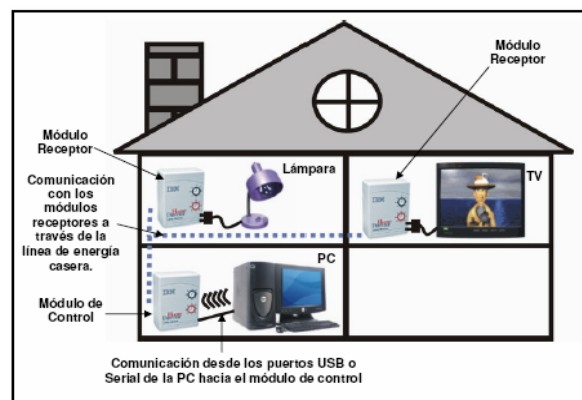
FIGURA 1.12 ESQUEMA GENERAL DEL FUNCIONAMIENTO DE LA TECNOLOGIA X-10
