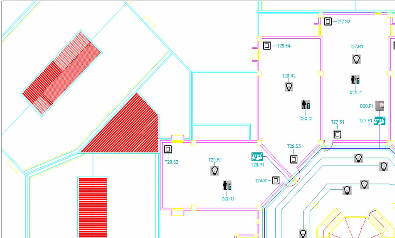
FIGURA 3.44 PLANO ILUMINACION PRIMER PISO SECCION 3
