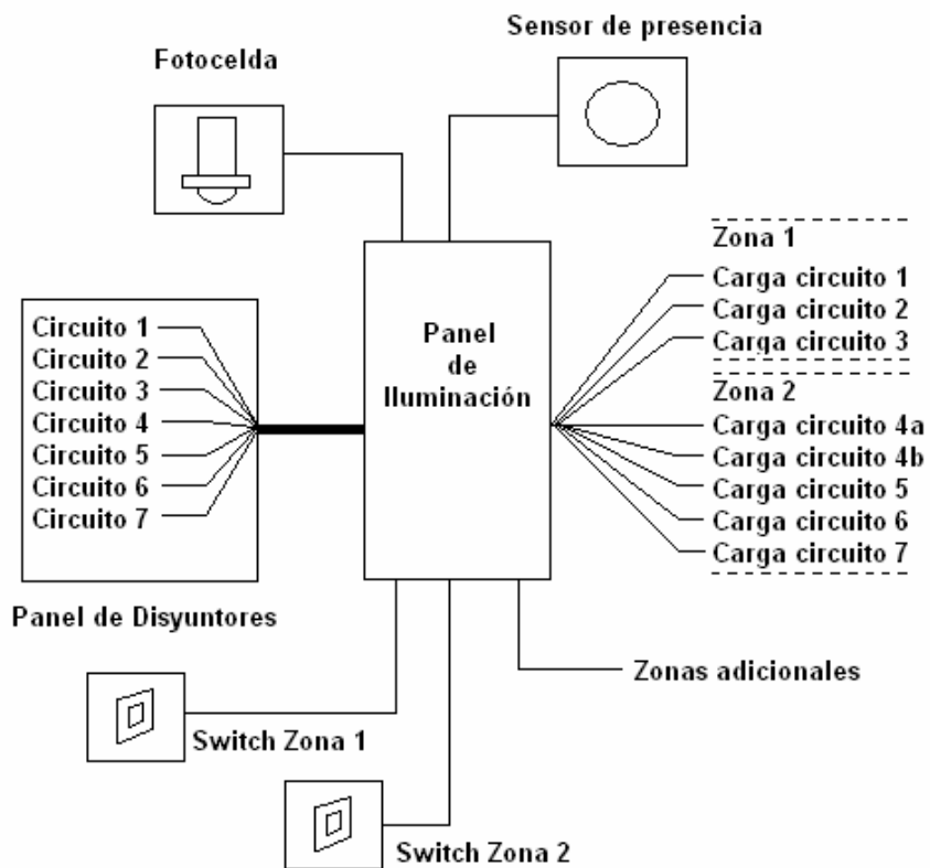
FIGURA 3.30 DIAGRAMA DE PANEL DE ILUMINACIÓN
