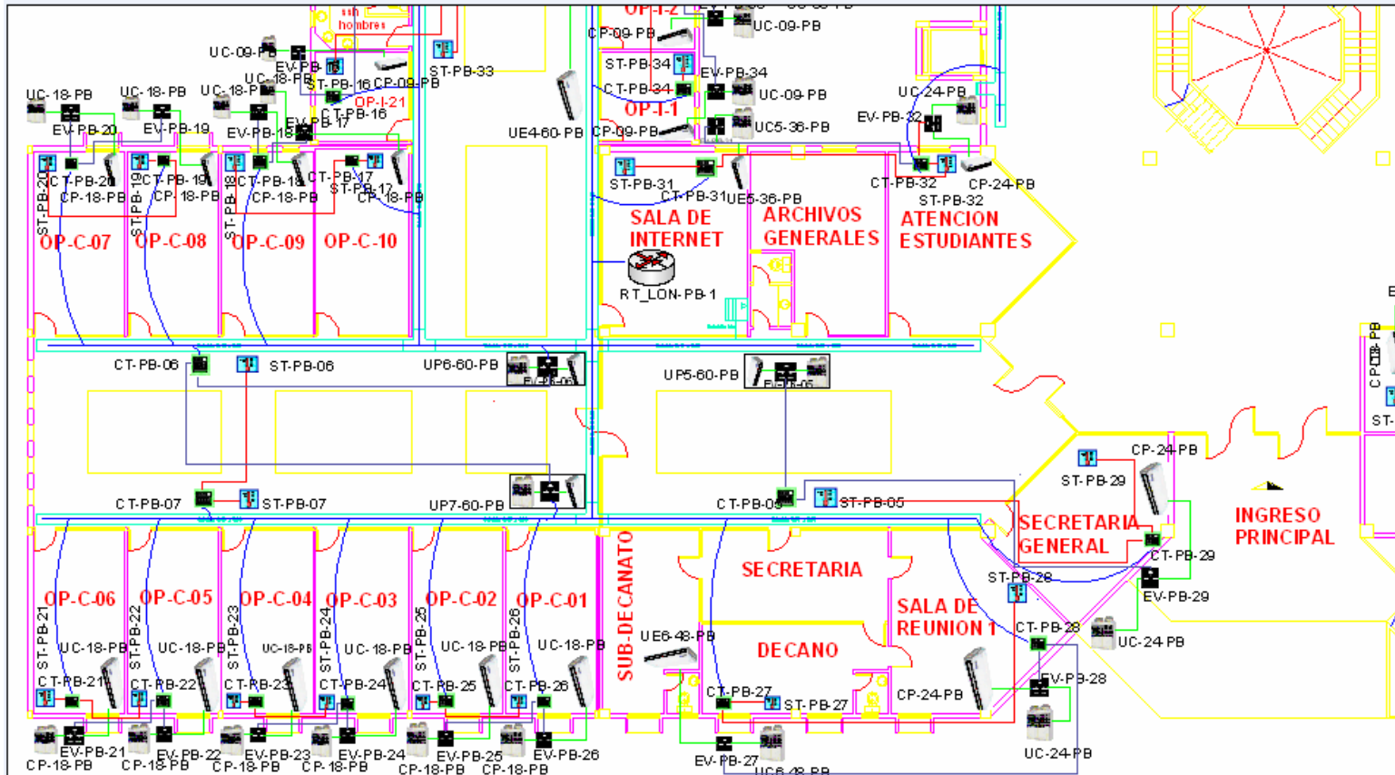
FIGURA 3.6 PLANO CLIMATIZACIÓN PLANTA BAJA SECCION 3
