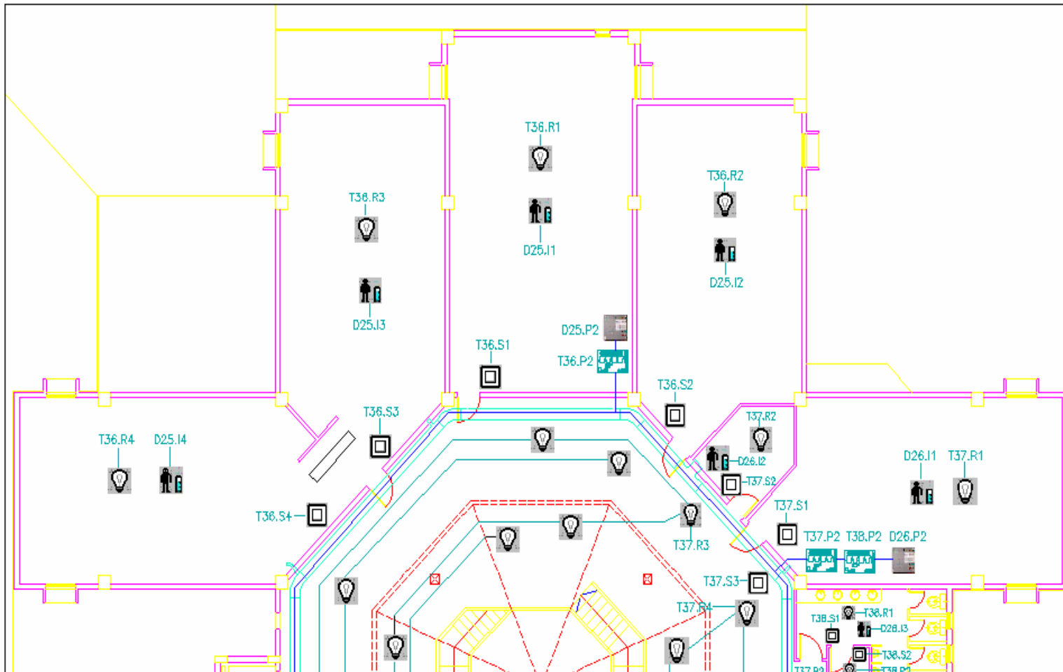
FIGURA 3.48 PLANO ILUMINACION SEGUNDO PISO SECCION 2
