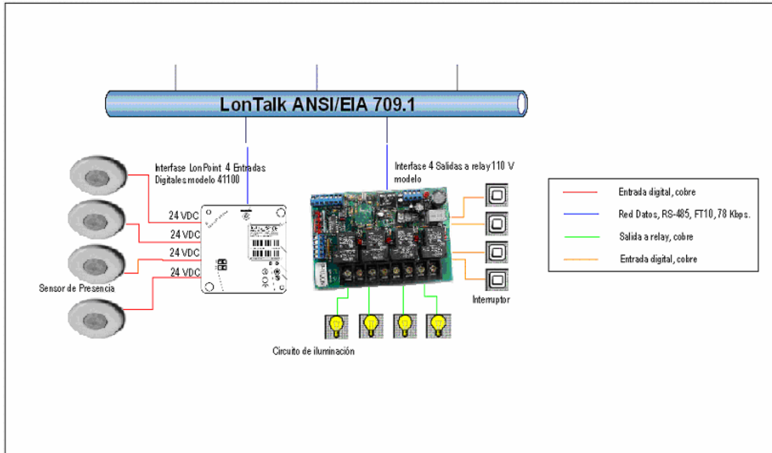
FIGURA 3.31 DIAGRAMA FISICO CONTROL DE ILUMINACION
