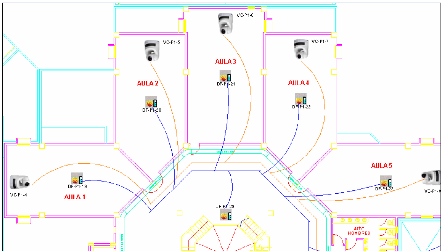
FIGURA 3.74 PLANO SEGURIDAD PRIMER PISO SECCION 1
