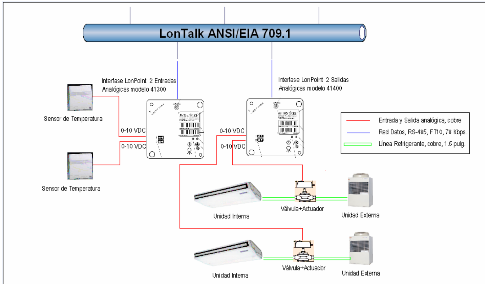
FIGURA 3.2 DIAGRAMA FISICO CONTROL DE CLIMATIZACIÓN
