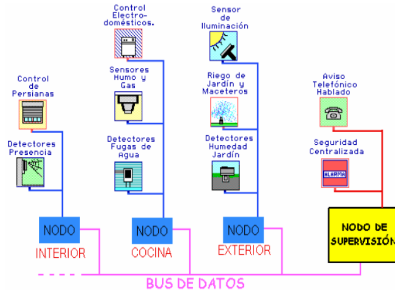
FIGURA 1.4 DISTRIBUCIÓN FÍSICA DE LOS ELEMENTOS DE CONTROL
