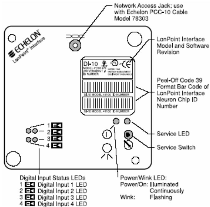
FIGURA 3.85 INTERFASE DE ENTRADAS DIGITALES LONPOINT
