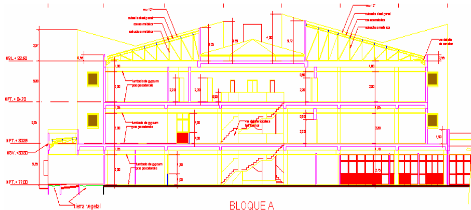
FIGURA 2.4 VISTA FRONTAL DEL EDIFICIO
