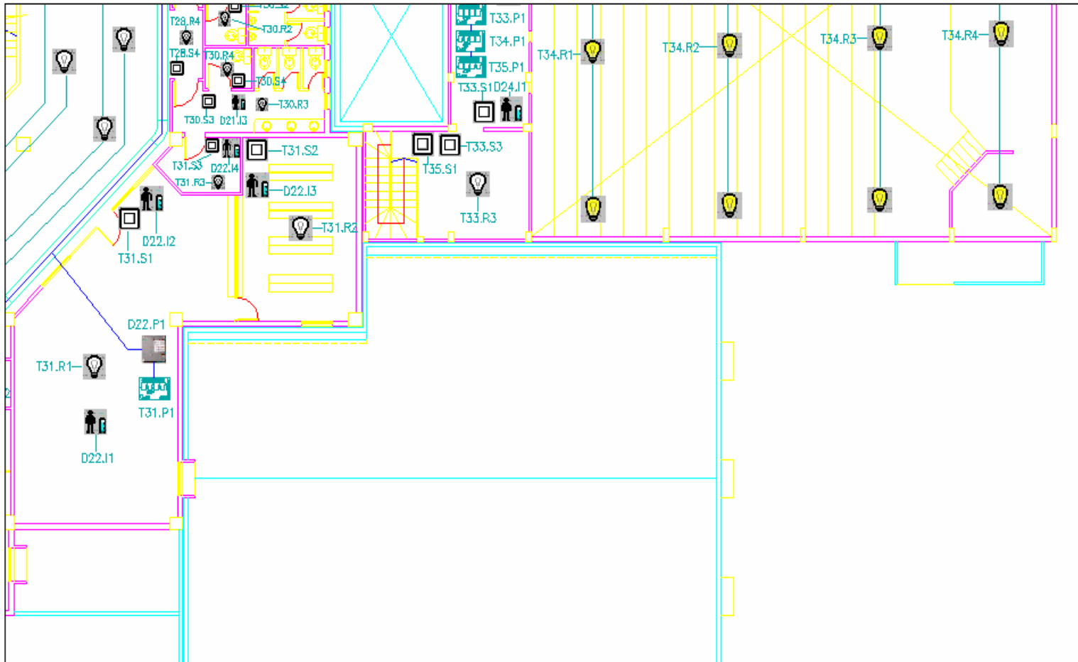
FIGURA 3.43 PLANO ILUMINACION PRIMER PISO SECCION 2
