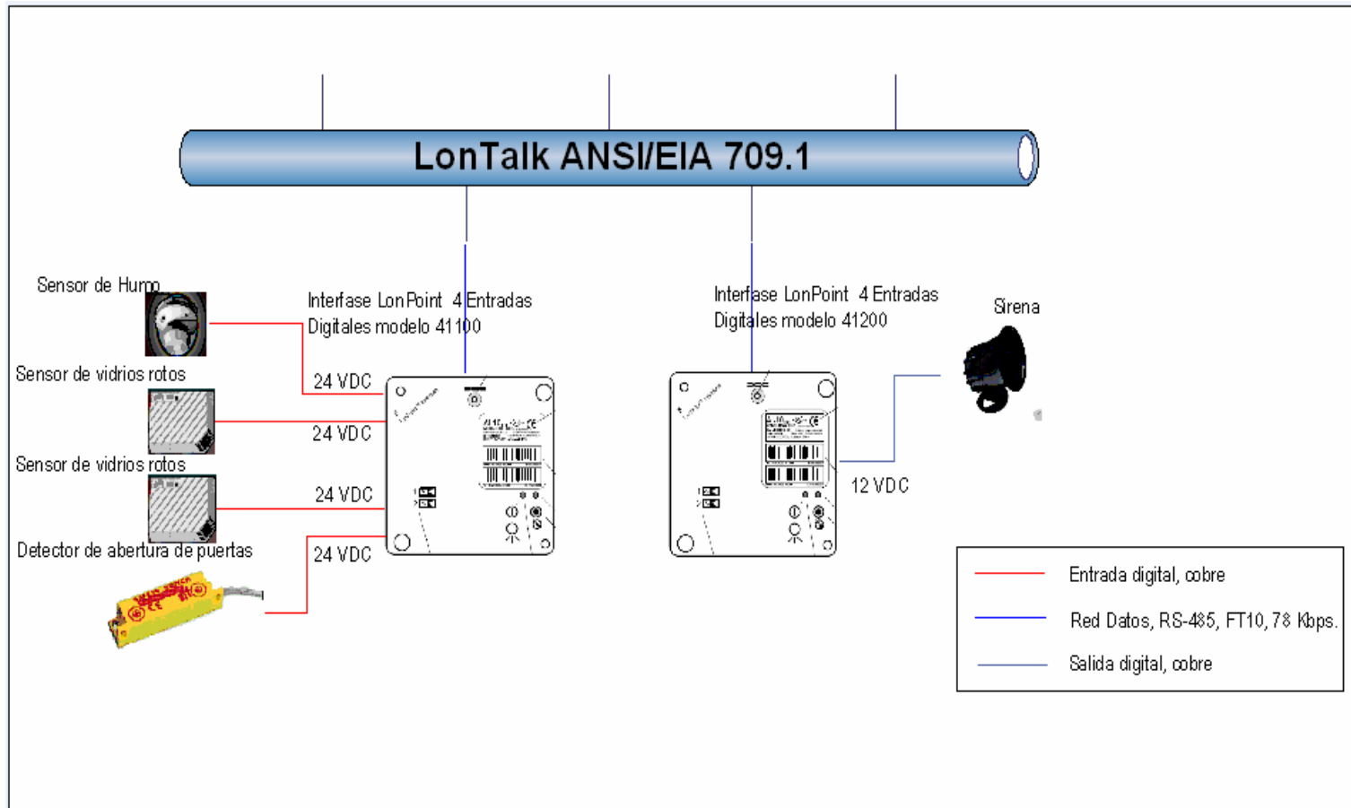
FIGURA 3.65 DIAGRAMA FISICO CONTROL DE SEGURIDAD (RED LONWORKS)
