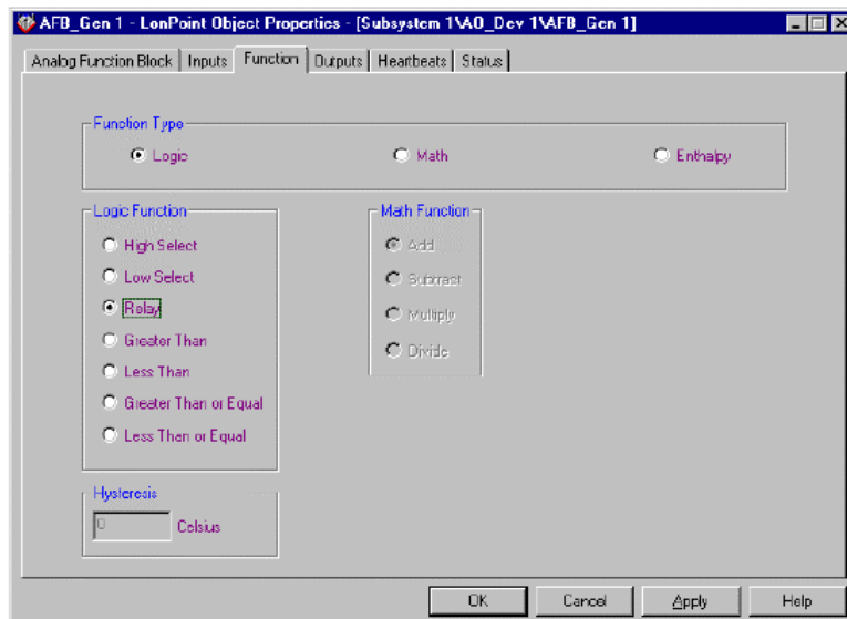
FIGURA 3.26 VENTANA PARA CONFIGURACION DE FUNCION PARA ENTRADAS ANALOGICAS
