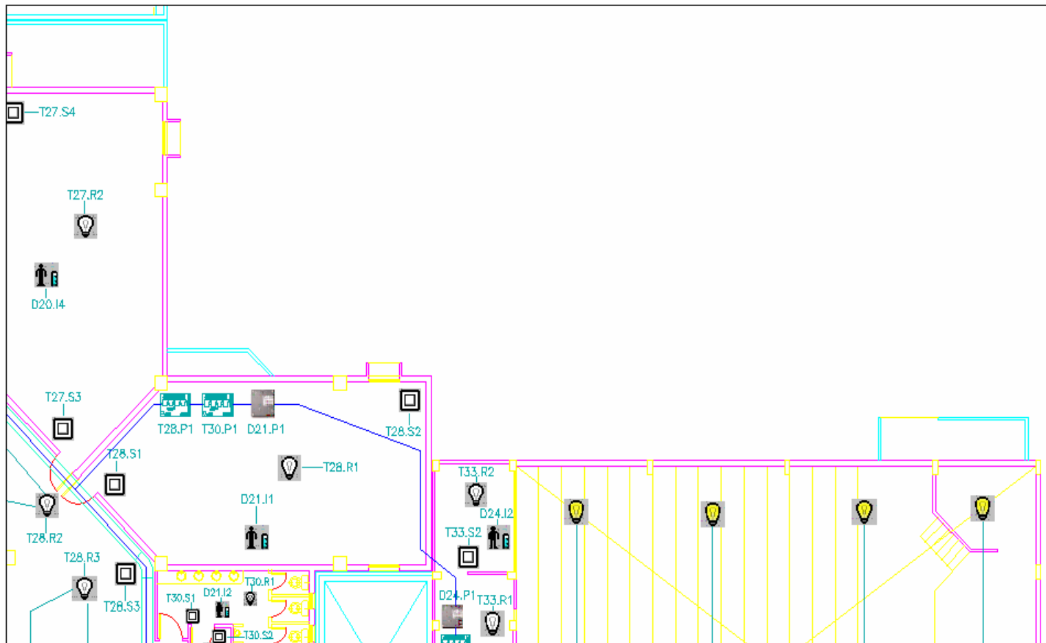
FIGURA 3.45 PLANO ILUMINACION PRIMER PISO SECCION 4
