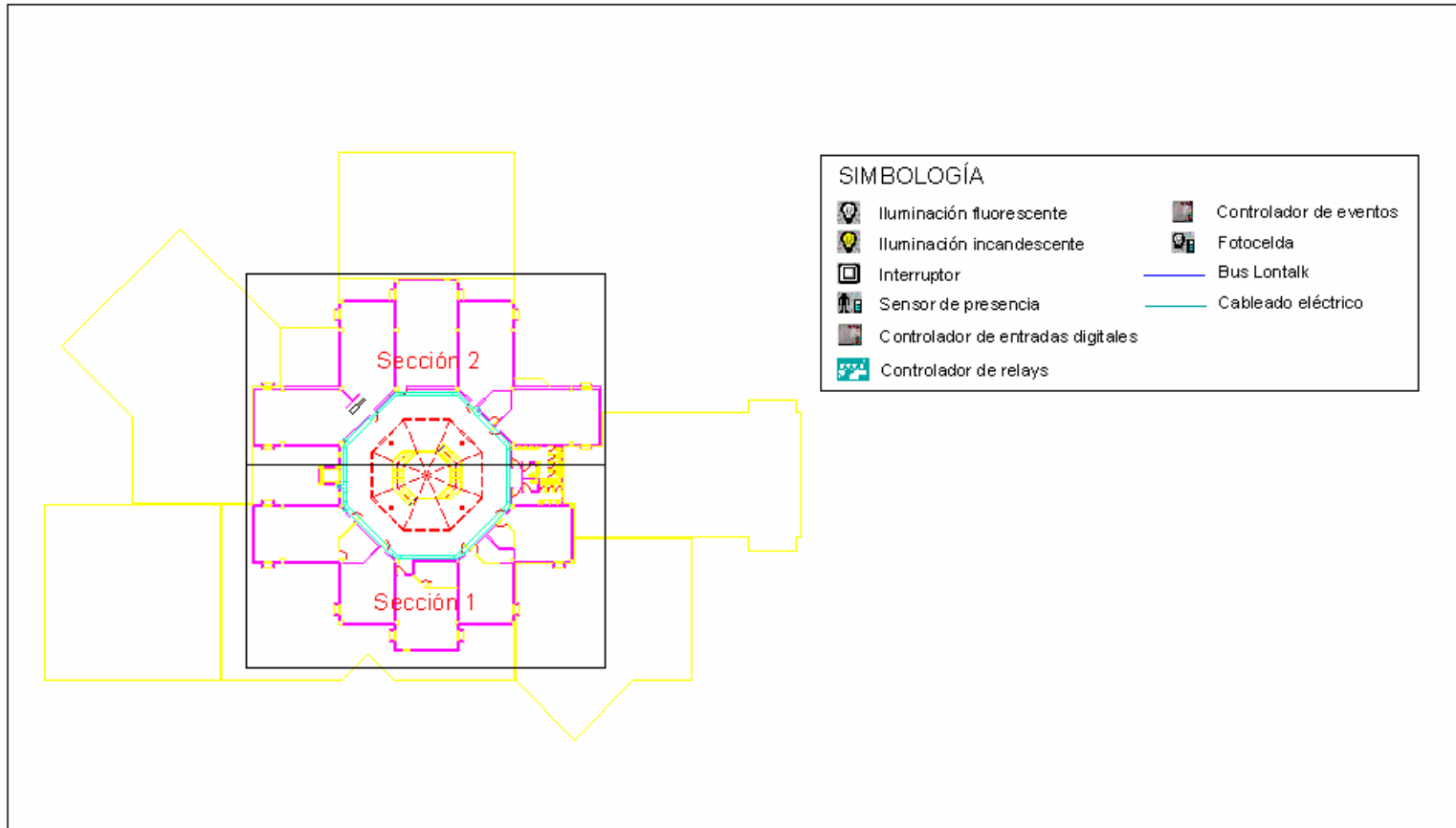
FIGURA 3.46 PLANO IILUMINACIÓN SEGUNDO PISO GENERAL
