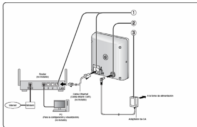
FIGURA 3.88 INSTALACIÓN DE CÁMARA IP
