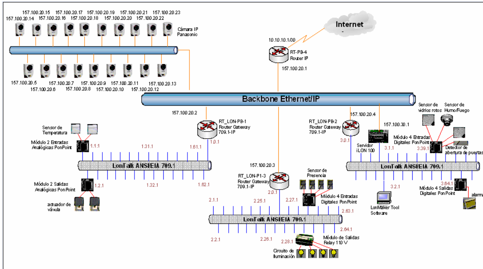
3.1 DIAGRAMA GENERAL DE LA RED PARA AHORRO ENERGÉTICO, SEGURIDAD Y CONTROL DE LAS INSTALACIONES
