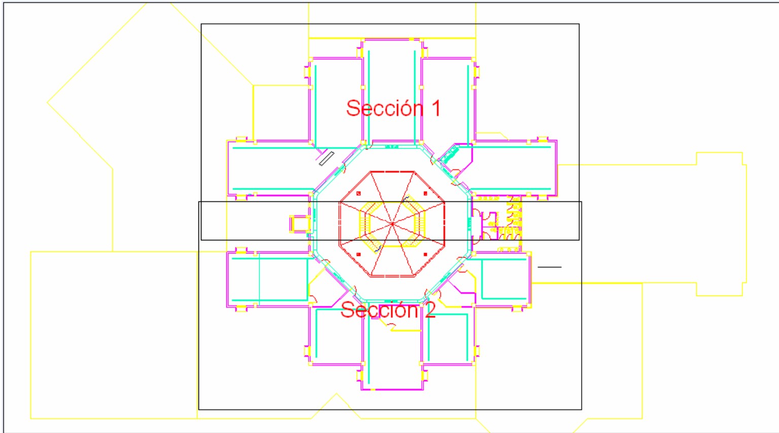
FIGURA 3.11 PLANO CLIMATIZACIÓN SEGUNDO PISO GENERAL
