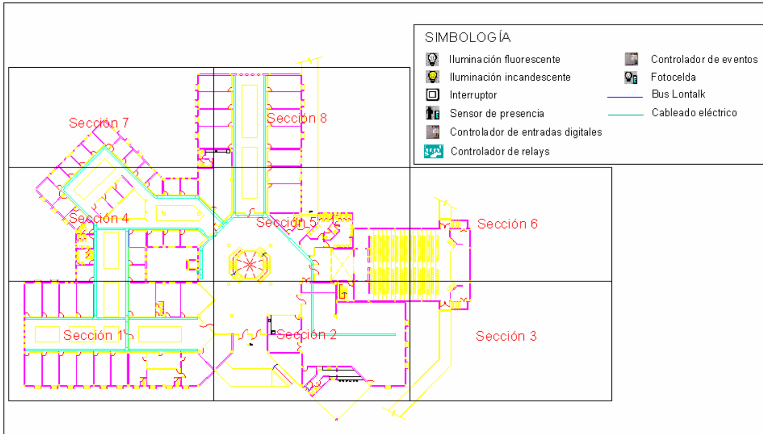
FIGURA 3.32 PLANO ILUMINACIÓN PLANTA BAJA GENERAL
