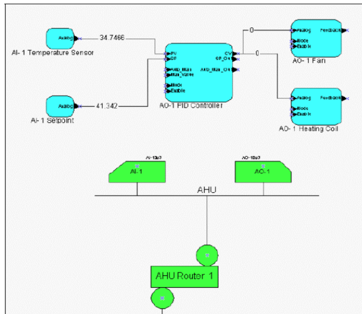
FIGURA 3.96 EJEMPLO DE DISEÑO DE RED CON HERRAMIENTA LONMAKER
