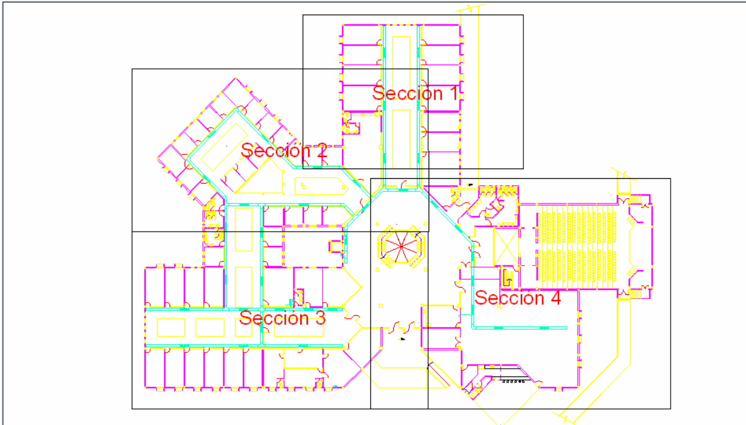
FIGURA 3.3 PLANO CLIMATIZACION PLANTA BAJA GENERAL
