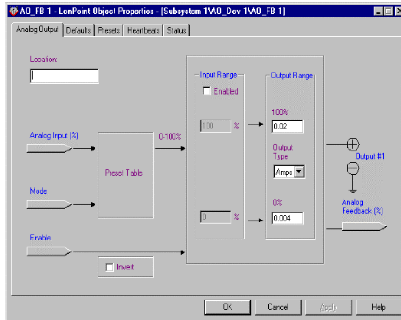
FIGURA 3.28 VENTANA PARA CONFIGURACION DE SALIDA ANALOGICA
