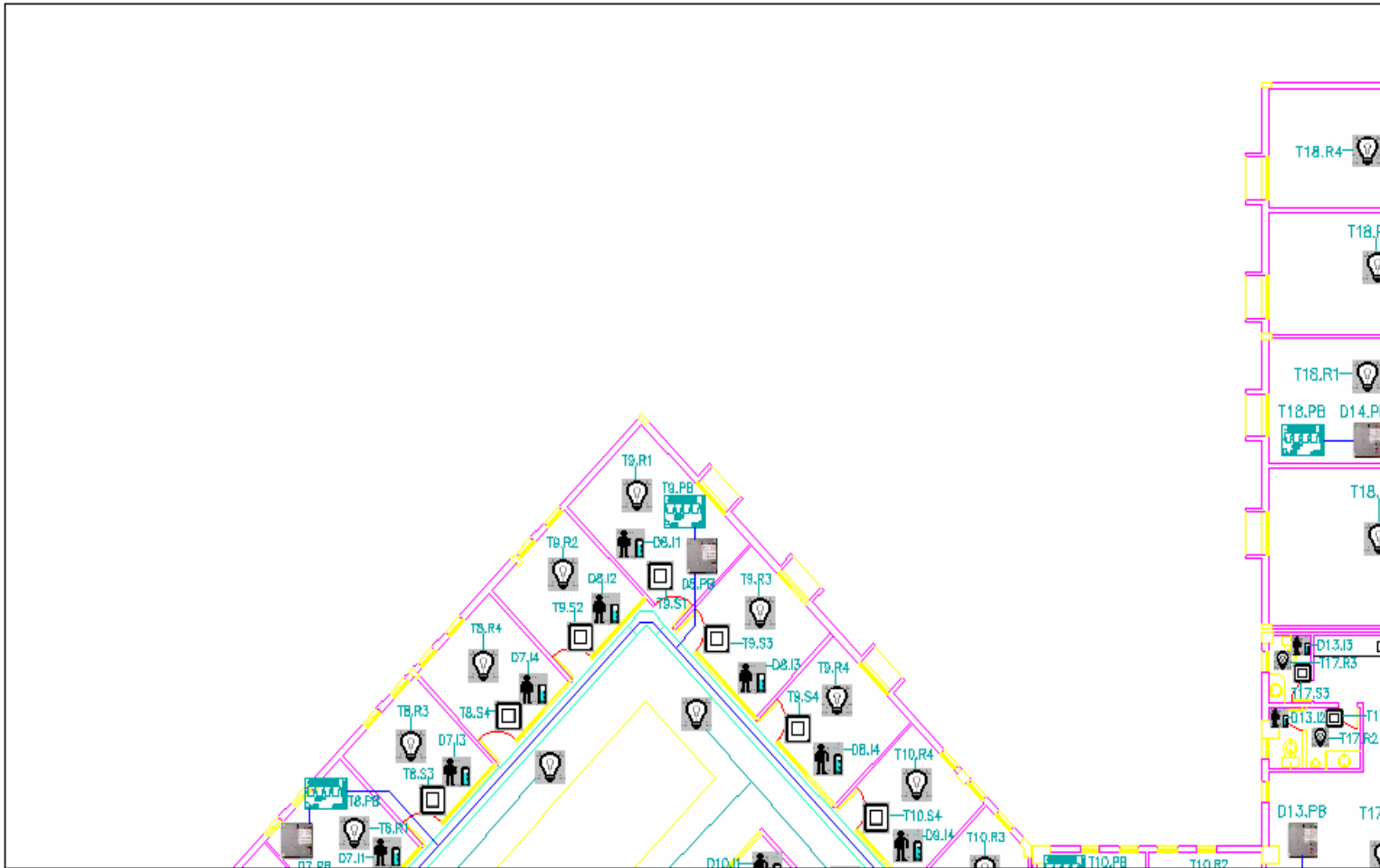
FIGURA 3.39 PLANO ILUMINACION PLANTA BAJA SECCION 7
