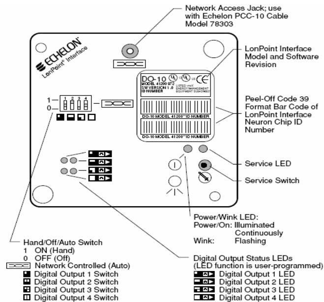
FIGURA 3.86 INTERFASE DE SALIDAS DIGITALES LONPOINT
