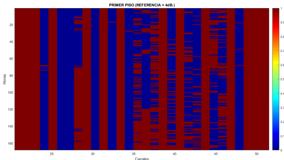
Figura 4.3 Disponibilidad de canales +4dB Planta baja
