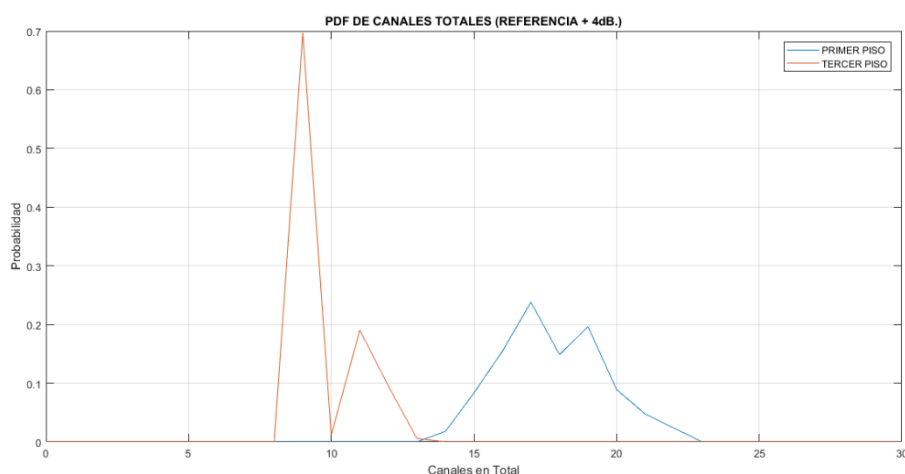
Figura 4.10 PDF Disponibilidad de canales +4dB
