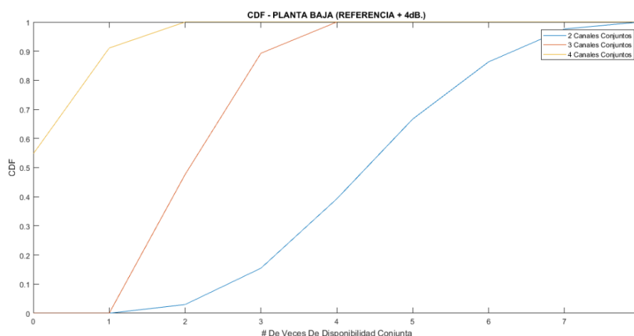
Figura 4.11 CDF Disponibilidad de canales conjuntos +4dB Planta baja
