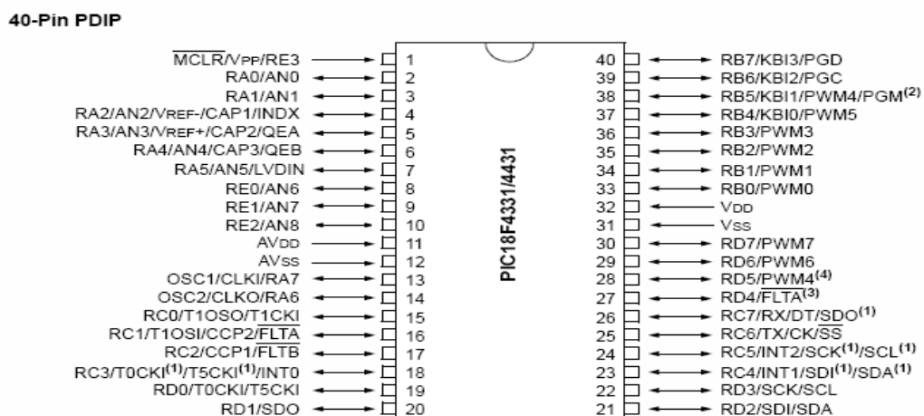
FIGURA 2-7: Diagrama de pines del PIC 18F4431
