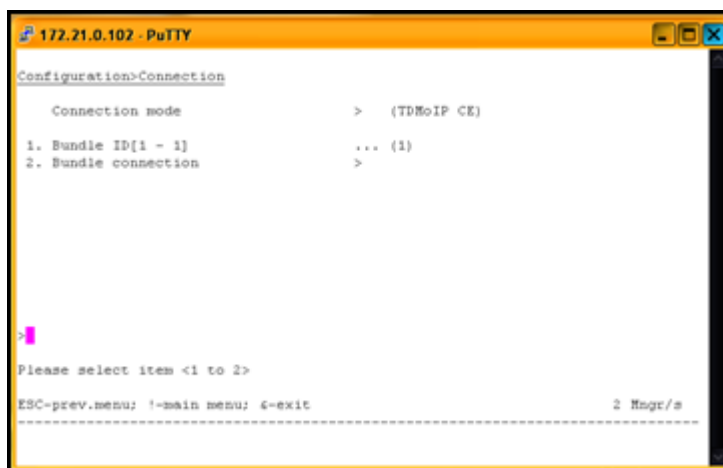
Figura 4. 43 Configuración de la Conexión, IPMUX-11.
