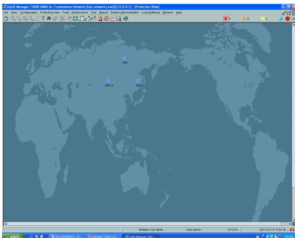
Figura 4. 19 Vista de protecciones SDH.
