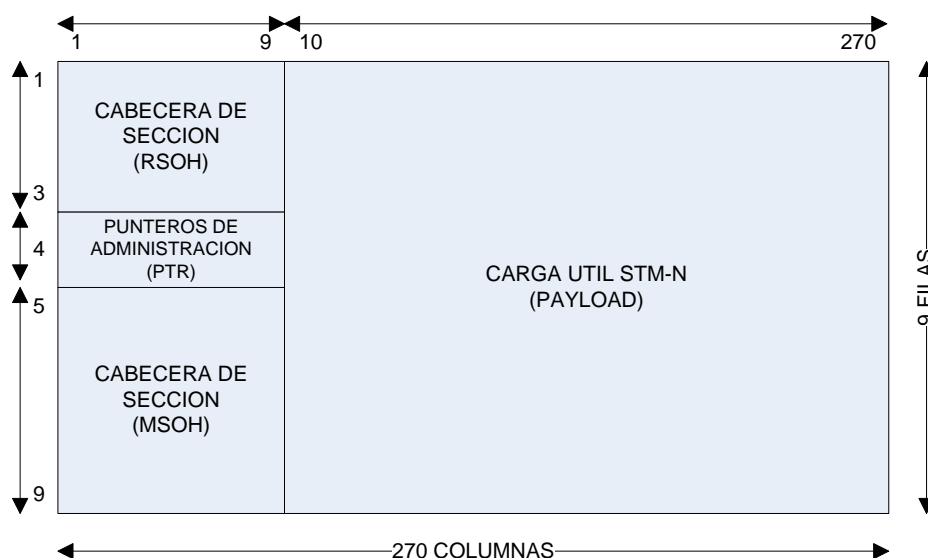
Figura 1. 7 Modulo de Transporte Síncrono (STM-N).
