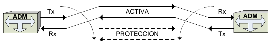
Figura 1. 16 Protección 1:1.
