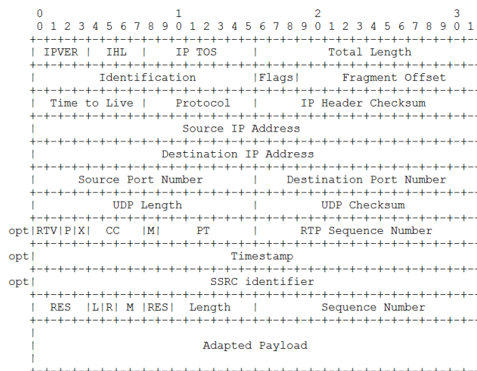
Figura 1. 24 Paquete TDMoIP con formato UDP/IP. [12]
