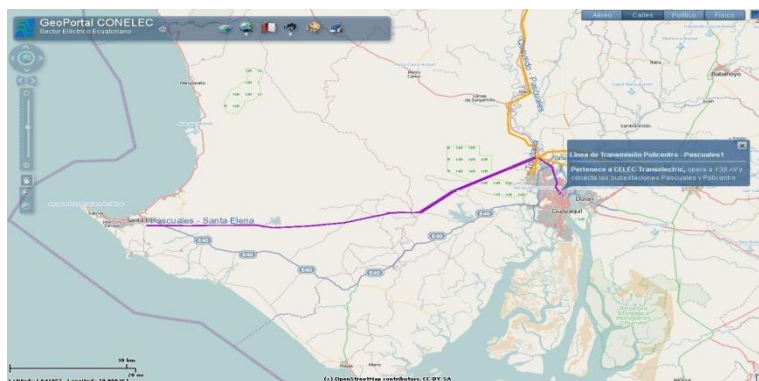
Figura 3. 7 Línea de Transmisión Energía Eléctrica Pascuales–Santa Elena. [25]
