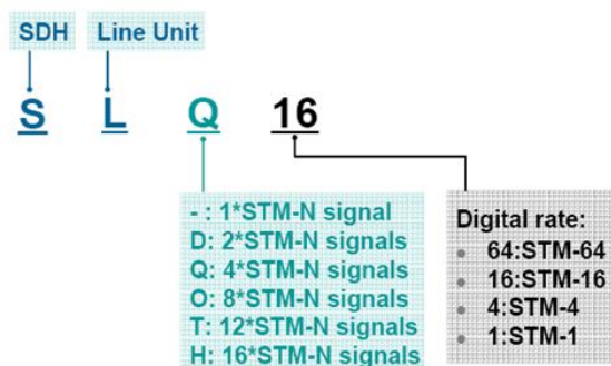
Figura 4. 3 Identificación de la tarjeta SLQ16.
