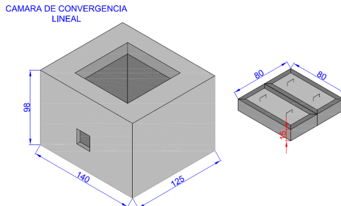
Figura 2. 7 Cámara telefónica homologada de hormigón armado.
