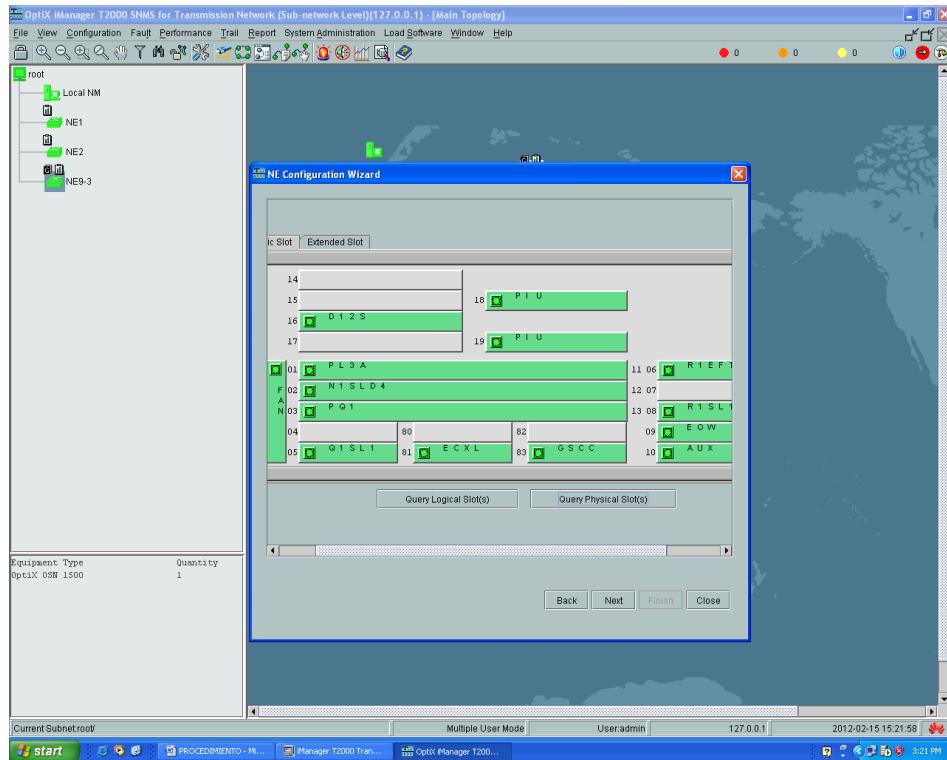
Figura 4. 16 Reconocimiento de las Tarjetas.
