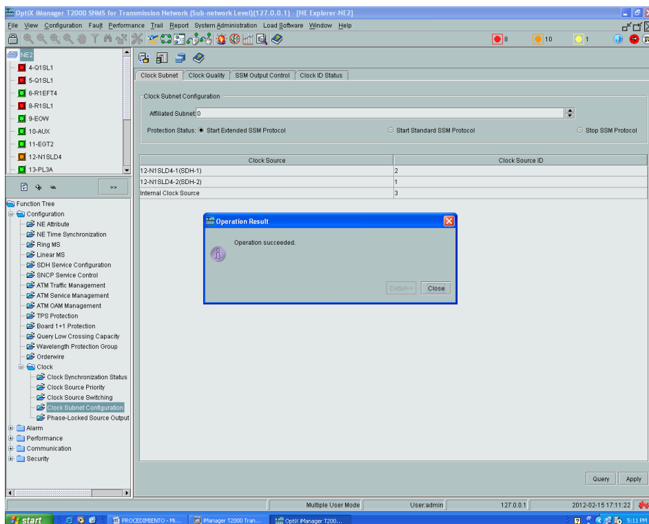
Figura 4. 29 Jerarquía de reloj NE2.
