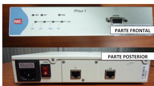
Figura 4. 5 Equipo IPmux-1.
