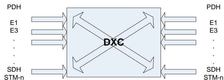
Figura 1. 11 de Cros-Conexión Digital.
