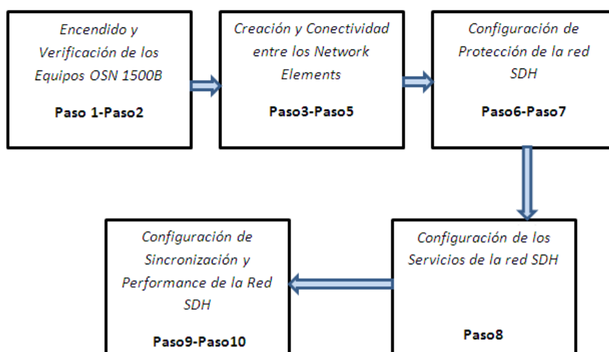
Figura 4. 7 Proceso de configuración del OSN 1500B.
