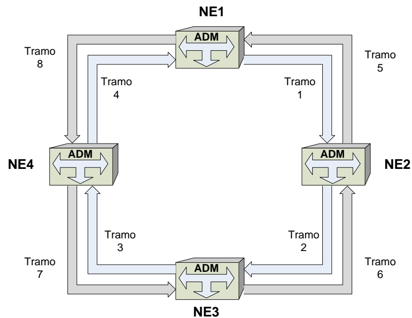
Figura 1. 18 Arquitectura de Protección Tipo Anillo 2 Fibra.
