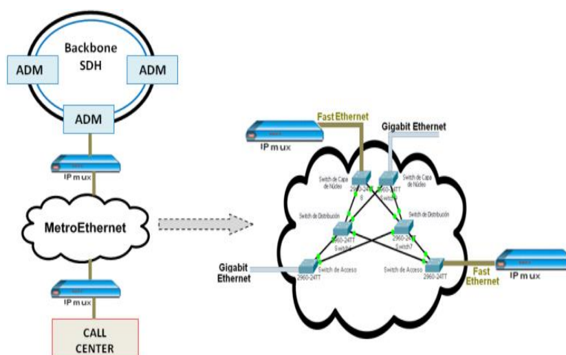
Figura 4. 6 TDMoIP usando MetroEthernet.
