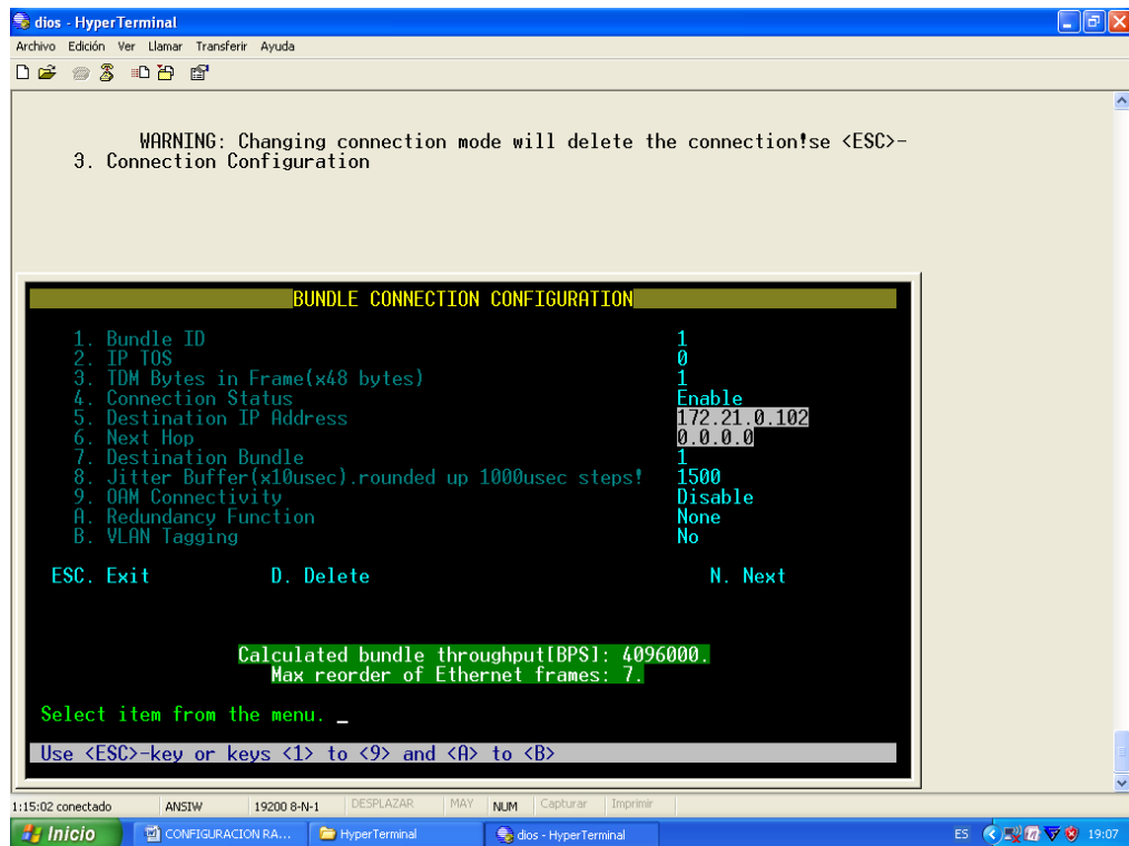
Figura 4. 37 Configuración de Conexión del Bundle, IPMUX-1.
