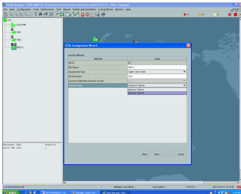
Figura 4. 15 Elección del tipo de Sub-rack.
