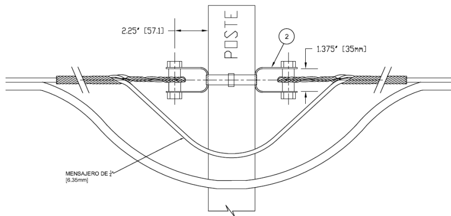
Figura 2. 1 Herraje de retención Tipo A.
