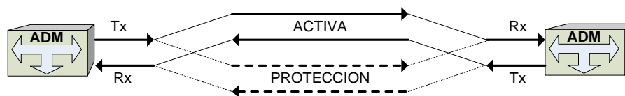
Figura 1. 15 Protección 1+1.
