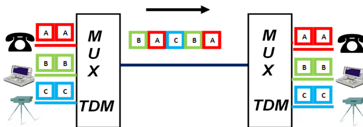
Figura 1. 22 Multiplexación por división de tiempo.
