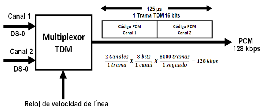
Figura 1. 23 Sistema PCM-TDM de 2 canales.
