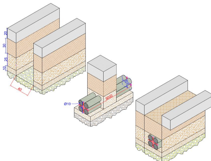
Figura 2. 3 Canalización de ductos PEAD, en zona urbana.
