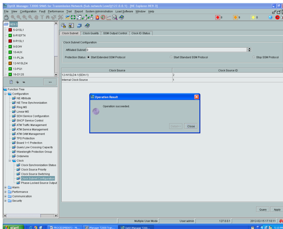
Figura 4. 28 Jerarquía de reloj NE3.
