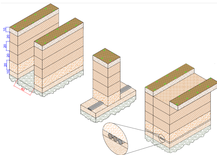
Figura 2. 4 Canalización de triductos, en zona rural.
