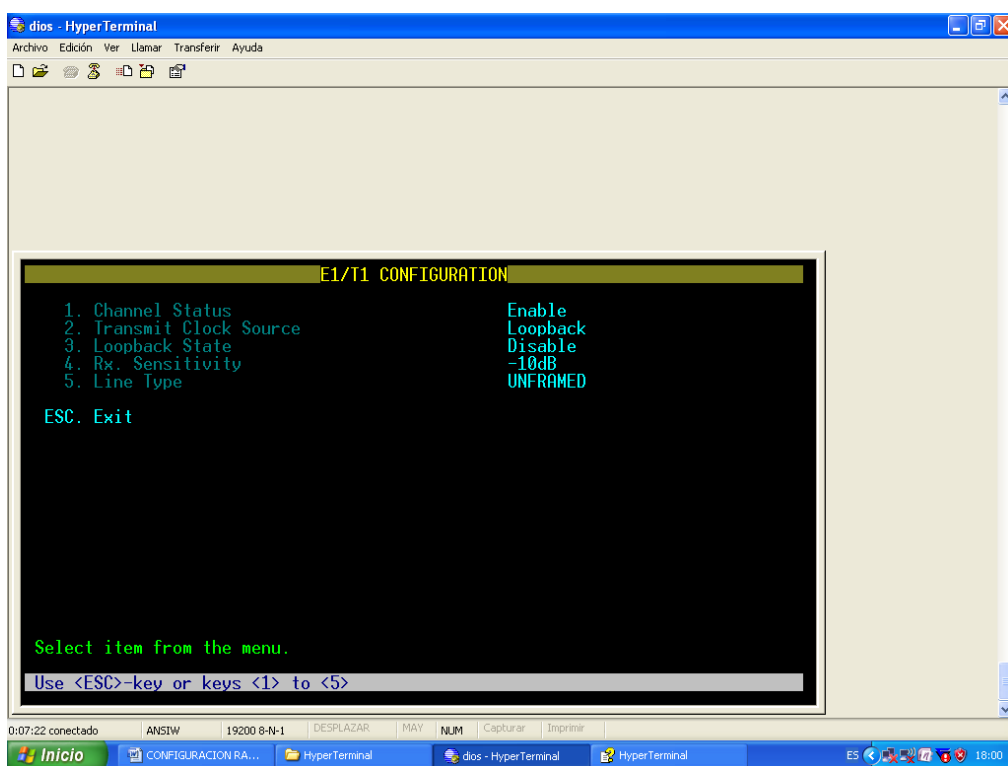
Figura 4. 35 Configuración del E1/T1, IPMUX-1.
