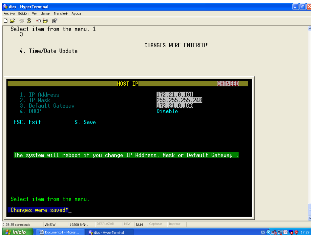
Figura 4. 34 Direccionamiento IP, IPMUX-1.
