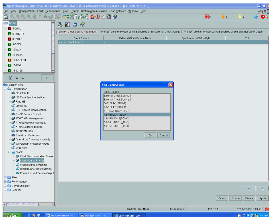
Figura 4. 27 Configuración del Clock.
