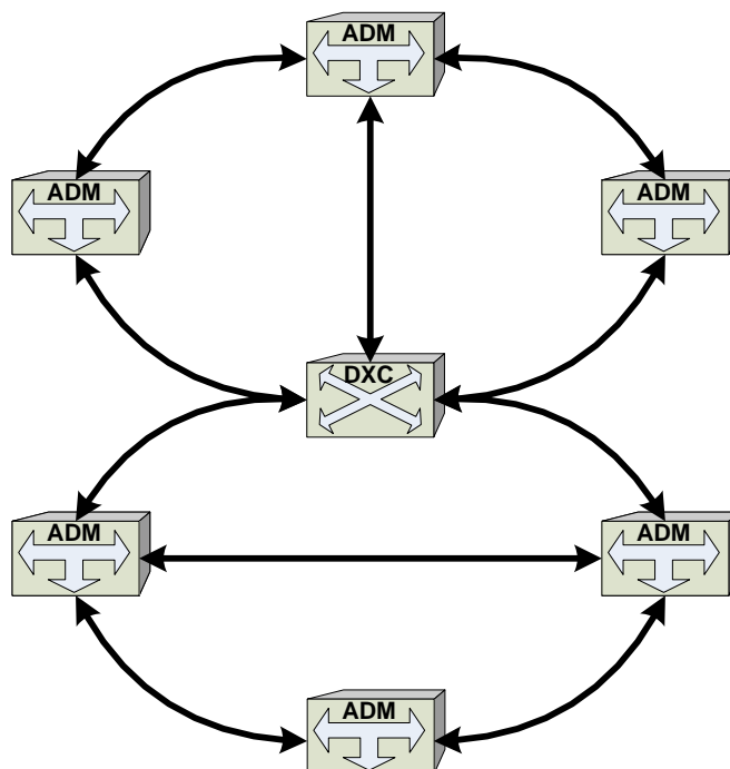
Figura 1. 14 Topología anillo full-mesh.
