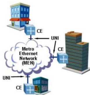
Figura 1. 30 Modelo de referencia de redes MEN. [14]
