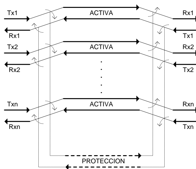
Figura 1. 17 Protección N:1.
