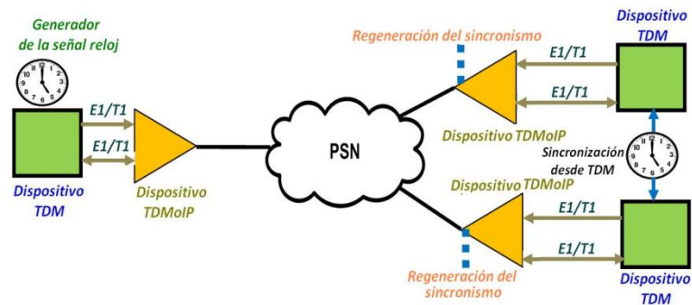
Figura 1. 28 Sincronización por recuperación de reloj adaptante.
