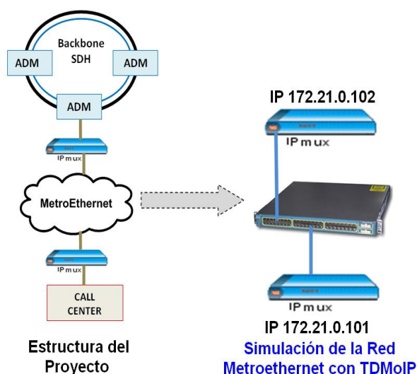
Figura 4. 31 Simulación de la red Metro Ethernet.
