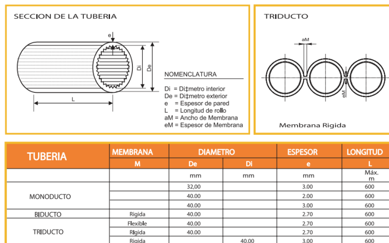
Figura 2. 6 Triducto para canalización eléctrica y de telecomunicaciones. [19]
