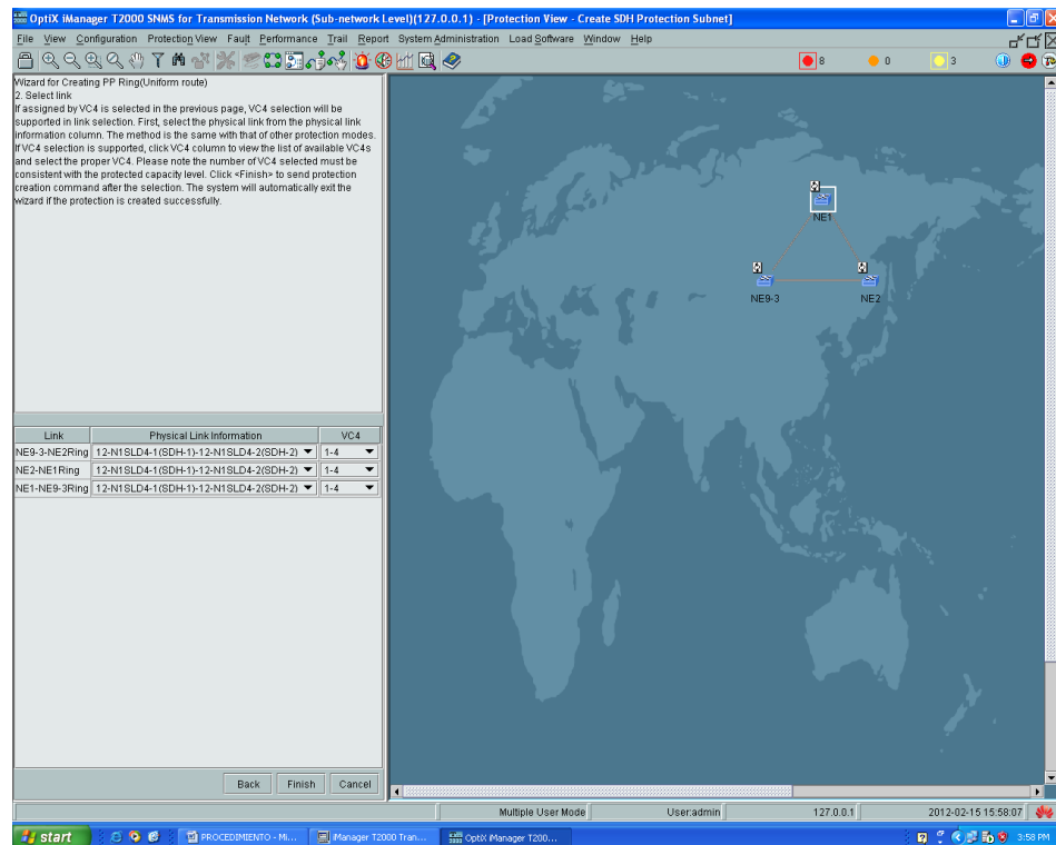
Figura 4. 20 Atributos de protección de camino.
