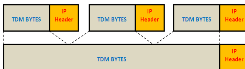
Figura 1. 26 Agrupación de tramas TDM en paquetes TDMoIP.
