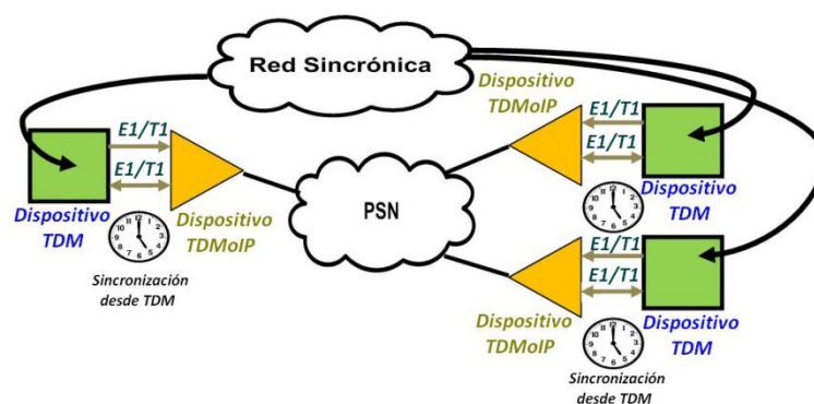
Figura 1. 27 Sincronización por reloj externo en ambos extremos.
