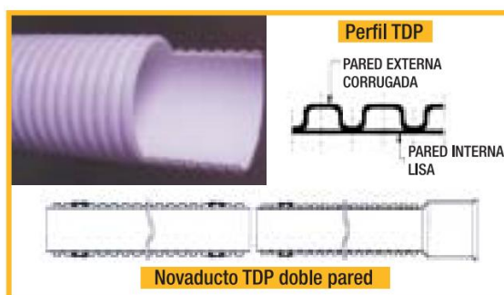
Figura 2. 5 Ducto para canalización eléctrica y de telecomunicaciones. [18]
