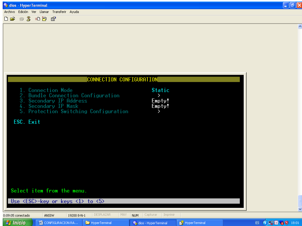
Figura 4. 36 Configuración de la Conexión, IPMUX-1.
