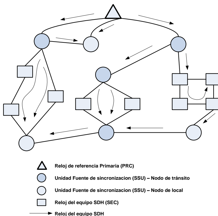
Figura 1. 20 Jerarquía de sincronización de relojes.
