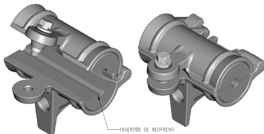
Figura 2. 2 Herraje de sucesión Tipo B.
