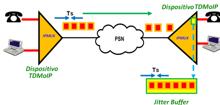
Figura 1. 29 Sincronización y reordenamiento de paquetes.
