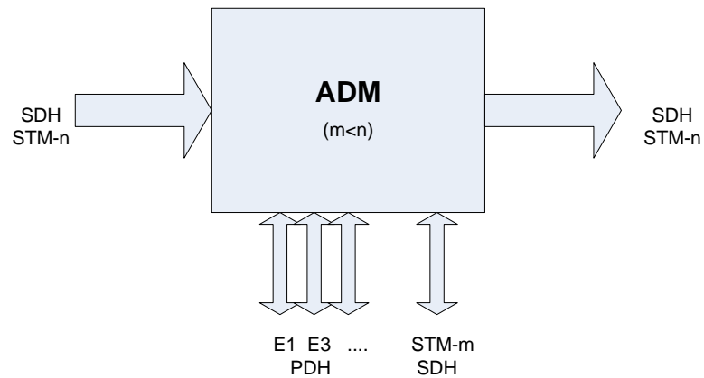
Figura 1. 10 Multiplexor de Extracción y Adición.
