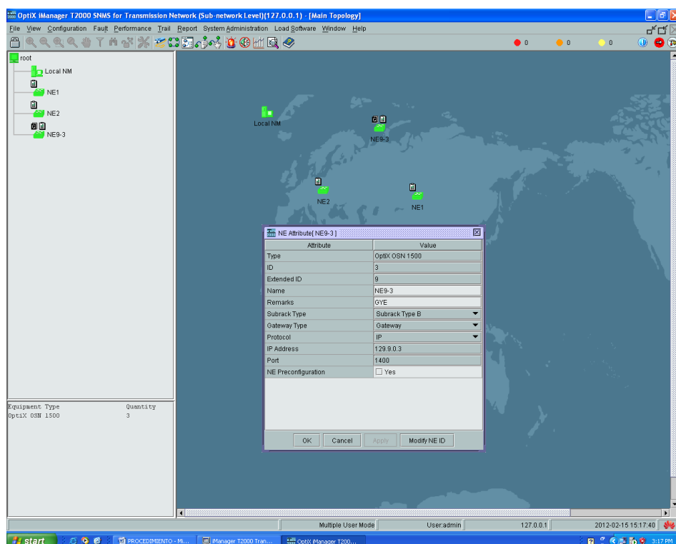
Figura 4. 13 NE como Gateway.
