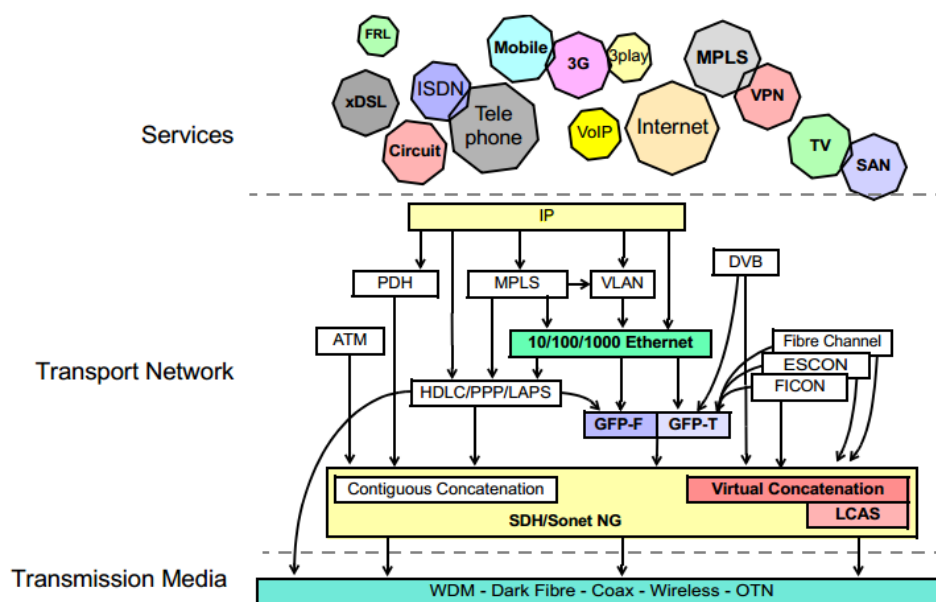
Figura 1. 21 Integración de servicios MSTP. [8]
