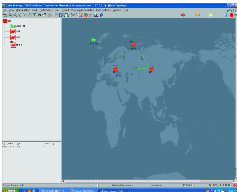
Figura 4. 18 SDH SNC-GYE-UIO.
