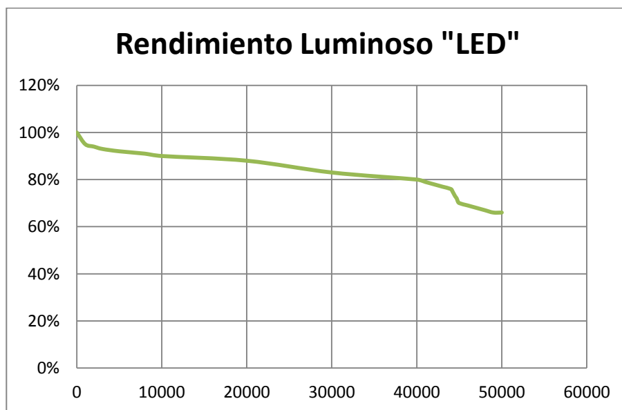
Figura 4.16 Rendimiento luminoso de foco LED
