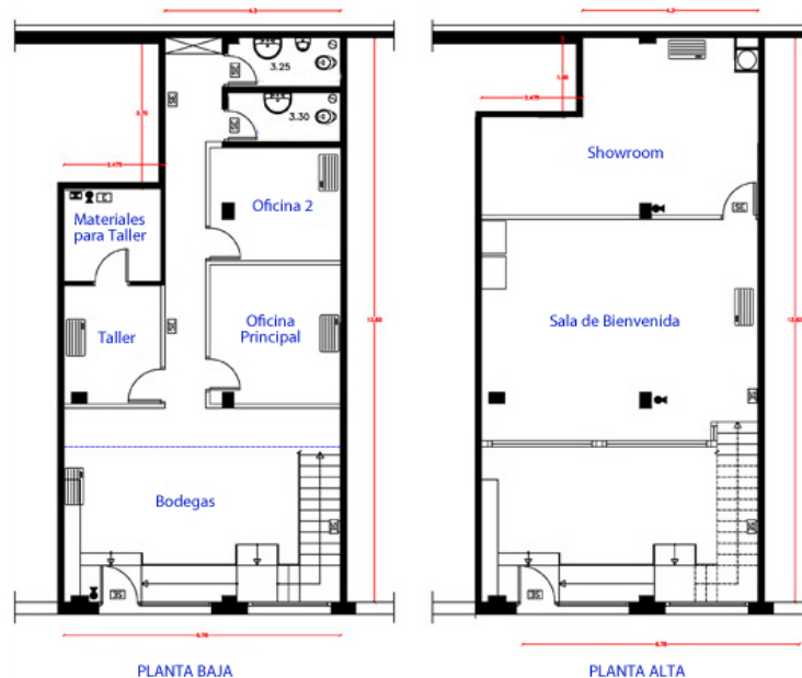
Gráfico 1-8 Plano Arquitectónico de la oficina en Quito.
