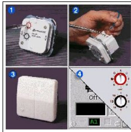
Figura 2.2.2.4 - Procedimiento de instalación de un modulo de empotrar
