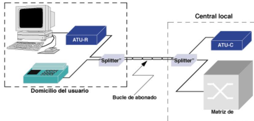
Figura 3.8: Conexión ADSL
