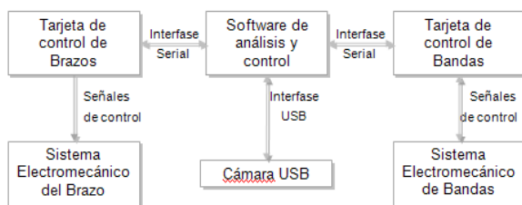
Figura 2. Diagrama de Control del Sistema
