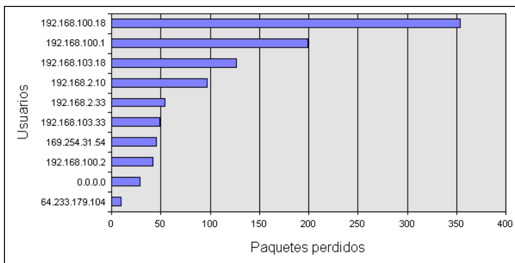
Figura 3.36 Diagrama de barras de los paquetes perdidos por usuario de la LAN después de la auditoría.
