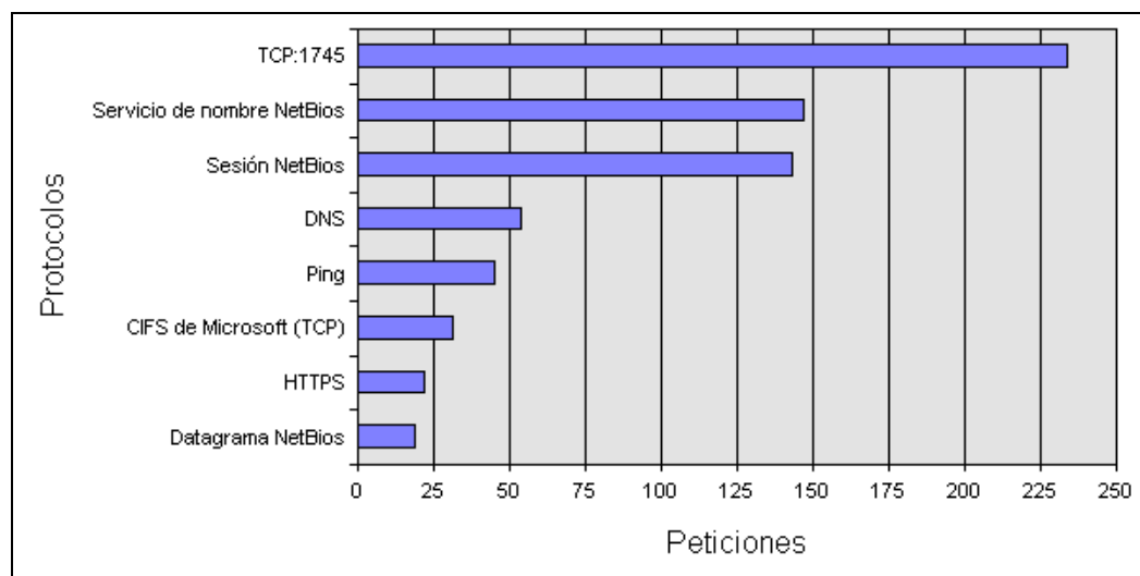
Figura 3.33 Diagrama de barras del tráfico por protocolos de aplicación después de la auditoria.
