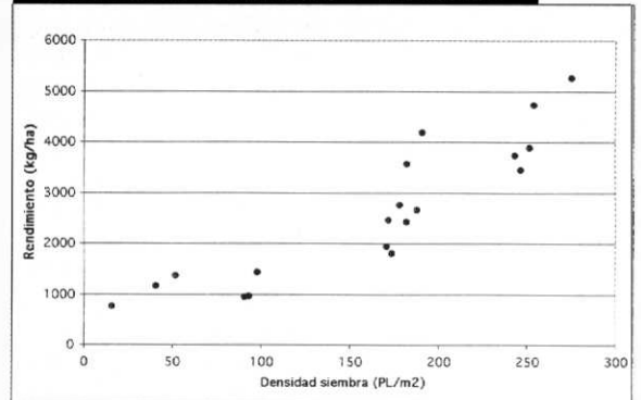
FIGURA 2: RELACION RENDIMIENTO – DENSIDAD DE SIEMBRA EN PRECRÍA BAJO INVERNADEROS
