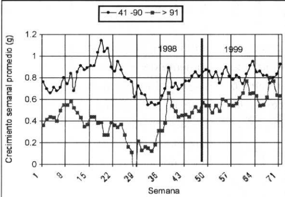
FIGURA 10: MEDIA CORRIDA MENSUAL DEL CRECIMIENTO SEMANAL DE LAS CUATRO ÚLTIMAS SEMANAS EN ESTANQUES CON PERIODOS DE CULTIVO ENTRE 41-90 DÍAS Y MÁS DE 91 DÍAS.
