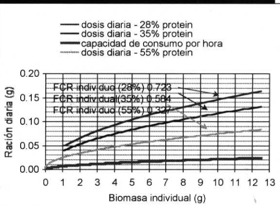
FIGURA 13: REQUERIMIENTO DE ALIMENTO BALANCEADO PARA DIETAS DE 28%, 35% Y 55% DE PROTEINA, EN FUNCION DE LA BIOMASA INDIVIDUAL.
