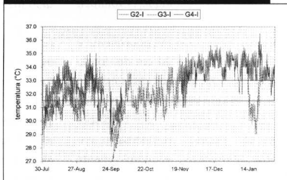
FIGURA 7: TEMPERATURA DEL AGUA EN TRES INVERNADEROS (0.23 HA, 0.26 HA Y 0.33 HA) ENTRE AGOSTO DEL 2002 Y FEBRERO DEL 2003.
