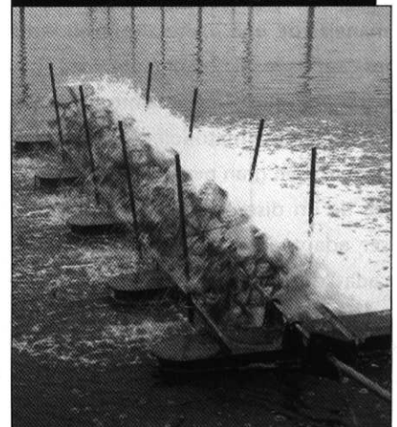
FIGURA 9: AIREADOR DE PALETA IMPULSADO POR UN MOTOR DIESEL DE 8HP.
