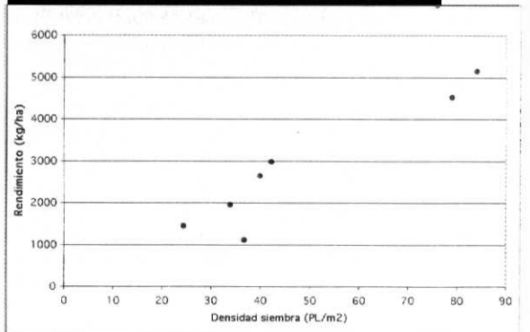
FIGURA 4: RELACION RENDIMIENTO – DENSIDAD DE SIEMBRA EN ENGORDE BAJO INVERNADEROS
