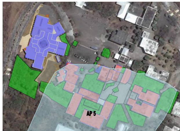
Figura 5-77 Cobertura real del AP5
