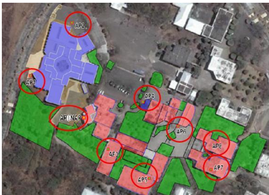
Figura 4-20 Ubicación de los nuevos puntos de acceso en la FIEC
