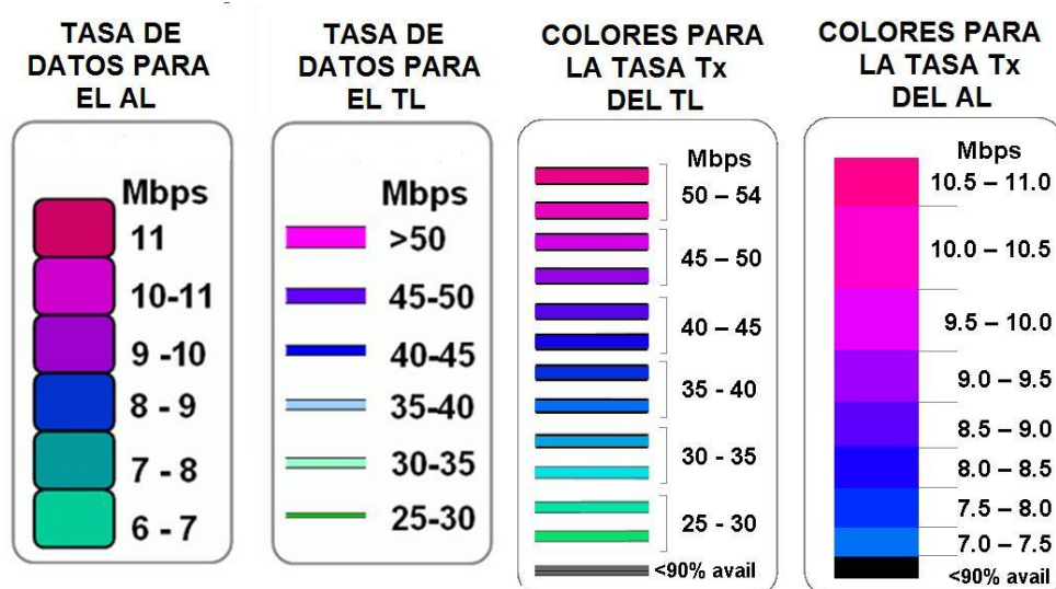
Figura 4-29 Indicadores de Cobertura
