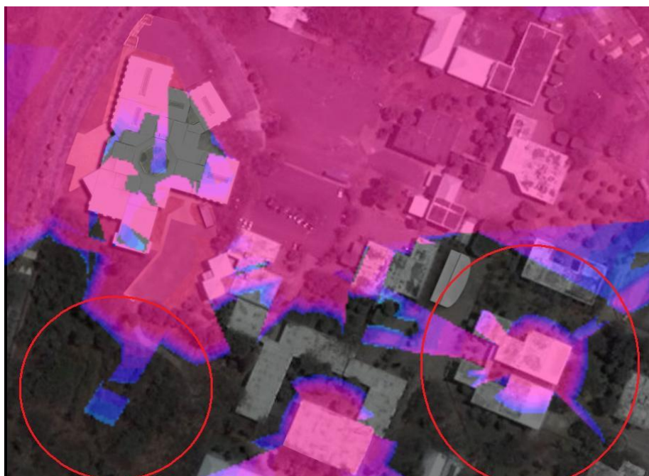
Figura 4-33 Detección de Zonas Muertas en el Diseño Teórico
