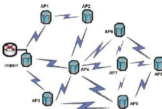
Figura 4-24 Topología de Red basados en resultados simulados en el Planner
