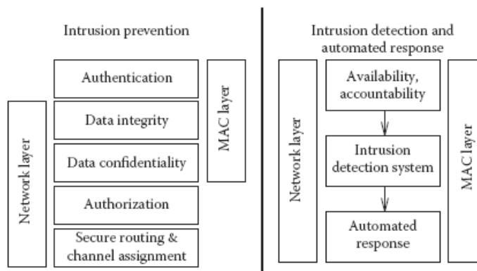
Figura 2-23 Prevención y detección de intrusos
