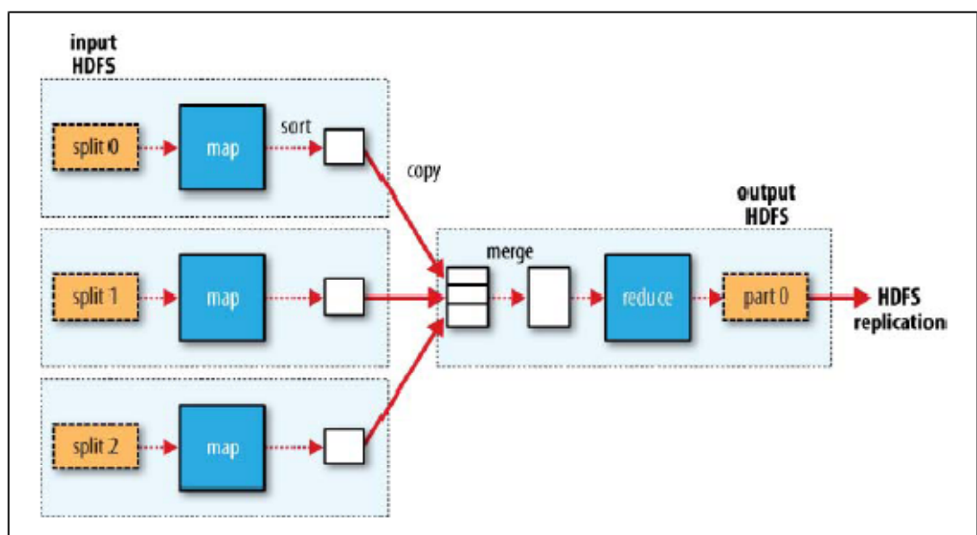
FIGURA 5.1. PROCESO MAP-REDUCE [22].
