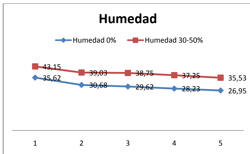
Figura 3.5. Pérdida de Humedad en el Almacenamiento
