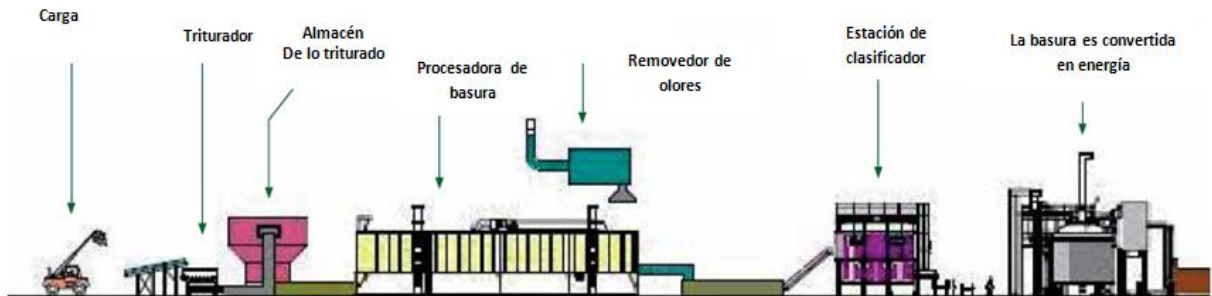
Fig. 5 (Esquema del proceso)
