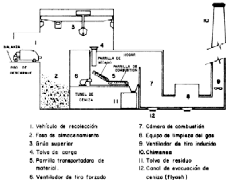
Fig. 9 (Sección transversal de un incinerador municipal de alimentación continua y encendido total.)
