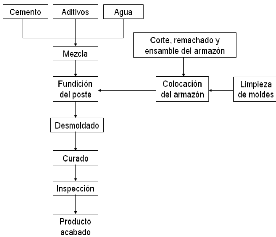
FIGURA 2.6 ORGANIGRAMA GENERAL DEL PROCESO
