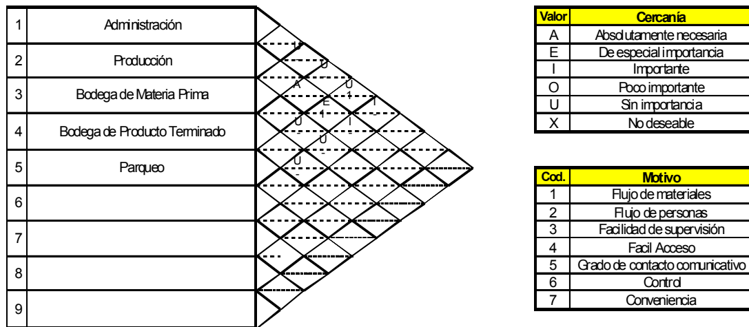
Figura 4.8 Diagrama de Relaciones
