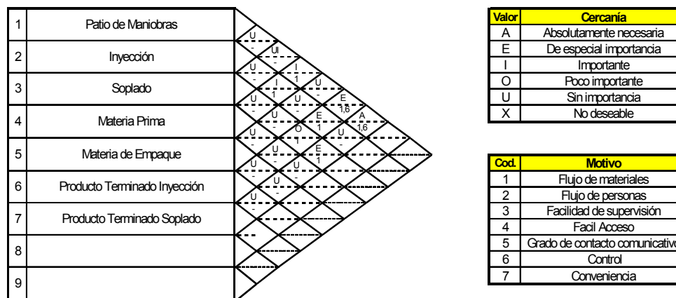
Figura 3.2 Diagrama de Relaciones de la Planta de Plásticos.
