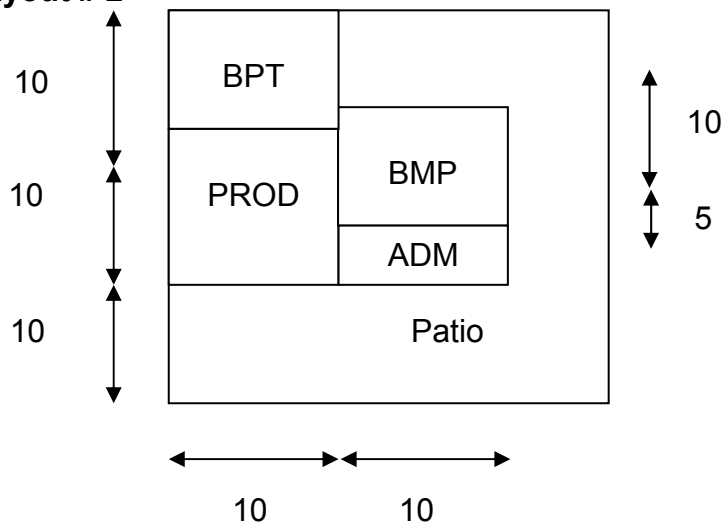
Figura 4.15 Alternativa de Distribución Física # 2
