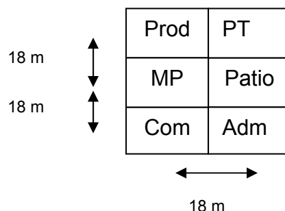
Figura 3.16 Distribución física final de la Planta de Puré de Banano.
