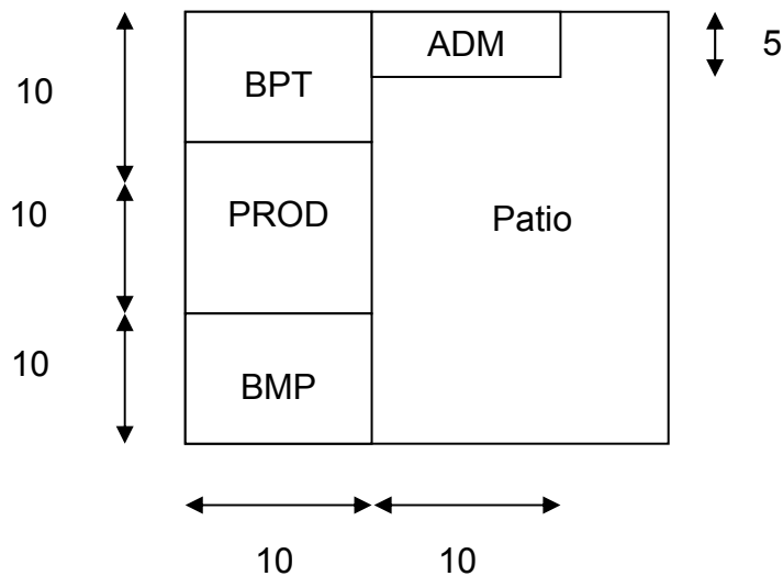
Figura 4.10 Alternativa de Distribución # 1
