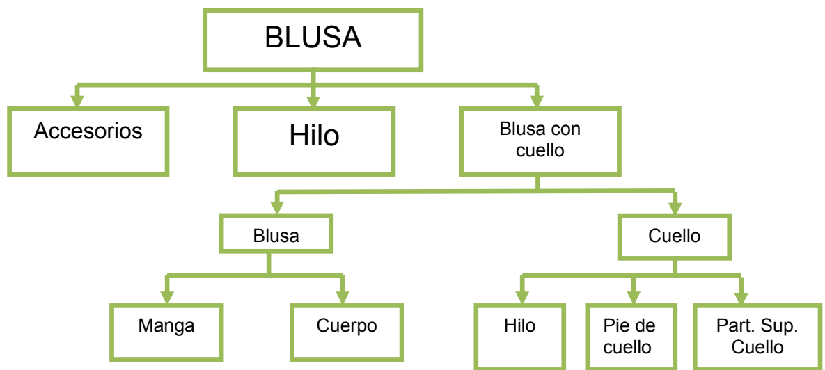
Figura 2.7 Diagrama Bill Of Materials de Blusas.
