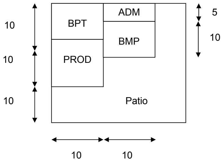
Figura 4.14 Alternativa de Distribución Física # 1.
