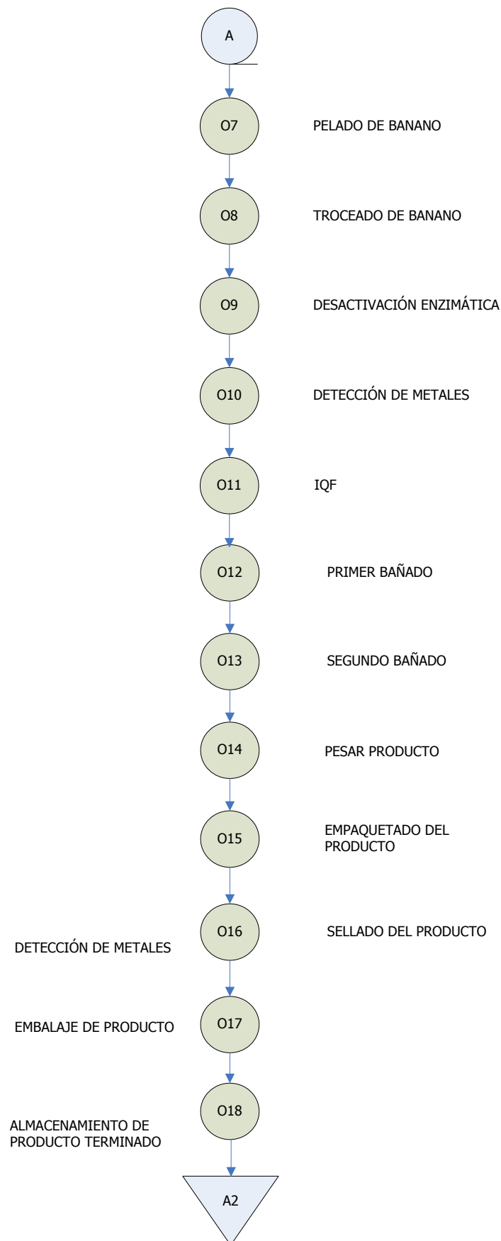
Figura 4.17 Proceso de Producción
