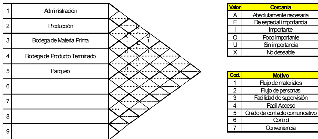
Figura 4.13 Diagrama de Relaciones.
