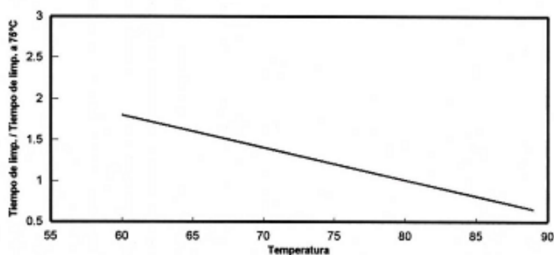
Fig. 3.6 Efecto de la temperatura sobre el tiempo de limpieza utilizando un detergente Single Stage.
