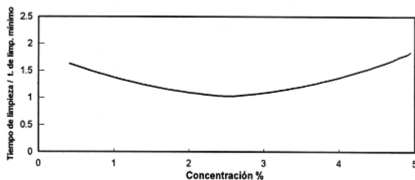
Fig. 3.5 Efecto de limpieza vs. la concentración del detergente Single Stage.
