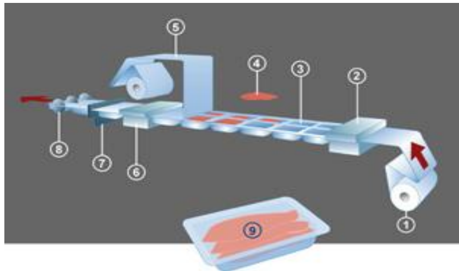
FIGURA 4.1 DIAGRAMA DE FUNCIONAMIENTO DE LA TERMOFORMADORA MULTIVAC.
