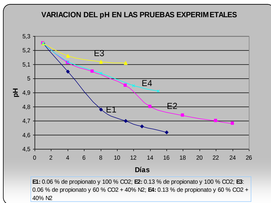
FIGURA 3.10. VARIACION DEL pH PARA LAS PRUEBAS EXPERIMENTALES.
