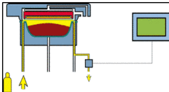
FIGURA 4.4. MONITORIZADO DE ATMÓSFERA EN EQUIPOS DE LAS SERIES EN LÍNEA.
