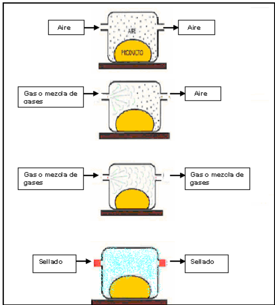
FIGURA 2.2. ESQUEMA DE DESPLAZAMIENTO DEL AIRE POR LA NUEVA ATMÓSFERA
