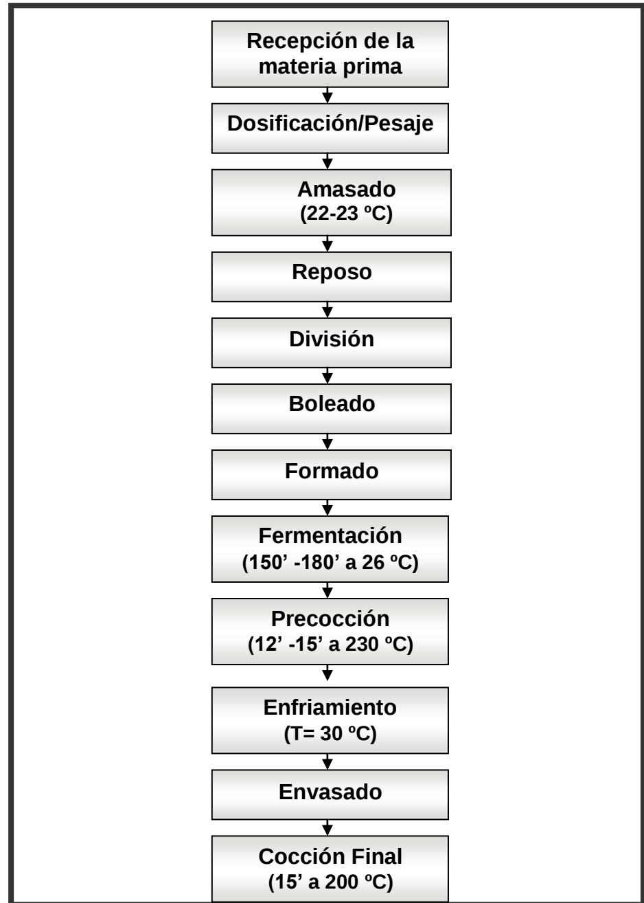
FIGURA 1.1 DIAGRAMA DE FLUJO DEL PROCESO DE ELABORACION DE PAN PRECOCIDO
