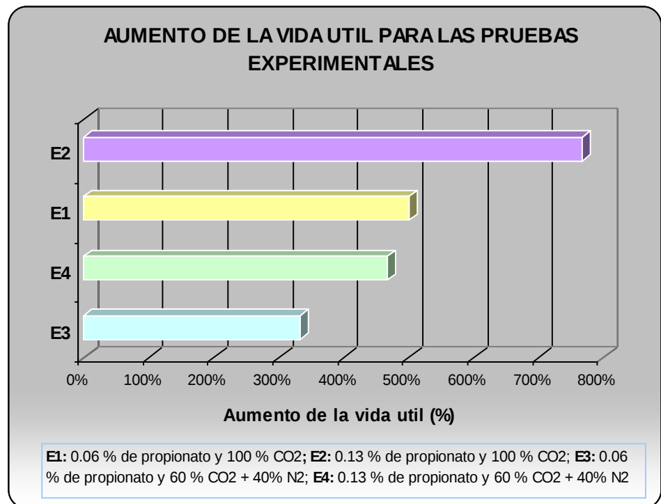
FIGURA 3.6. AUMENTO DEL TIEMPO DE VIDA UTIL DE LAS PRUEBAS EXPERIMENTALES SIN CRECIMIENTO DE MOHOS Y LEVADURAS.
