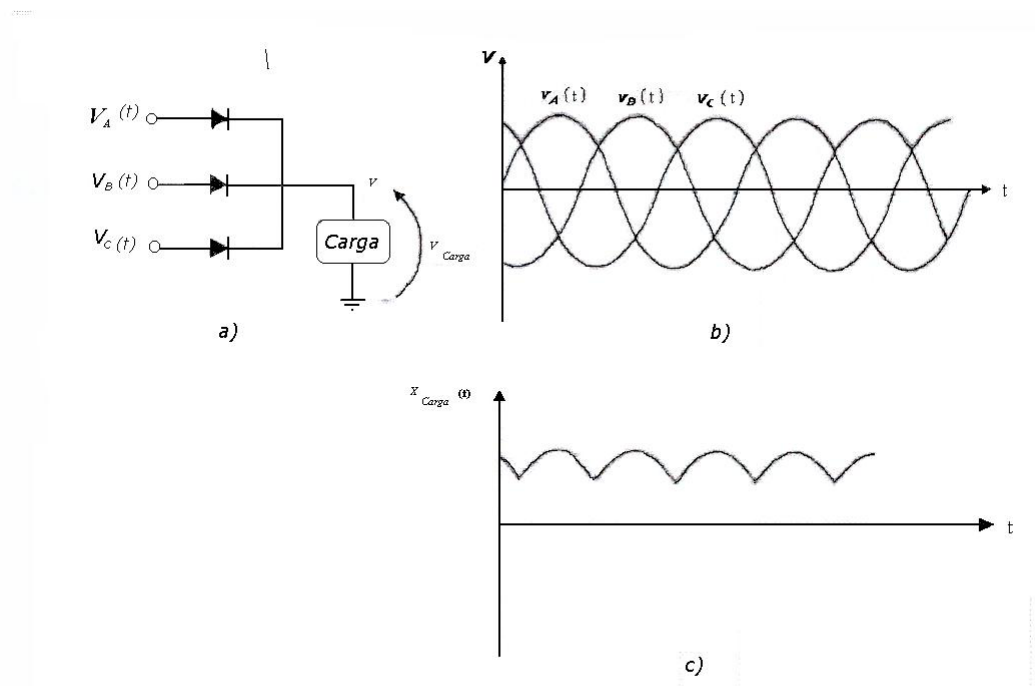
Figura 2.4: Regulación de carga:
