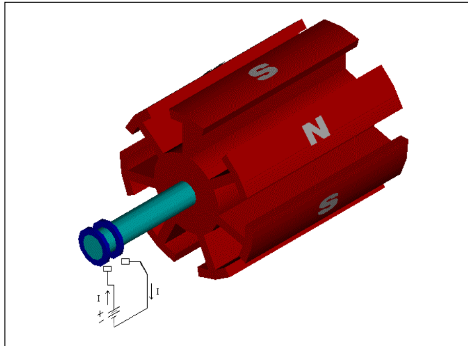
Figura 2.7: Generador Trifásico con electroimán.
