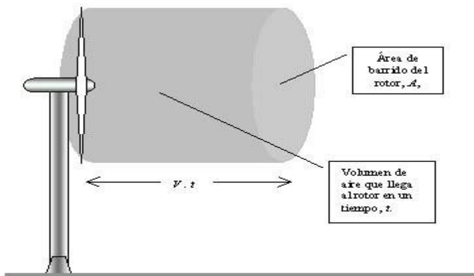
Figura 1.8: Volúmen de aire que llega al rotor
