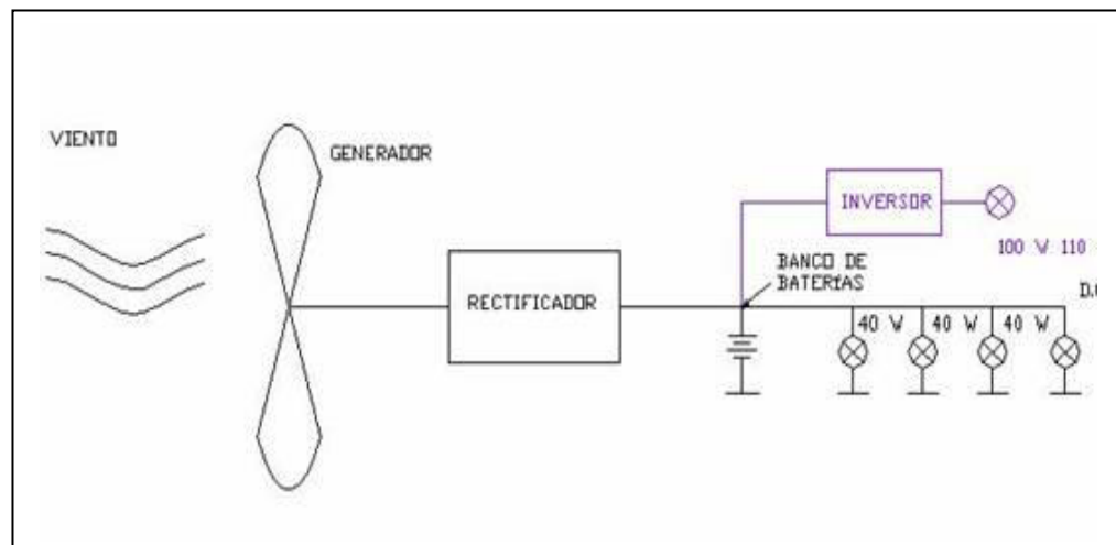
Figura 2.8: Esquema del generador ubicado en el CENAE.
