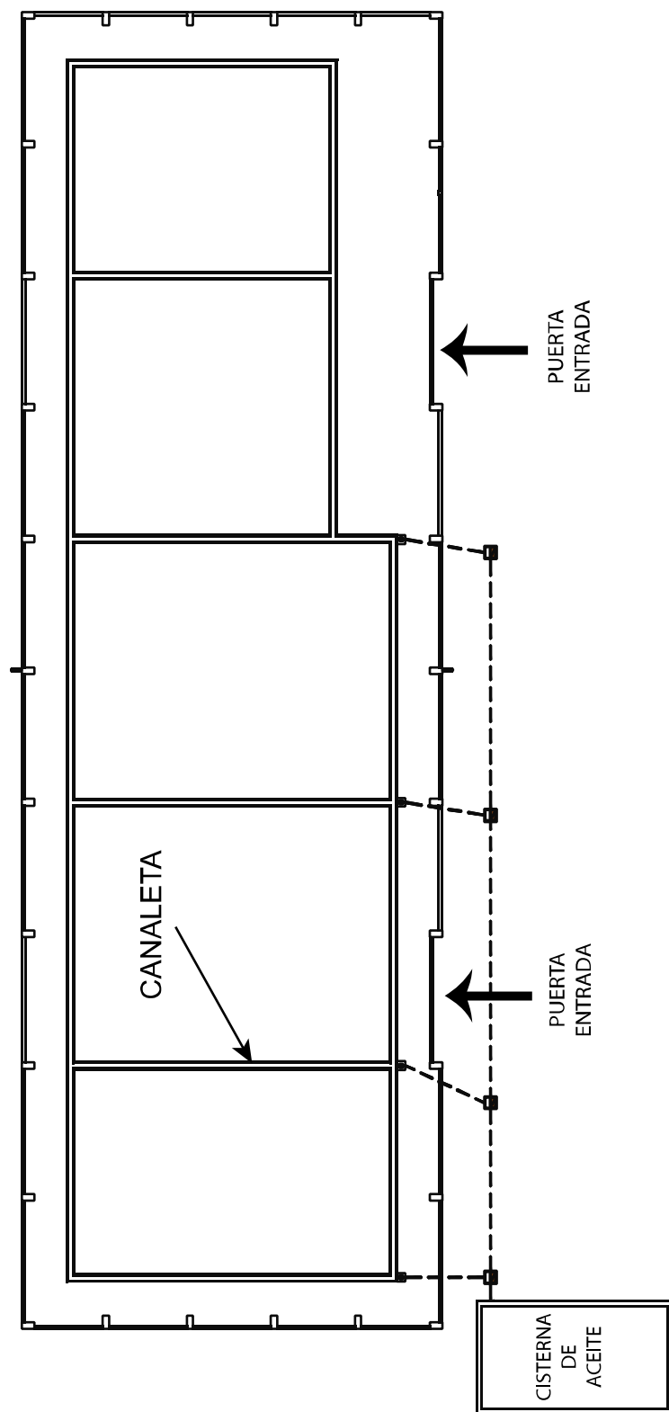
FIGURA 4.3 MODELO DE PLANO DE BODEGA DE ALMACENAMIENTO DE PCB's
