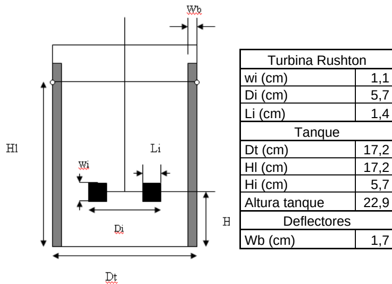
Figura 2.3. Dimensiones del quimiostato piloto (Elaborado por: Gandhi Armas Andrade)
