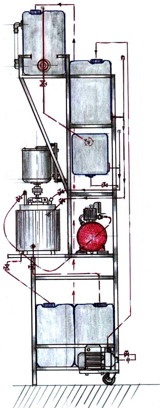
Figura 3.3. Quimiostrato. Vista lateral derecha. (Elaborado por: Gandhi Armas Andrade)
