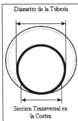
FIGURA 2.4 ÁREA DE LA TUBERÍA ENTERRADA EN LA COSTRA DE LODO
