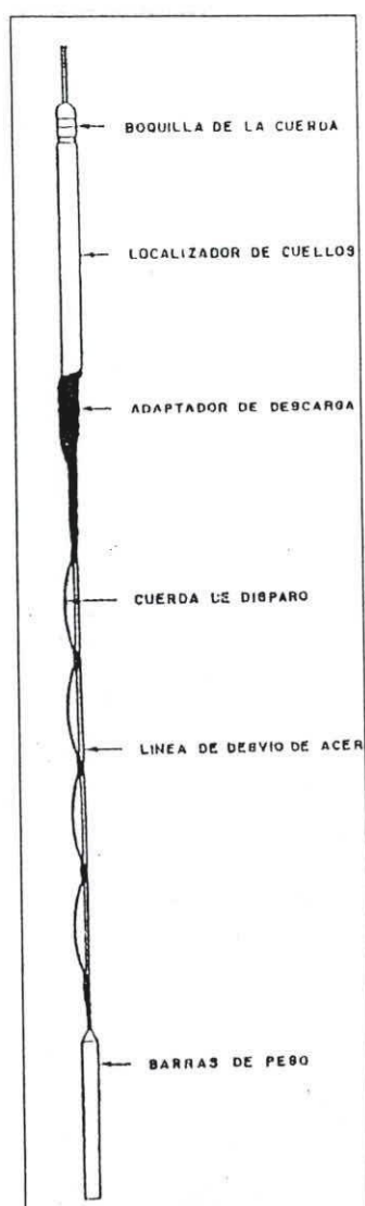
FIGURA 3.6 CUERDA DE TIRO DE DESENROSQUE
