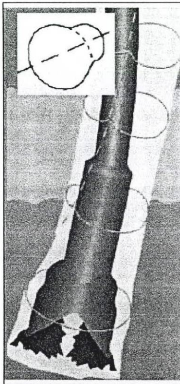
FIGURA 2.11 AGUJERO NO VERTICAL
