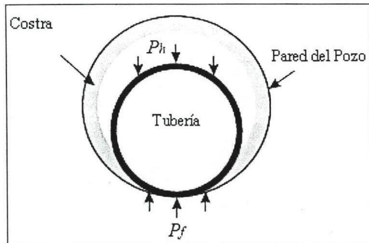
FIGURA 2.2 PEGA DIFERENCIAL.
