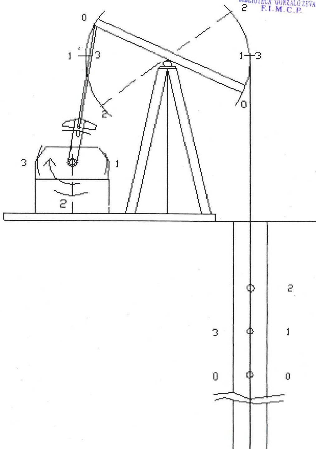
FIGURA 1.6 POSICIONES DEL BALANCÍN EN BOMBEO MECÁNICO.
