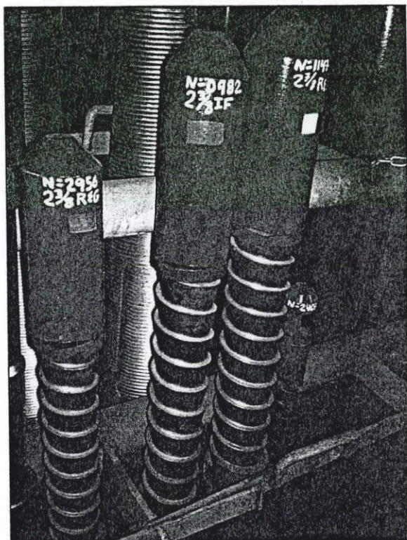
FIGURA 3.11B PESCANTE ARPÓN RECUPERABLE, COMPAÑÍA WEATHERFORD
