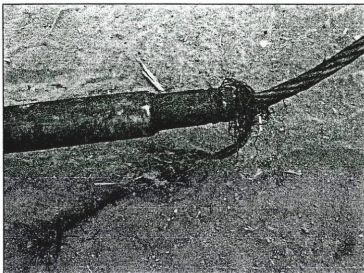
FIGURA 2.12 RUPTURA EN LA UNIÓN CABLE-HERRAMIENTA LOCAL
