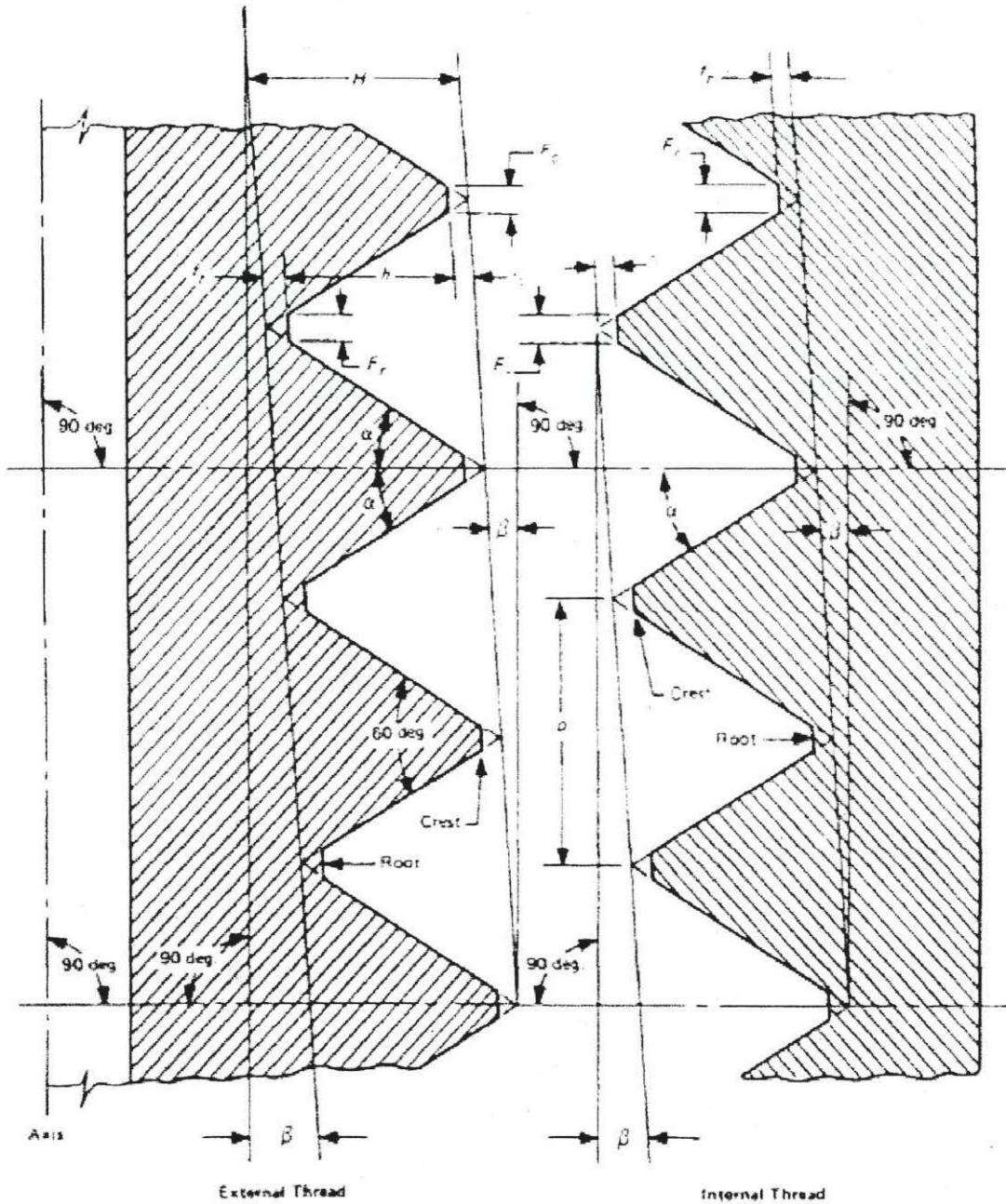
Forma Básica de una Rosca NPT (Norma ASME B1.20.1)
