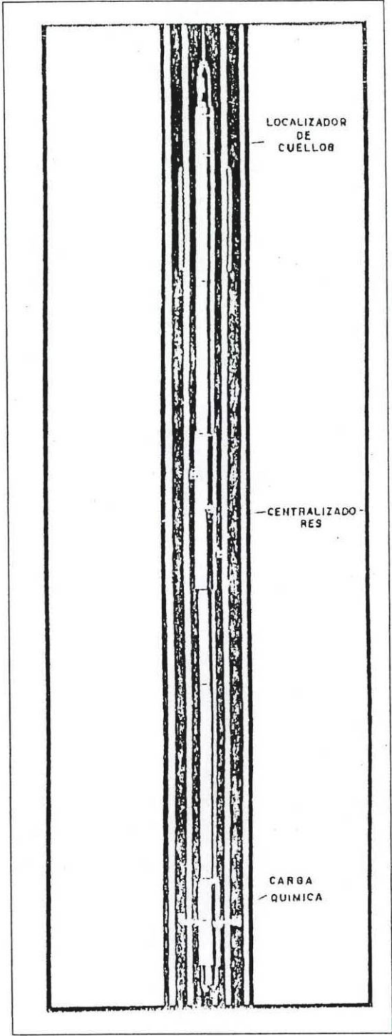
FIGURA 3.9A. CORTADOR QUÍMICO DE TUBERÍA
