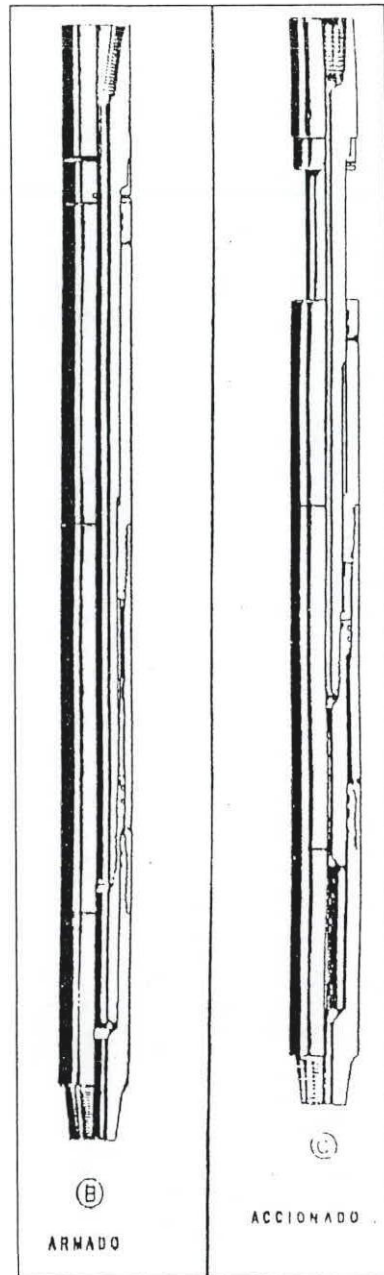
FIGURA 3.15 MARTILLO HIDRÁULICO
