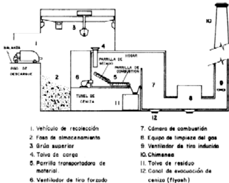
Fig. 9 (Sección transversal de un incinerador municipal de alimentación continua y encendido total.)
