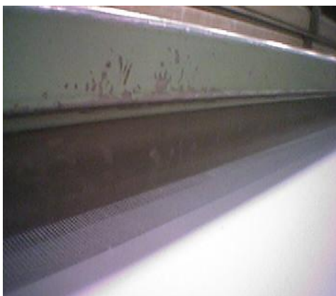
FIGURA 3.28. Batán con Peine.
