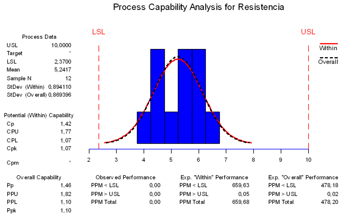
FIGURA 6.2 ANÁLISIS DE CAPACIDAD RESISTENCIA
