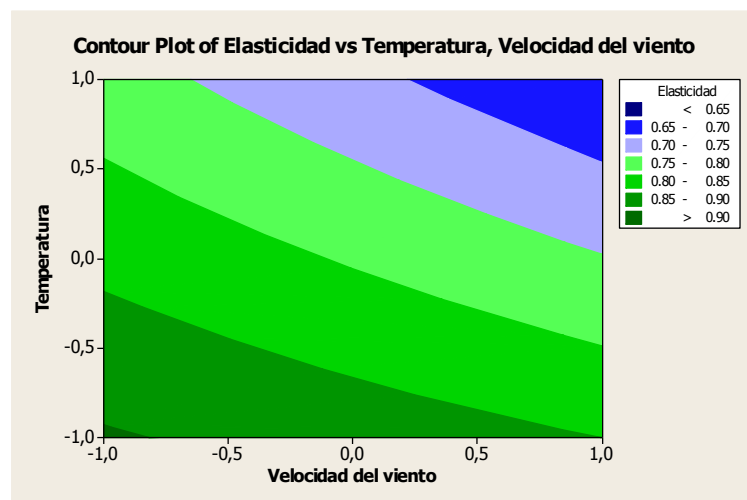
FIGURA 5.9 CONTORNO ELASTICIDAD
