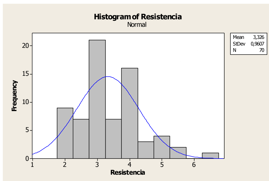
FIGURA 4.4 HISTOGRAMA RESISTENCIA (APÉNDICE 4)
