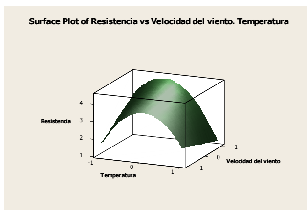
FIGURA 5.17 SUPERFICIE DE REPUESTA RESISTENCIA
