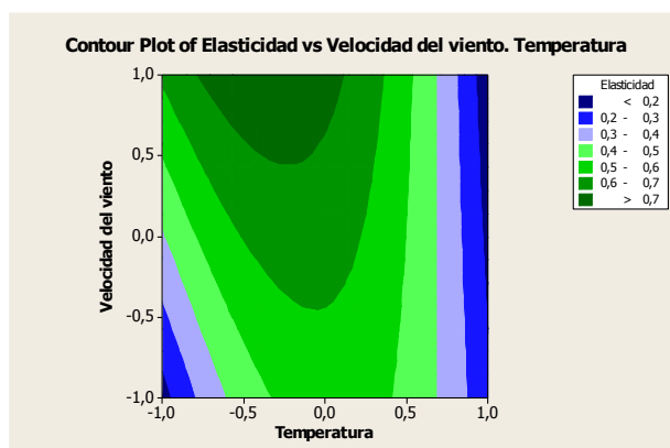
FIGURA 5.18 CONTORNO ELASTICIDAD
