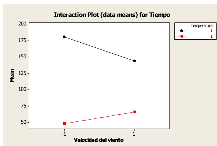
FIGURA 5.5 EFECTOS VARIABLES VS. TIEMPO DE SECADO
