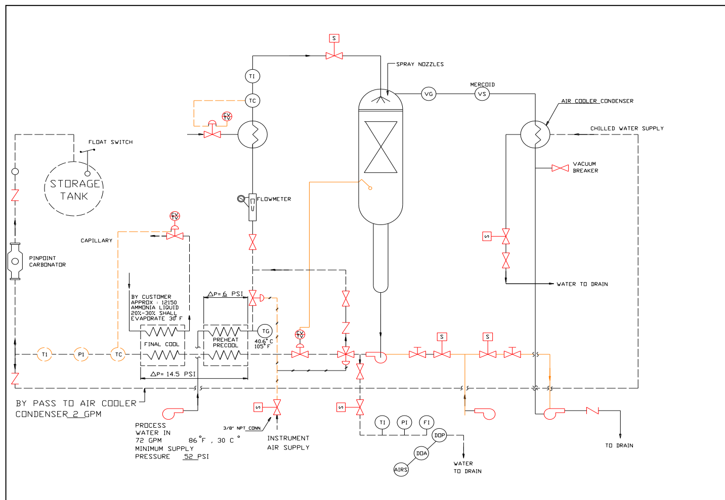
FIGURA 1.6 DIAGRAMA DE FUNCIONAMIENTO SEGÚN EL FABRICANTE
