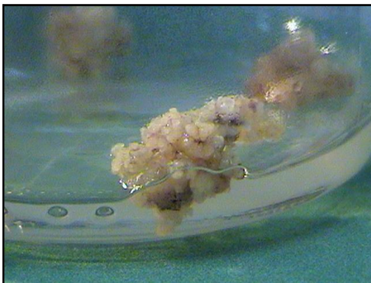
Figura 2.4. Inducción de callos en medio sólido enriquecido con 2,4-D. CINCAE, 2006.
