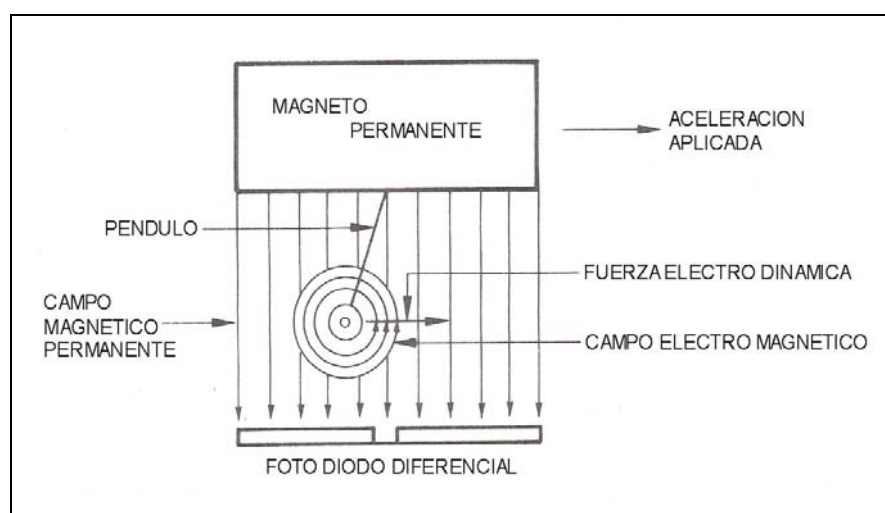
Figura 9.- Interacción del Campo Magnético, [9].
