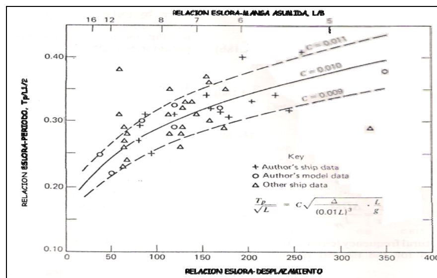
Figura 16.- Periodo de Cabeceo en función de la relación Eslora-Desplazamiento, [4].
