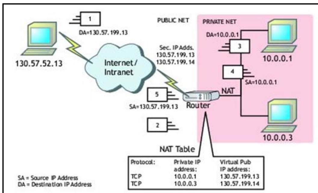
Figura 1.13 NAT Básico
