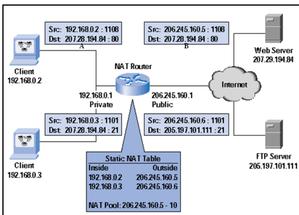
Figura 1.12 NAT Dinámico
