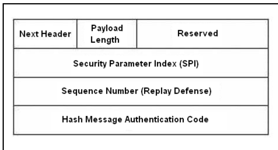
Figura 1.18 Cabecera AH
