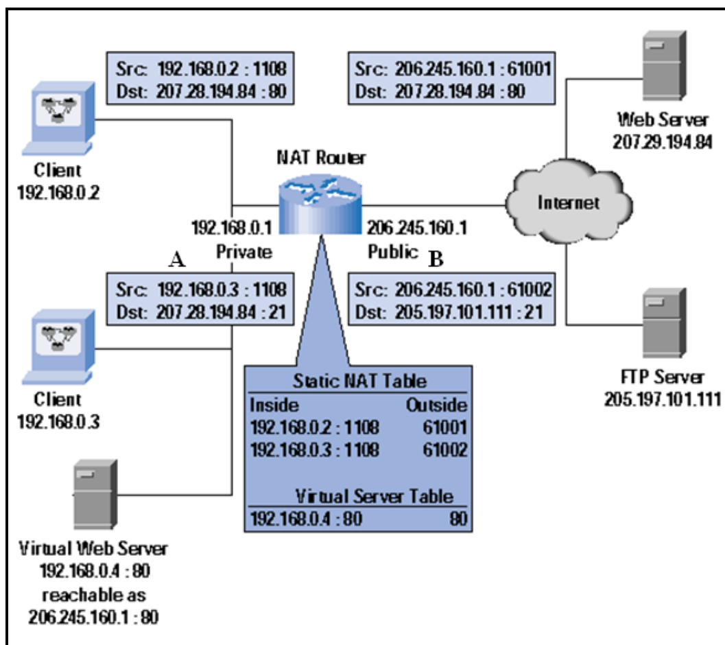
Figura 1.14 NAPT
