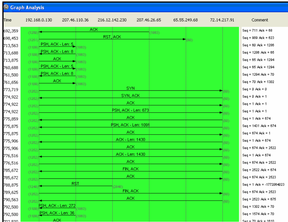
Figura 3.21.1 Análisis de Intrusión en Ethereal
