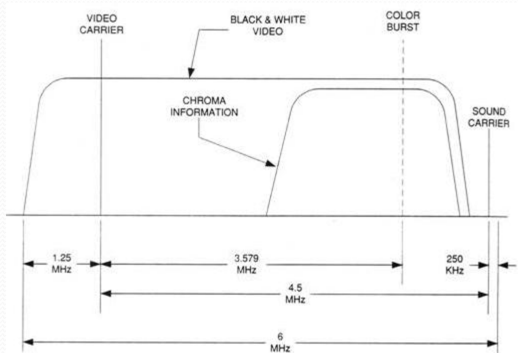
Ancho de banda de señal de video [3].
